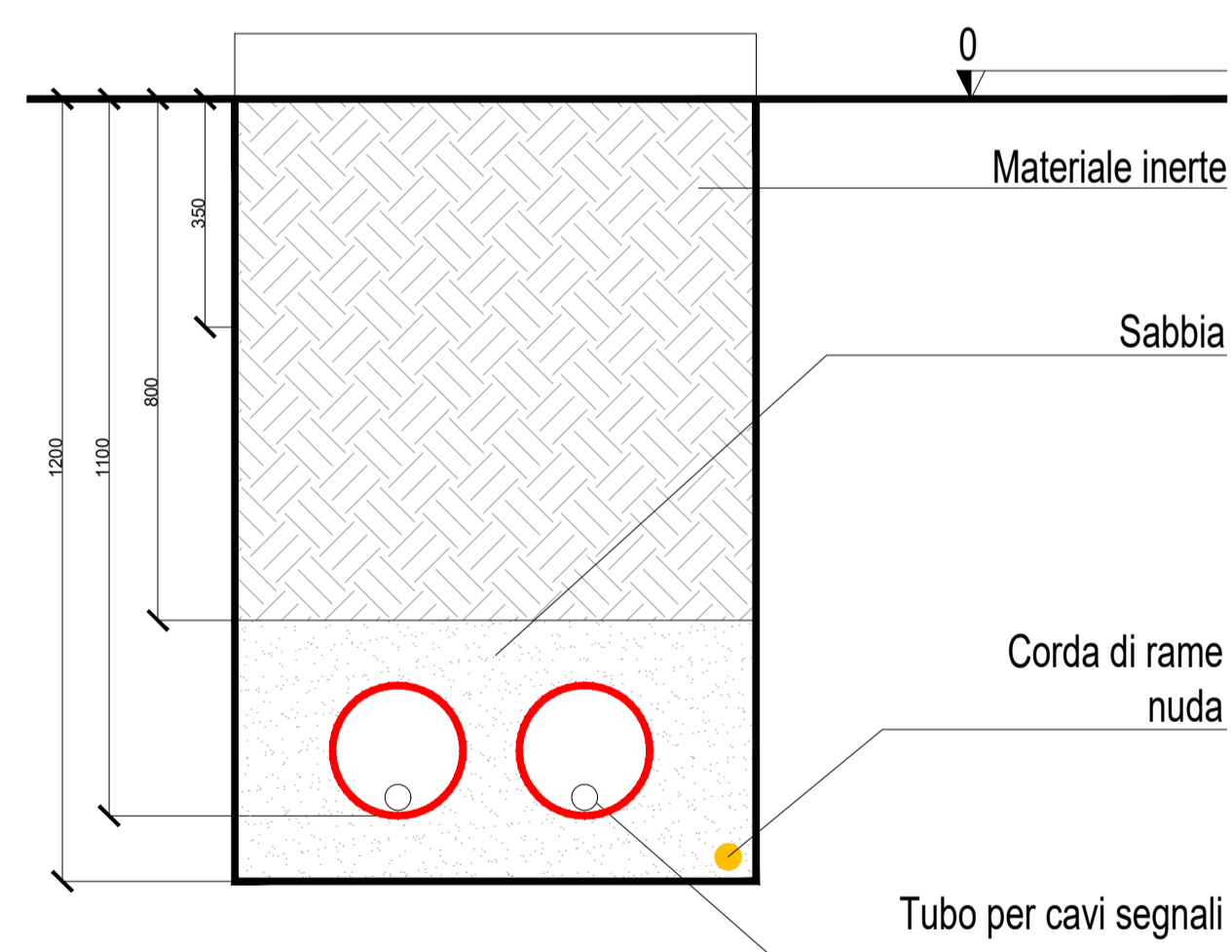
T04 - Tipologico scavo cavi segnale
