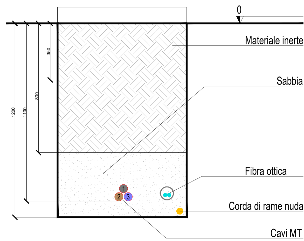
T01 - Tipologico scavo MT
