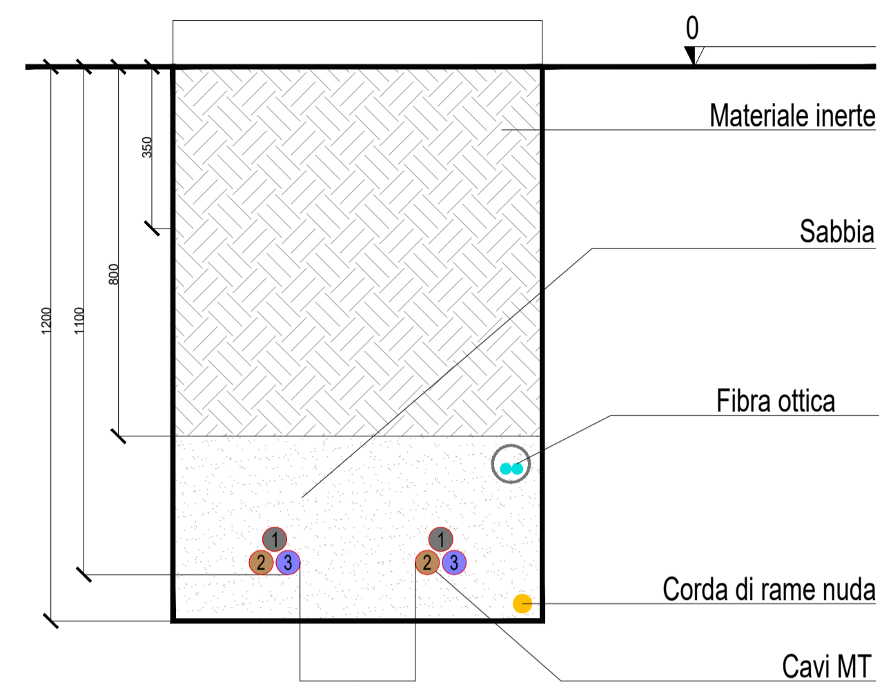
T02 - Tipologico scavo MT
