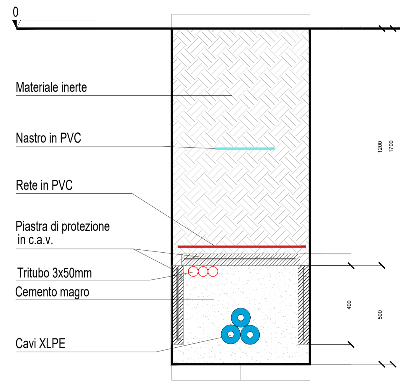
T05 - Tipologico cunicolo cavi segnale
