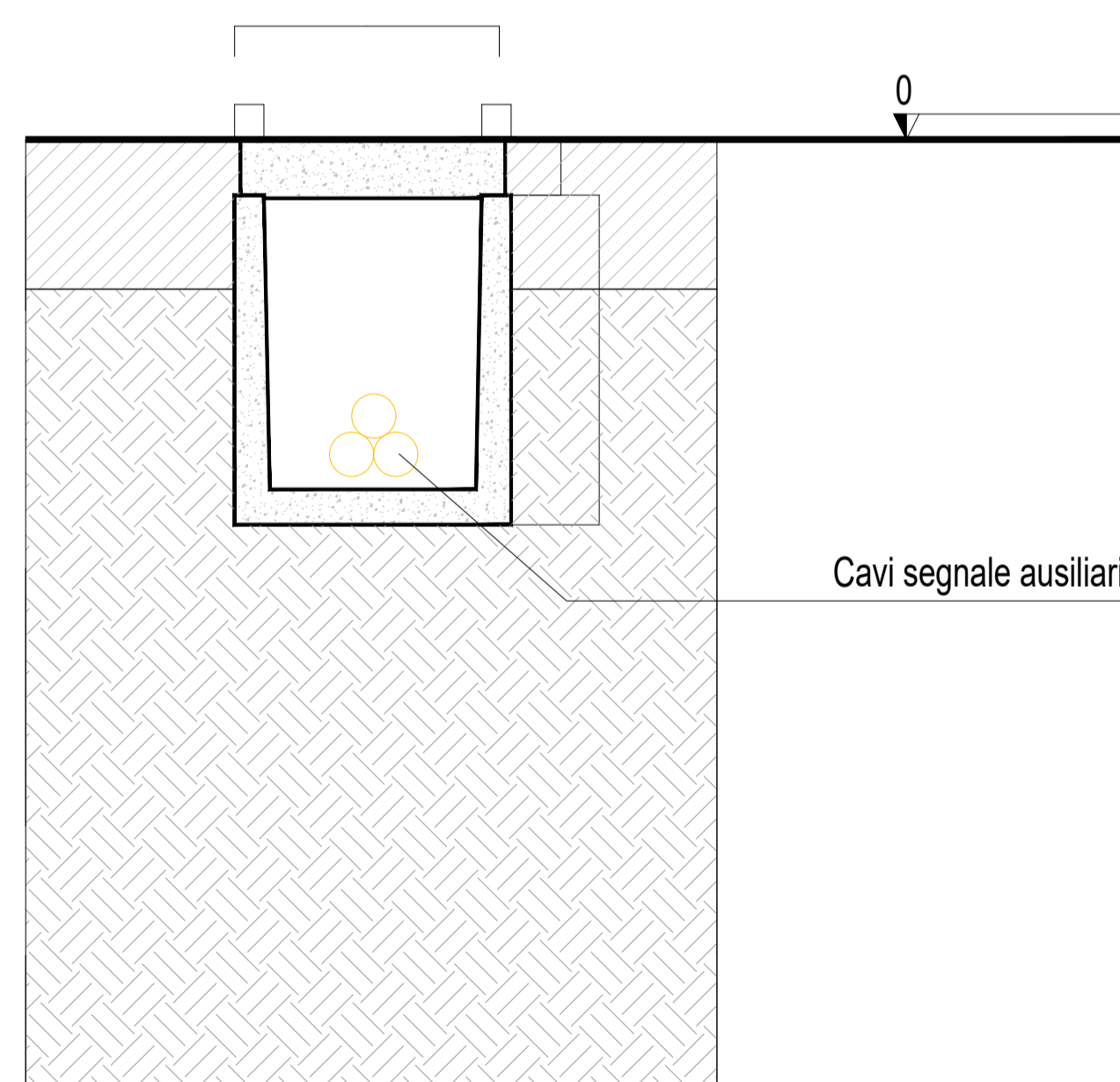
T05 - Tipologico cunicolo cavi segnale
