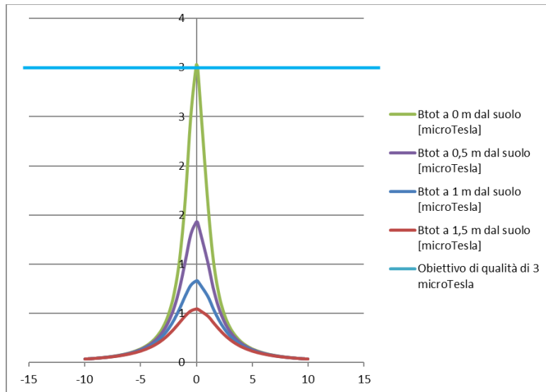
Figura 3: Andamento del campo magnetico generato dal cavidotto, composto da una terne da 95 mm 2
