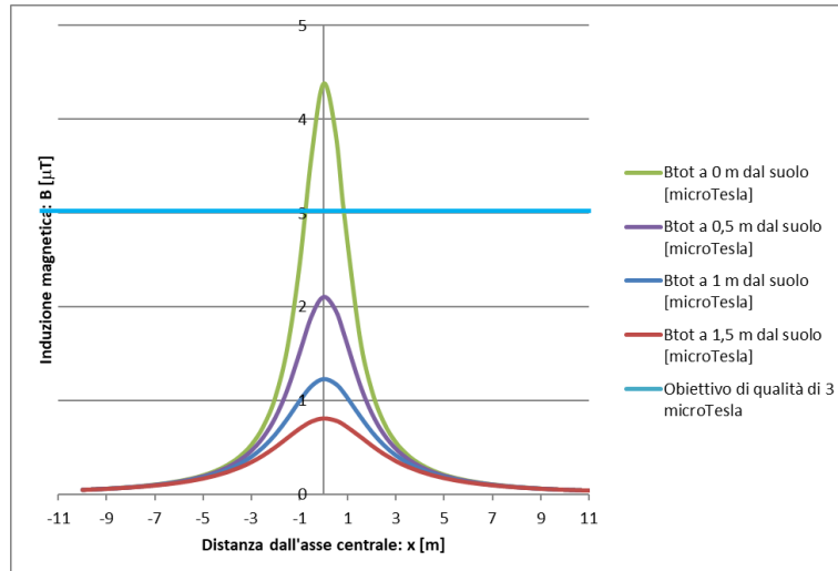
Andamento del campo magnetico generato composto da due terne una da 240 mm 2 e una da 630 mm 2
