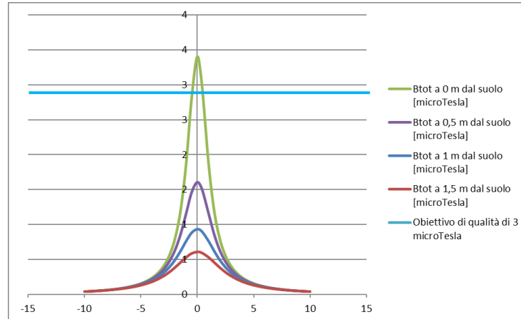
Andamento del campo magnetico generato dal cavidotto, composto da una terne da 240 mm 2
