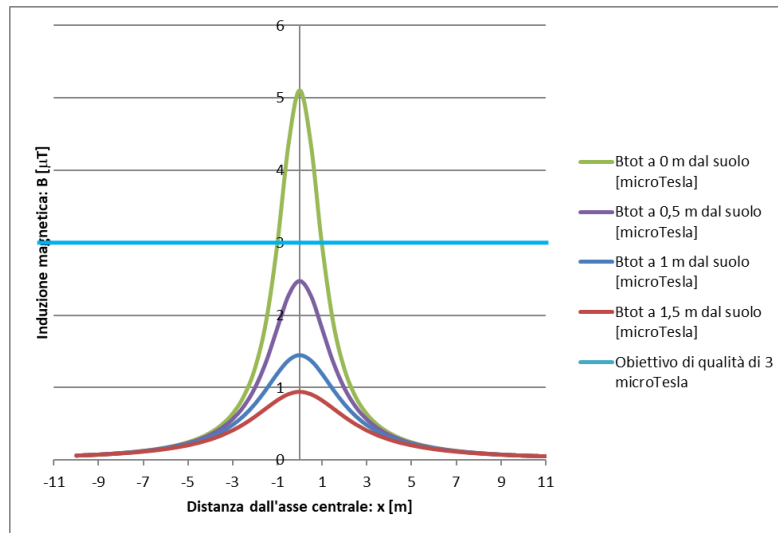
Andamento del campo magnetico generato dal cavidotto, composto da due terne una da 630 mm 2 e una da 400 mm 2
