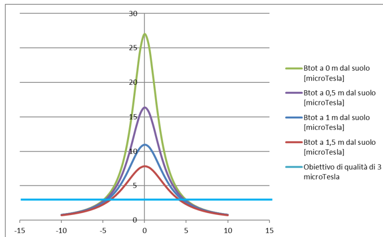
Andamento del campo magnetico generato dal cavidotto, composto da una terne da 1.600 mm 2
