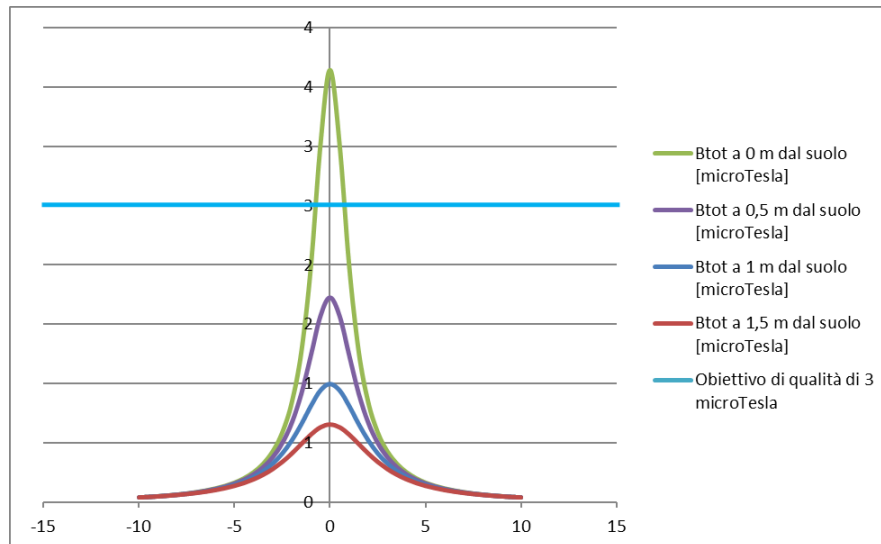
Andamento del campo magnetico generato dal cavidotto, composto da una terne da 630 mm 2
