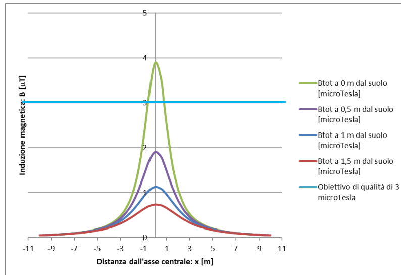
Andamento del campo magnetico generato dal cavidotto, composto da due terne una da 240 mm 2 e una da 400 mm 2
