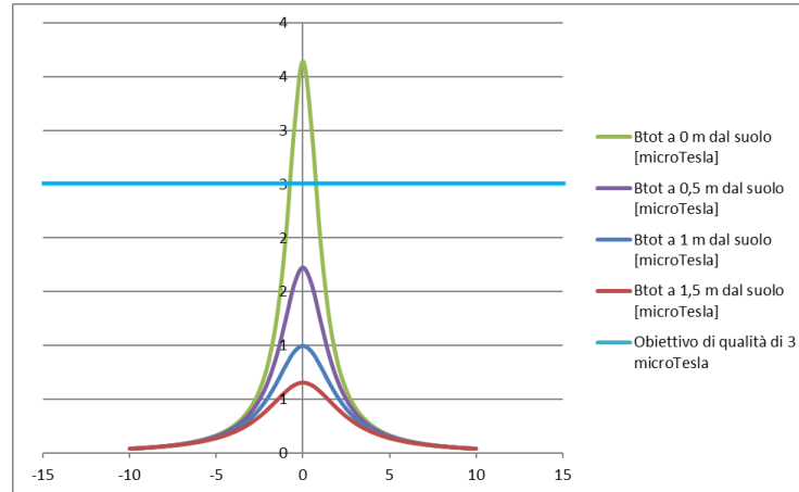
Andamento del campo magnetico generato dal caviodotto, composto da una terne da 400 mm 2
