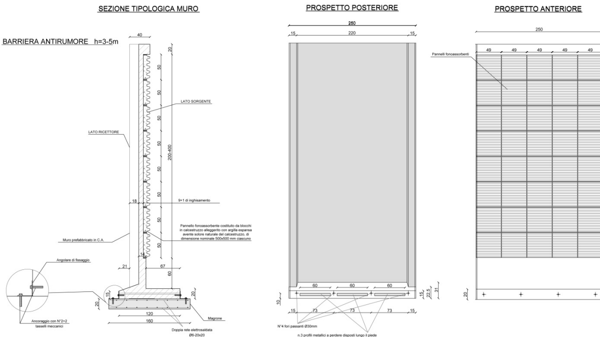
Figura 4 Tipologico barriere
