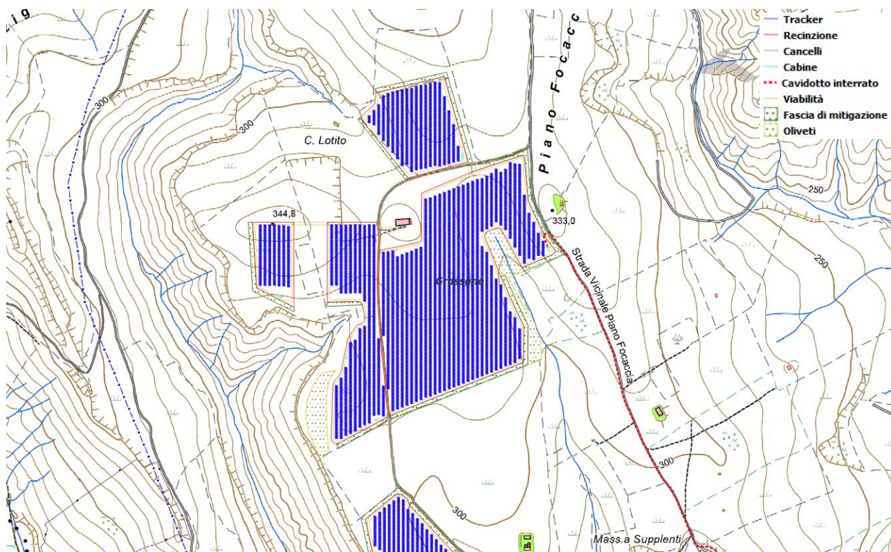
Figura 1.3a. -Individuazione dell'impianto agro-voltaico su CTR - dettaglio
