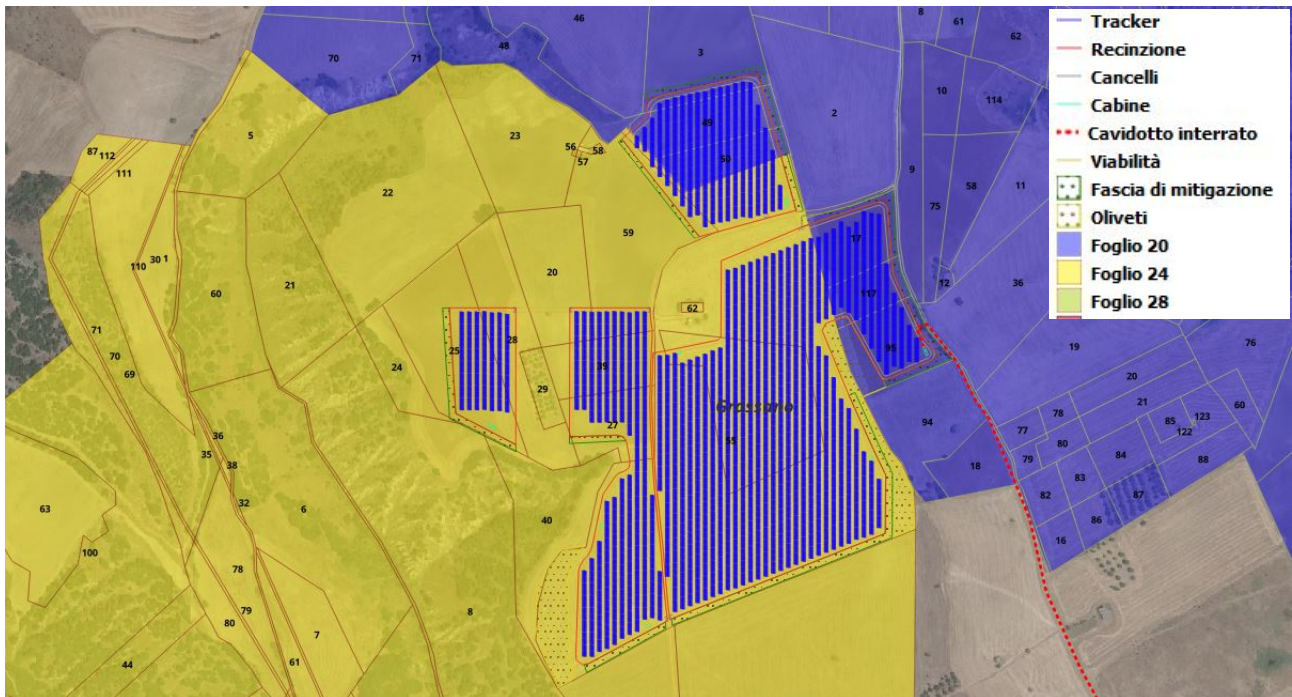
Figura 1.4a. – Inquadramento dell'area di progetto su catastale - dettaglio
