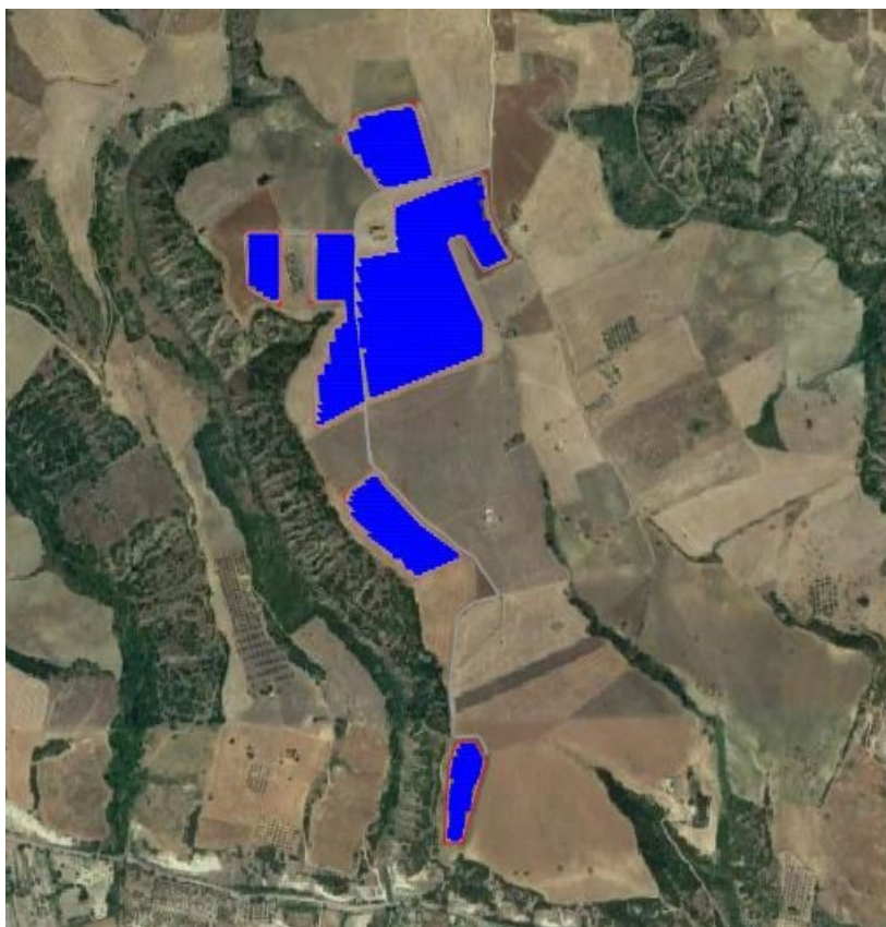
Figura 4.5. – Layout del sistema fotovoltaico con supporti fissi.
