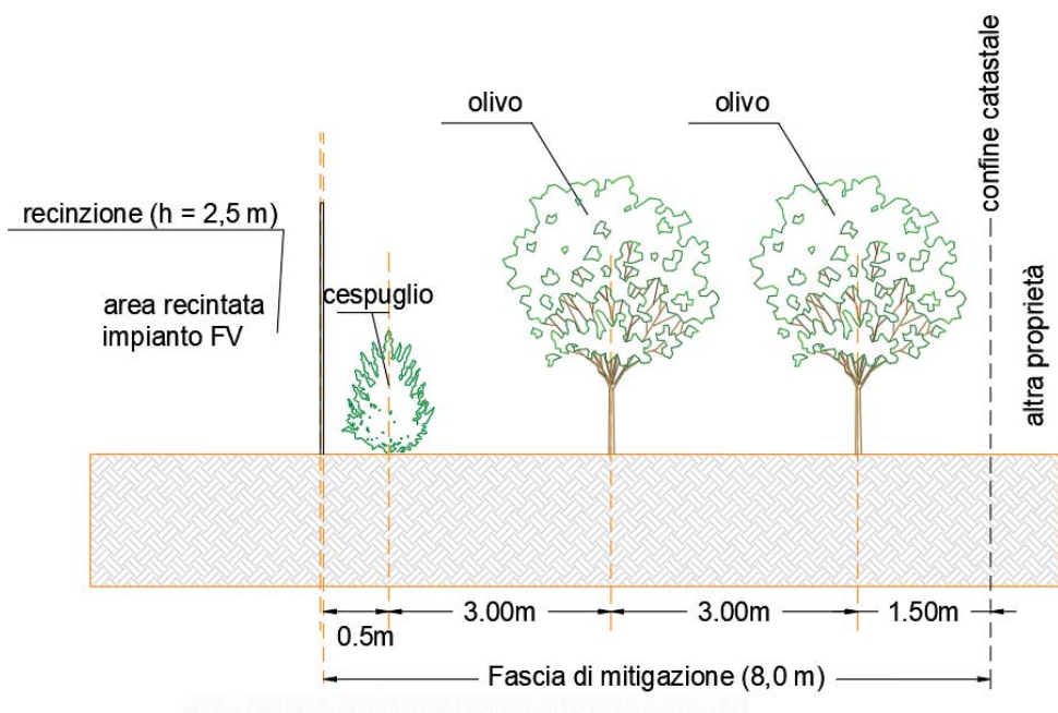
Figura 2.15. – Stralcio di sezione dell'area perimetrale dell'impianto _siepe e doppio filare di olivo
