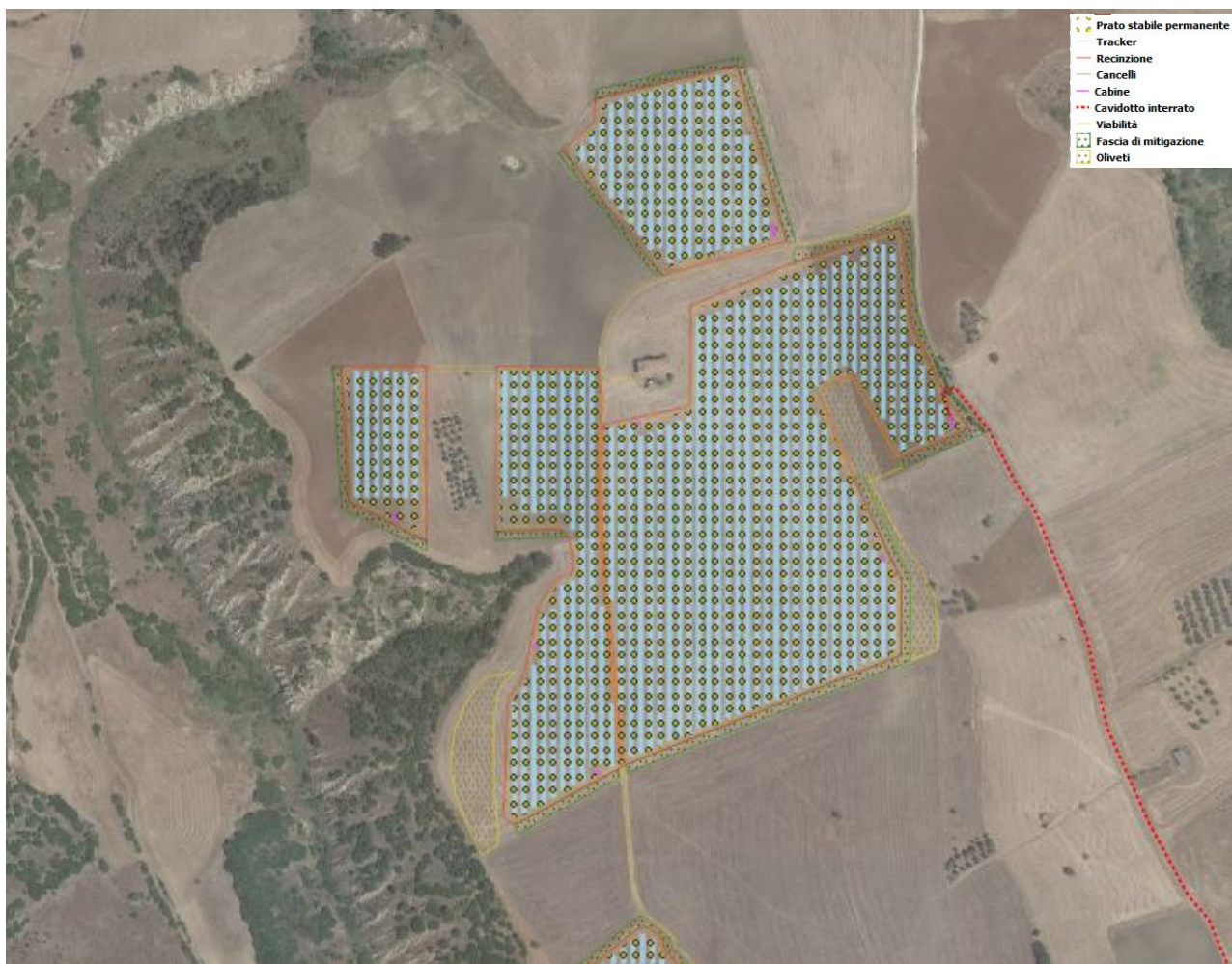
Figura 2.10 – Area di interesse dell’Impianto Agrovoltaiico -dettaglio
