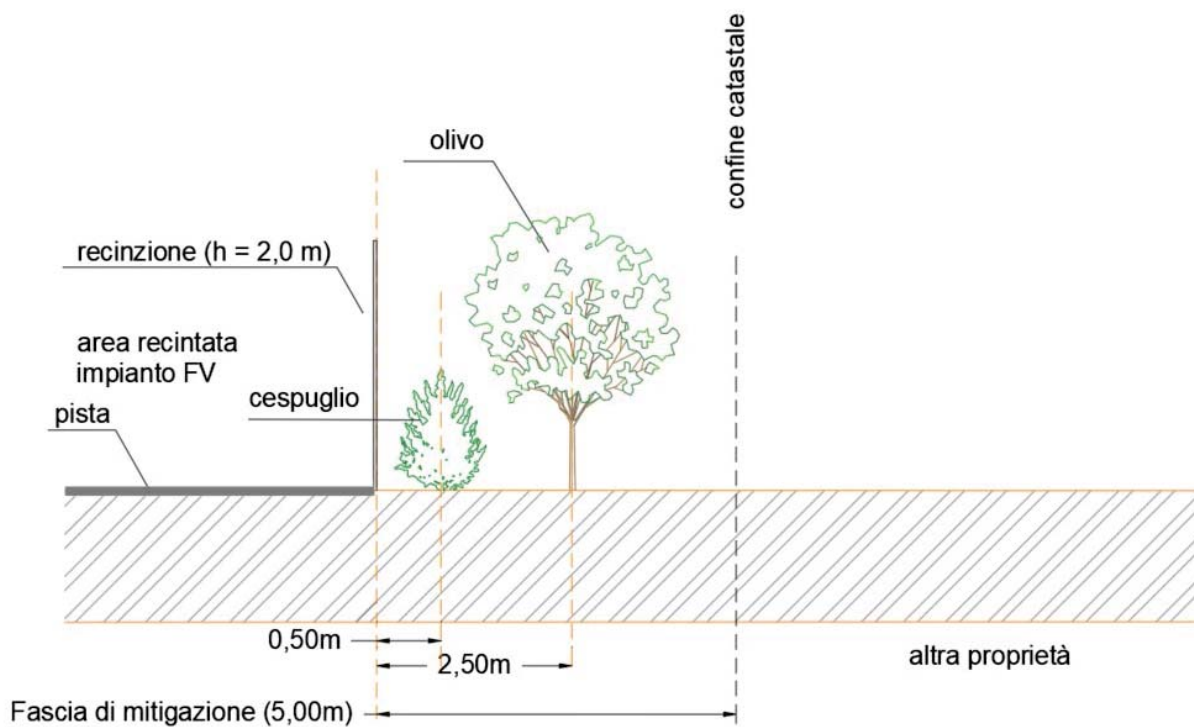
Figura 2.12. – Stralcio di sezione dell'area perimetrale dell'impianto- siepe e unico filare di olivo
