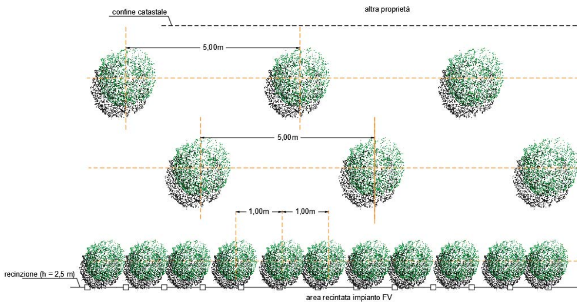
Figura 2.14 – Siepe polispecifica (planimetria di progetto) _siepe e doppio filare di olivo
