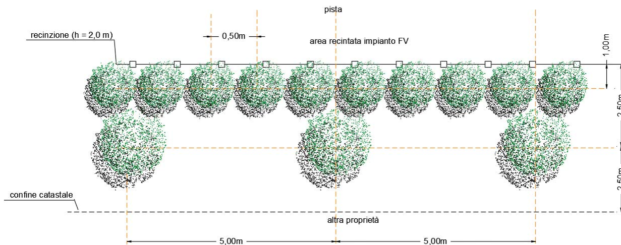
Figura 2.11 – Siepe polispecifica (planimetria di progetto) - siepe e unico filare di olivo
