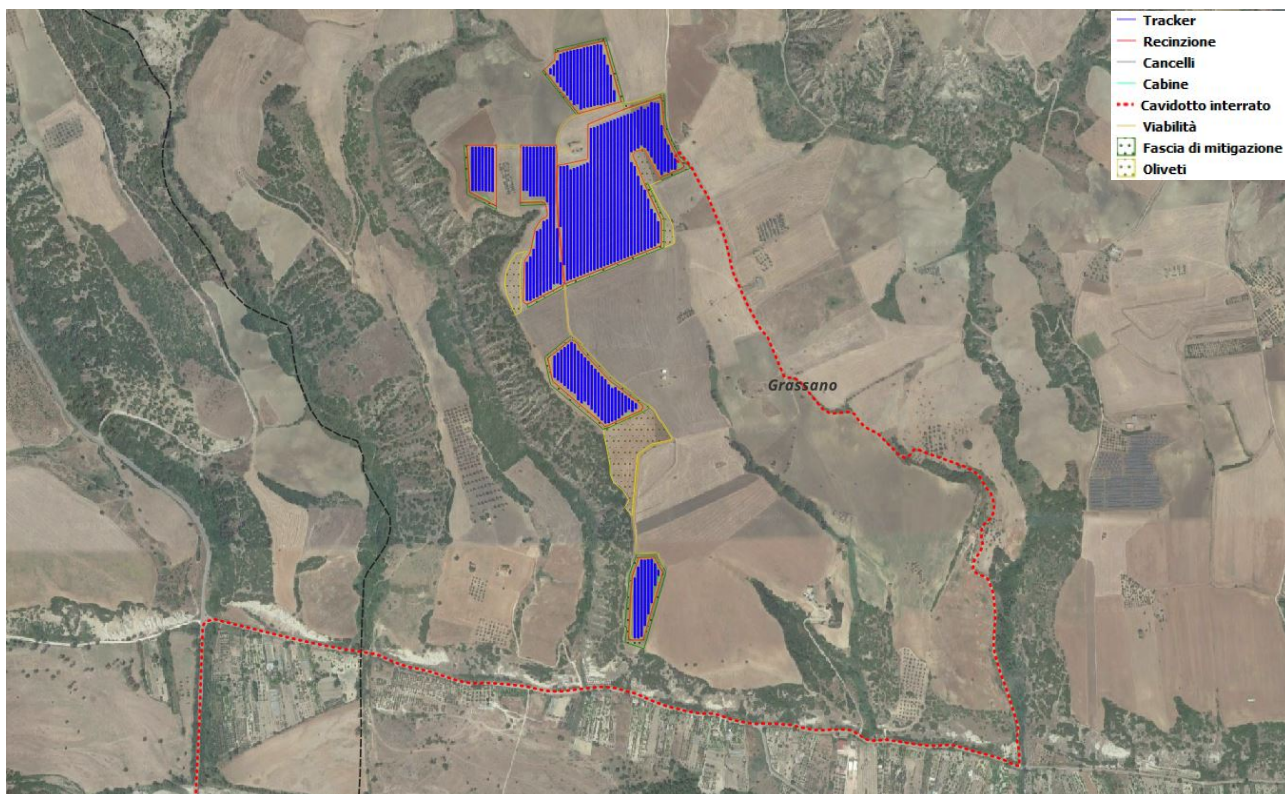
Figura 1.2a – Area di progetto impianto agrivoltaico su ortofoto - dettaglio.
