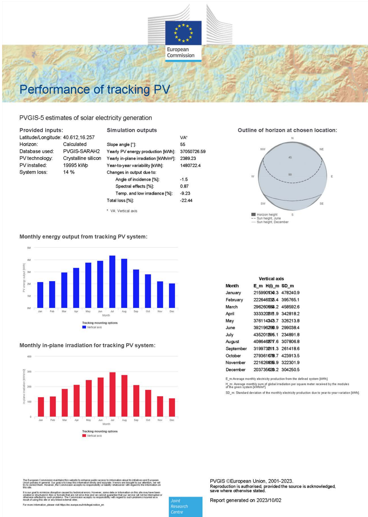
Figura 4.9. – Simulazione di producibilità annua del sistema fotovoltaico Agrivoltaico con tracker.
