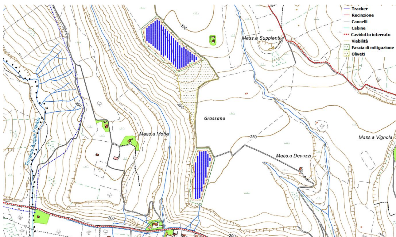
Figura 1.3b. –Individuazione dell’impianto agro-voltaico su CTR - dettaglio
