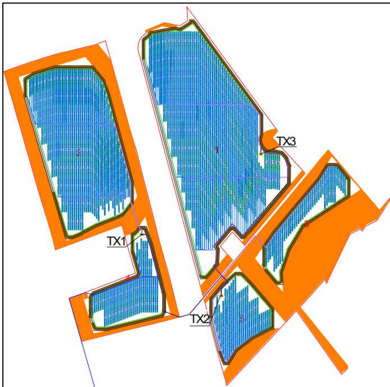
Lay-out impianto con indicazione dei trasformatori
