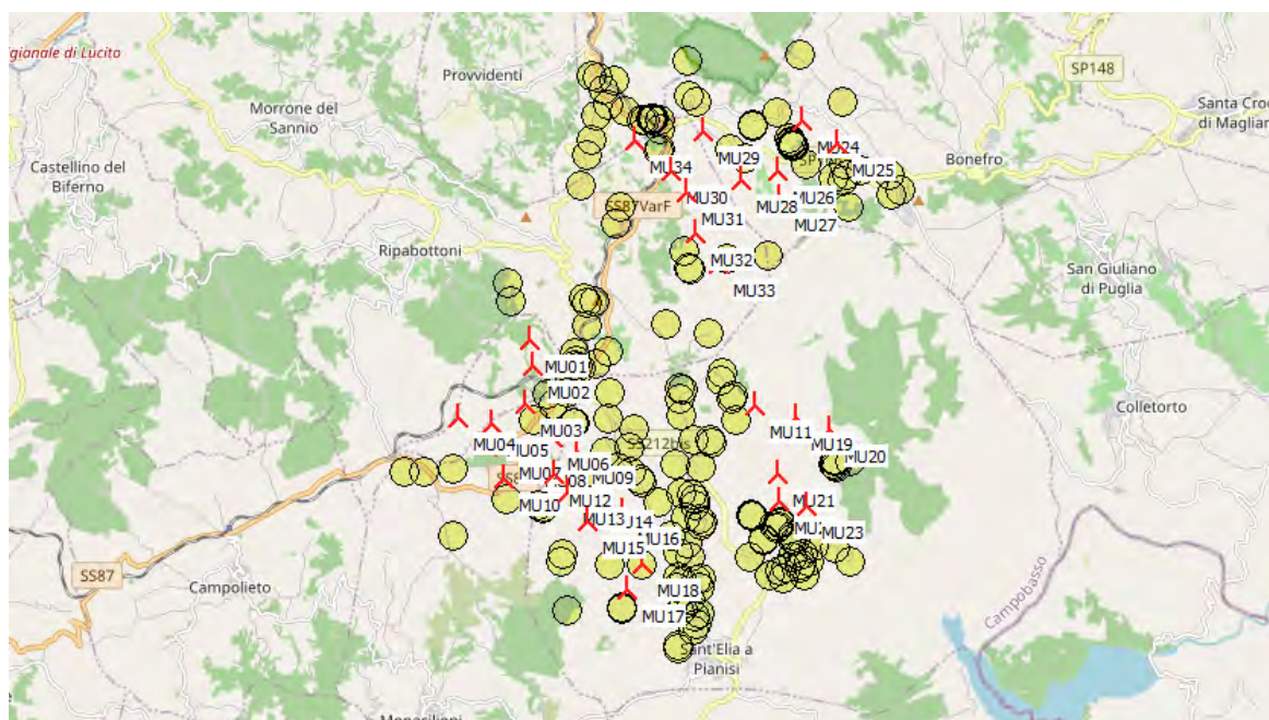
Figura 6.1: Disposizione planimetrica degli aerogeneratori di progetto e dei recettori
