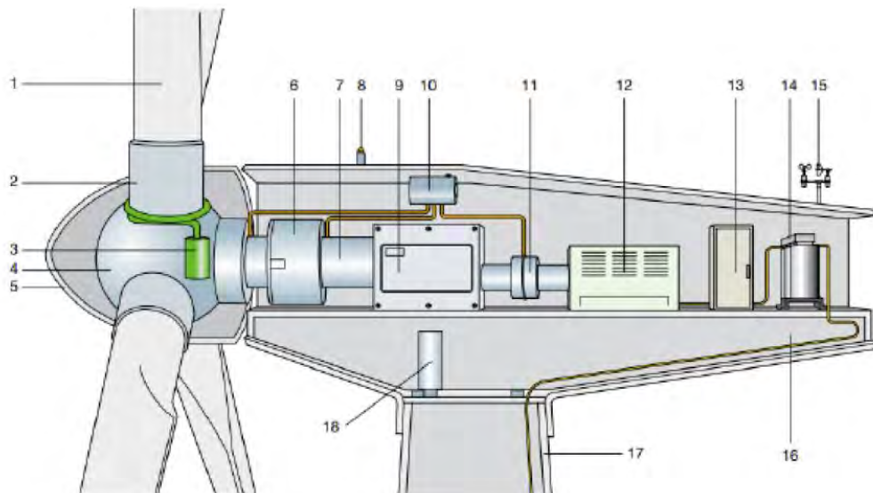
Figura 4.1: Schema navicella aerogeneratore
