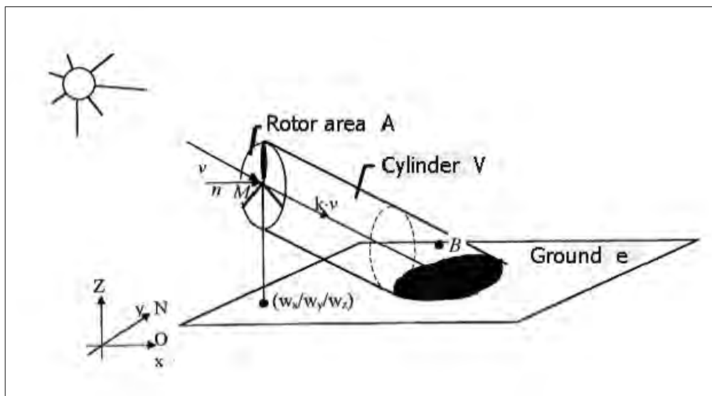
Figura 6.2: Schema di calcolo del modulo Shadow
