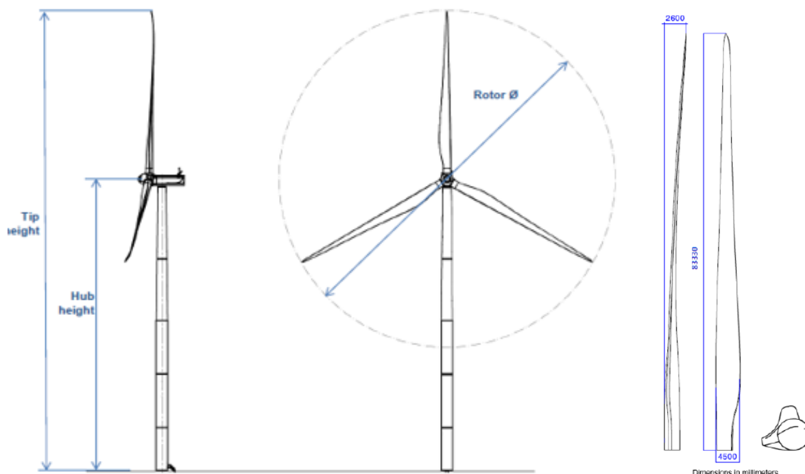
Figura 2.1: Struttura aerogeneratore
