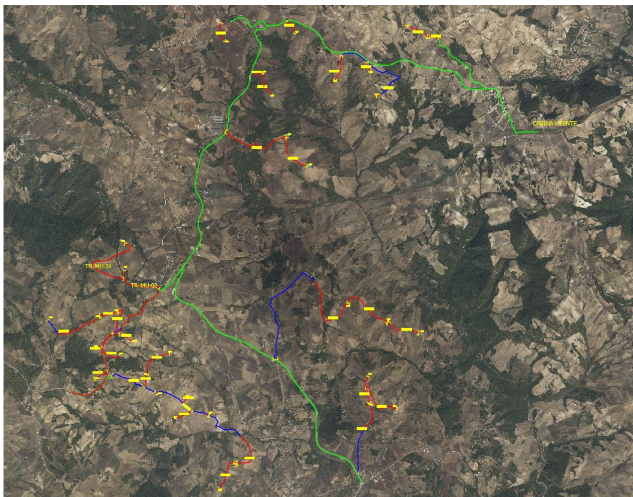
Figura 2.9: viabilità interna al sito (rosso=nuove piste; verde=strade asfaltate esistenti; blu=strade esistenti da adeguare)
