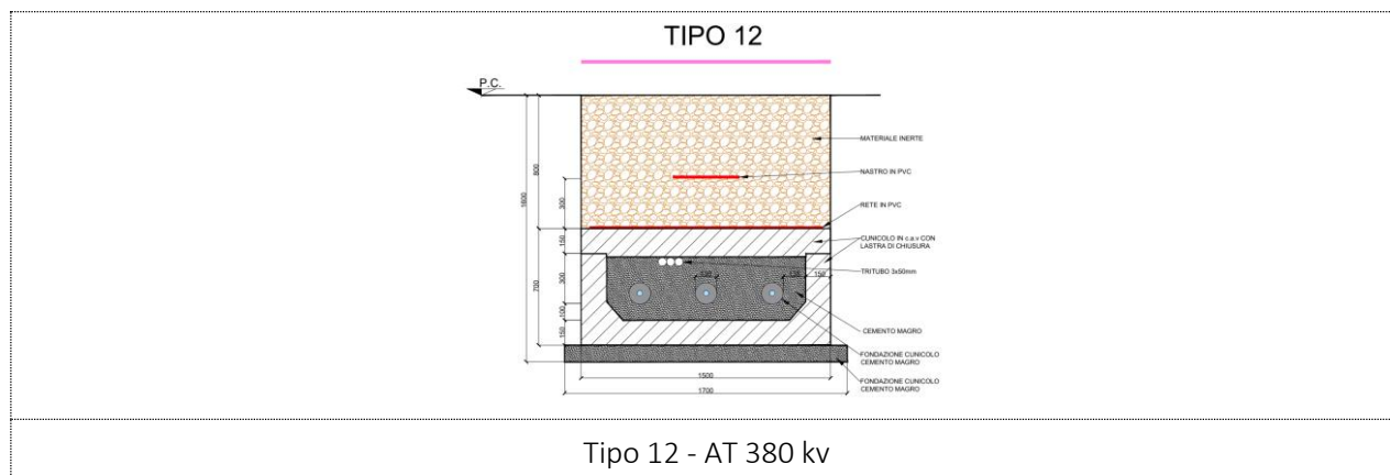
Figura 2.11 – Sezioni tipo posa cavidotti
