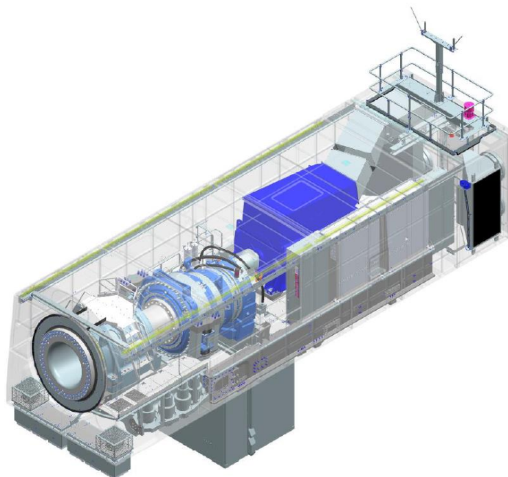
Figura 2.3 - Struttura navicella
