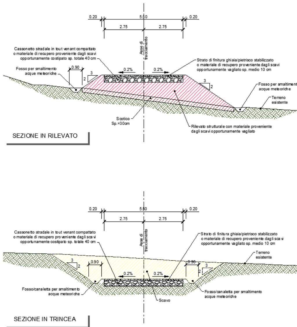
Figura 2.10 – Sezione tipo piste di accesso
