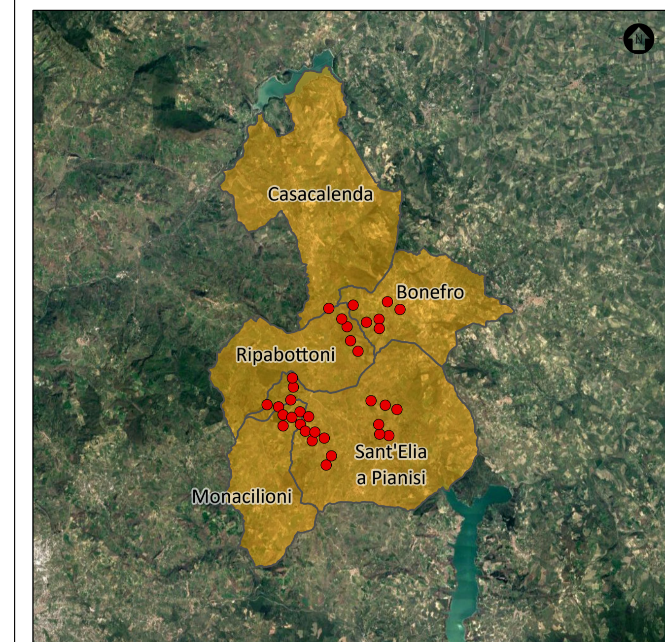
INQUADRAMENTO TERRITORIALE SCALA 1:200.000 1 cm = 2 km 0 4 8 16 km LEGENDA ● Aerogeneratore di progetto ■ Comune di riferimento
