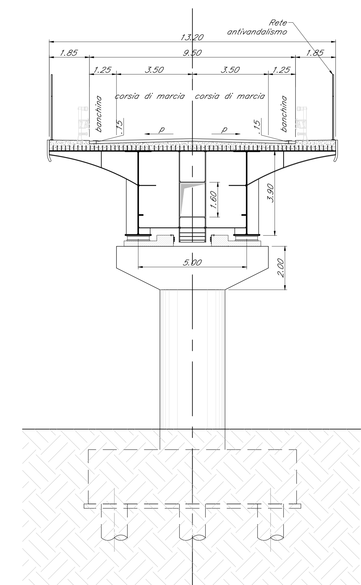
SEZIONE APPOGGI PILA 9
