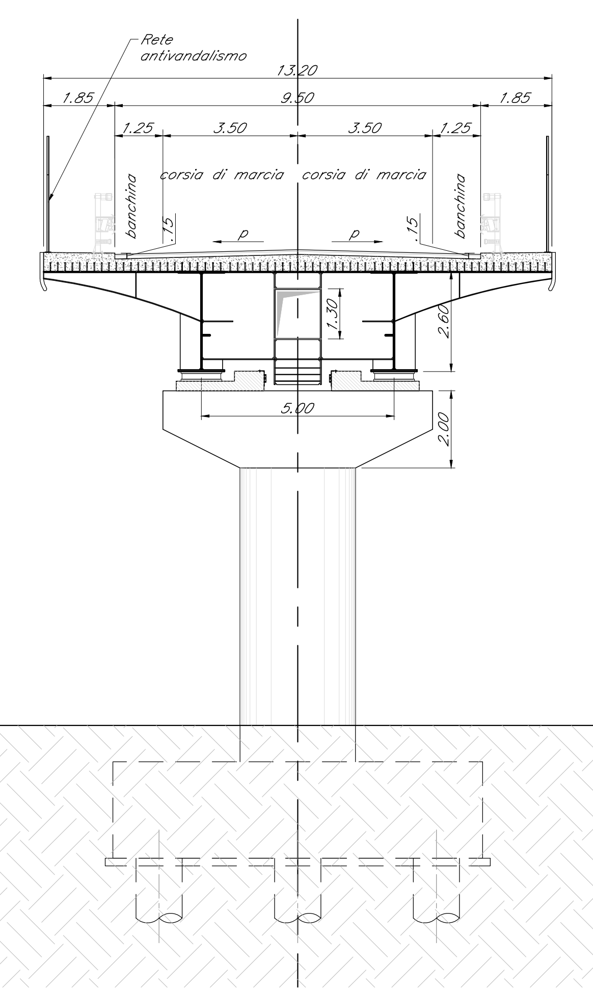
SEZIONE APOGGI PILA 12
