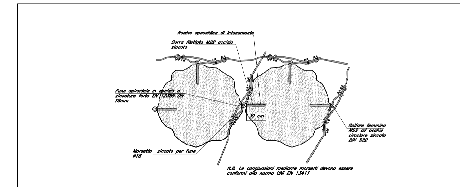
Particolare legatura massi scala 1:25
