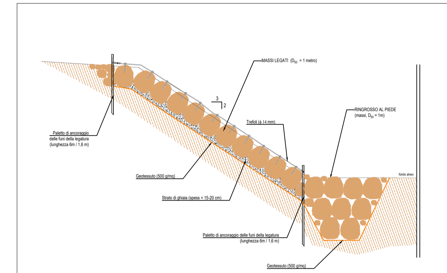
Tipologico sistemazione spondale scala 1:100
