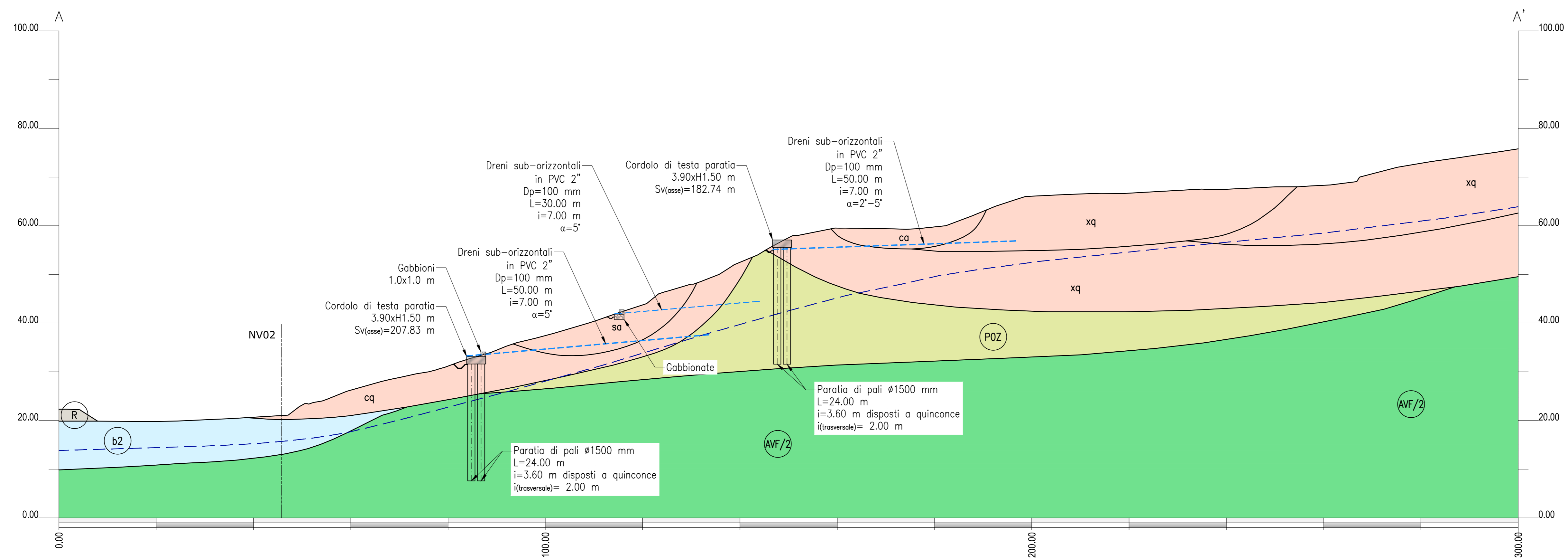
SEZIONE A-A' Scala 1:500
