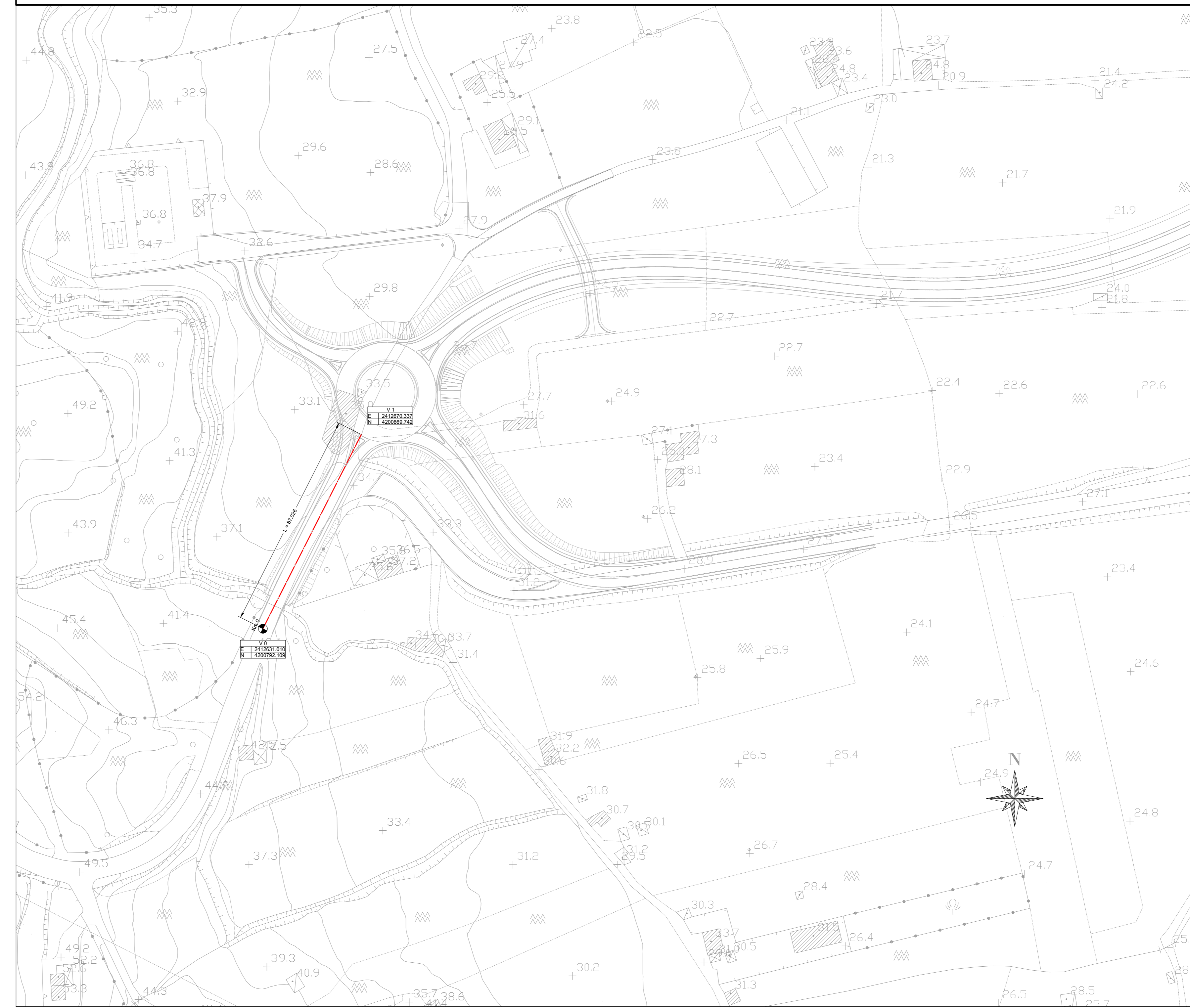
PLANIMETRIA DI TRACCIAMENTO ROTATORIA OVEST - Scala 1:1000
