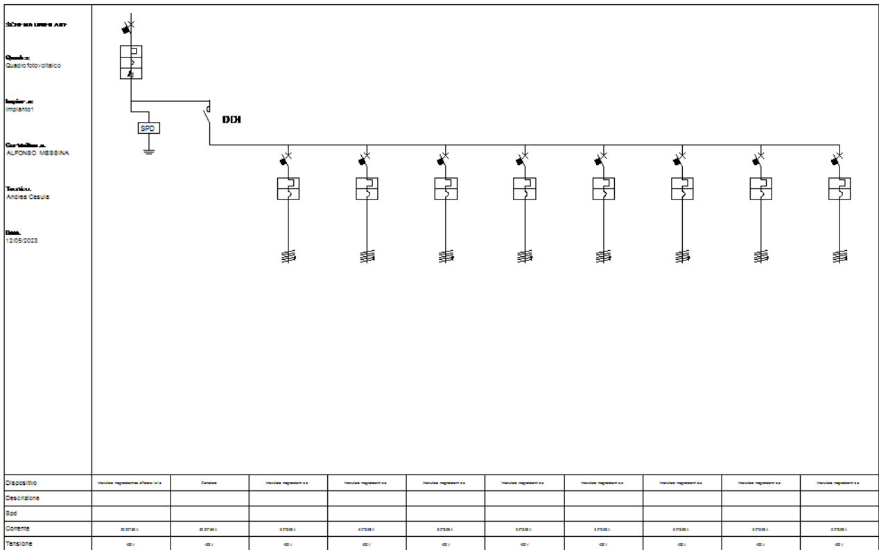
Fig. 5: Schema unifilare quadro "Quadro fotovoltaico"
