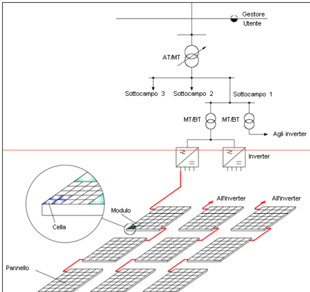
Figura 1: Schema collegamento centrale fotovoltaica
