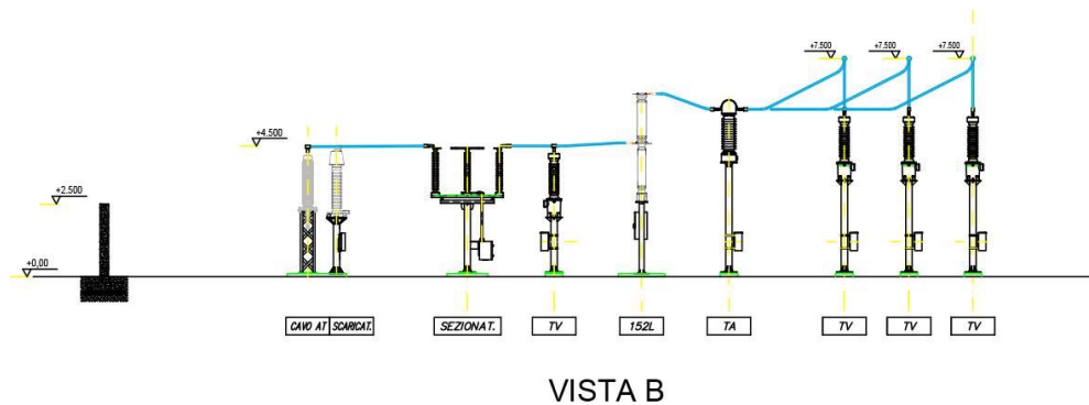
Figura 3: Sezioni SS Terna Seu tre progetti SF
