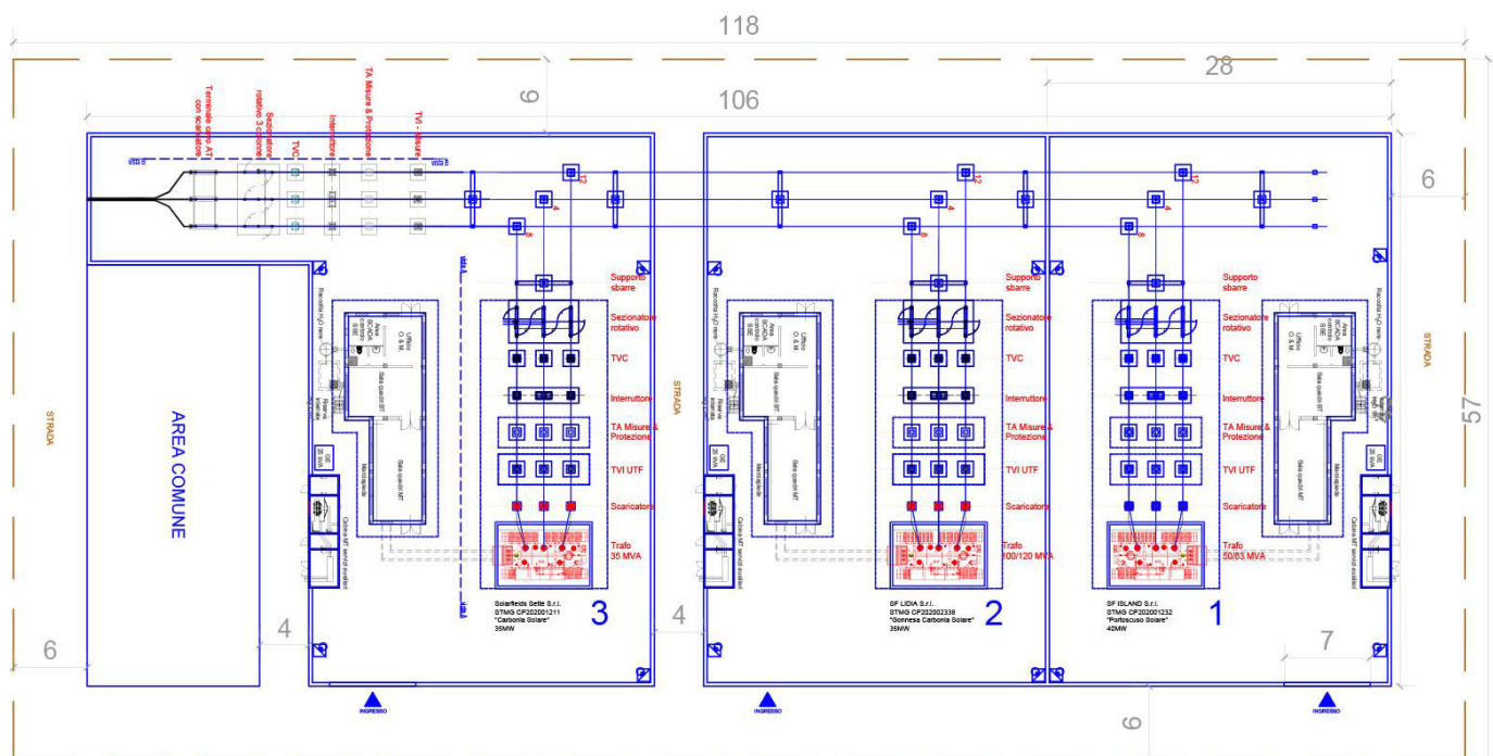
Figura 2 : Planimetria SS Terna Seu tre progetti SF
