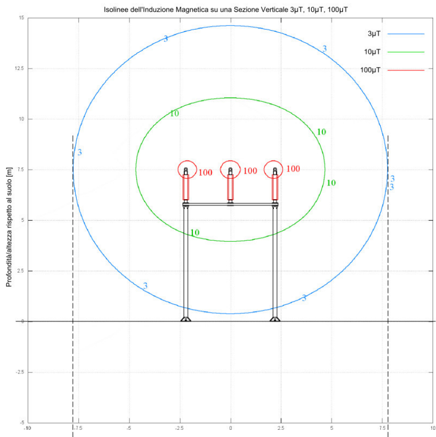
Figura 7 - Sbarre AT in aria - Isolinee induzione magnetica 3, 10 e 100 \mu T
