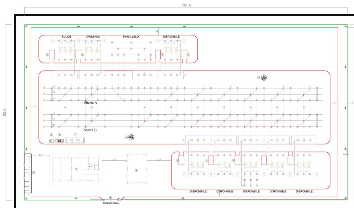
Figura 9 - Sbarre AT in aria – Planimetria elettromeccanica nel quali si registra l' induzione magnetica 3, 10 e 100 \mu\text{T}
