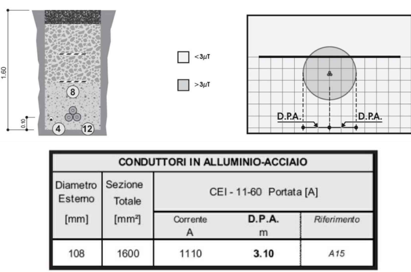
D.P.A - SEZIONI CAVI COLLEGAMENTO QUADRI CAMPO-TRAFI STATION
