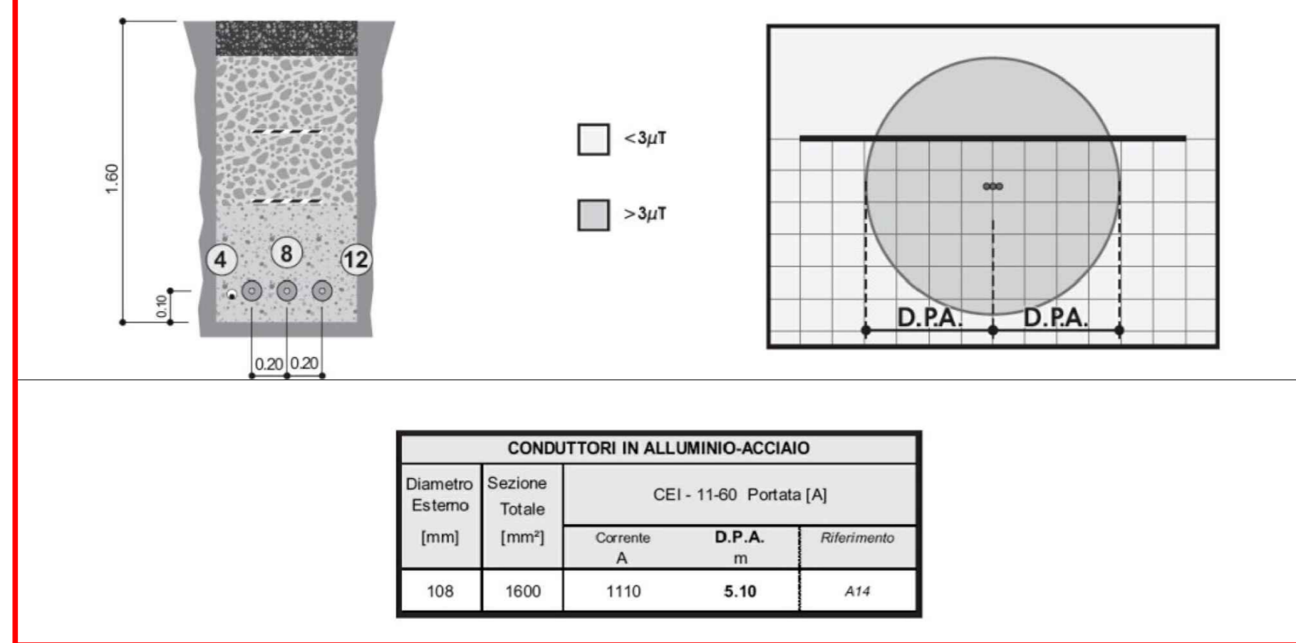
D.P.A - SEZIONI CAVI COLLEGAMENTO CABINA CONCENTRAZIONE-RTN
