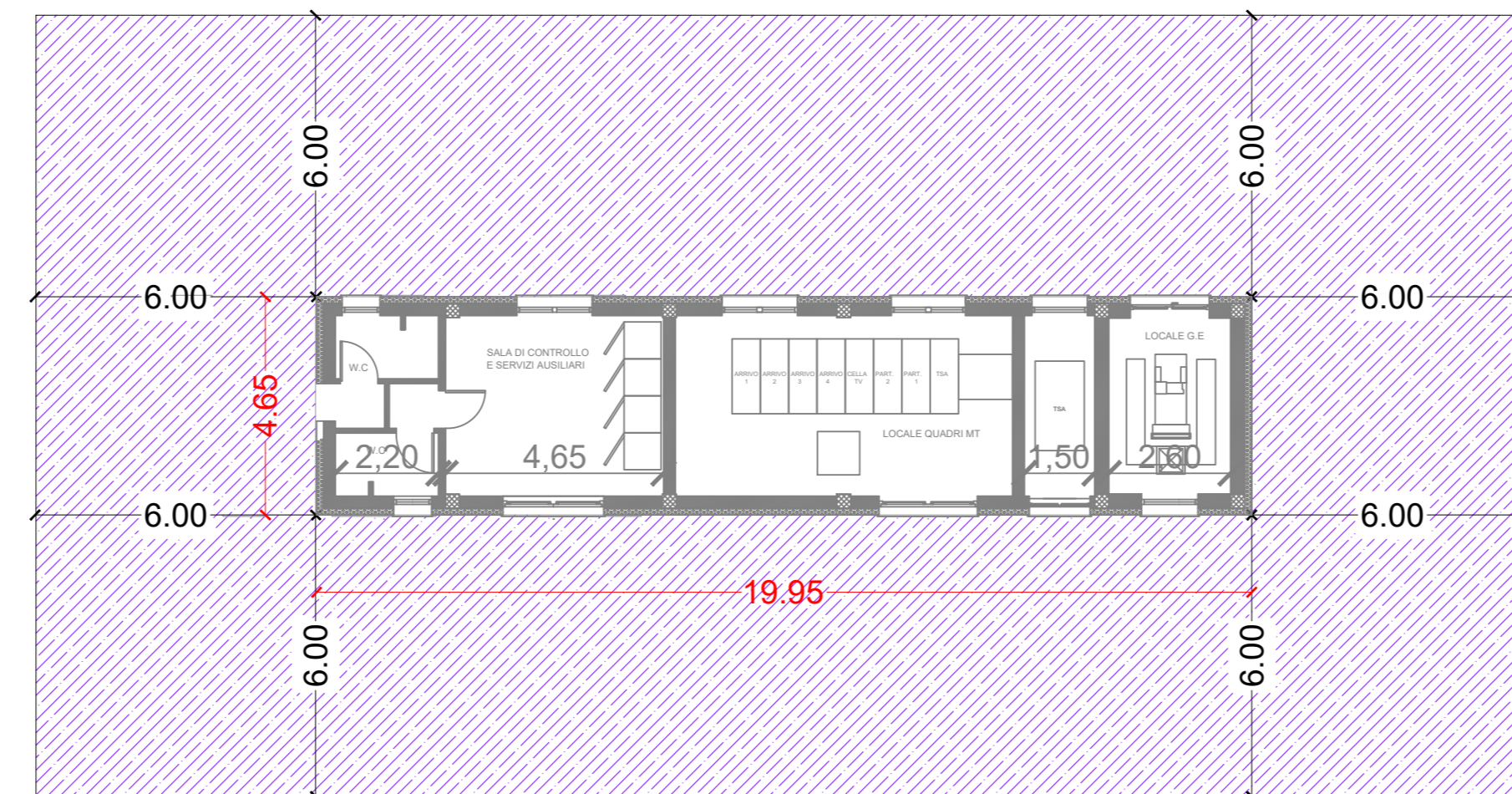
D.P.A - CABINA DI CONCENTRAZIONE SCALA 1:100
