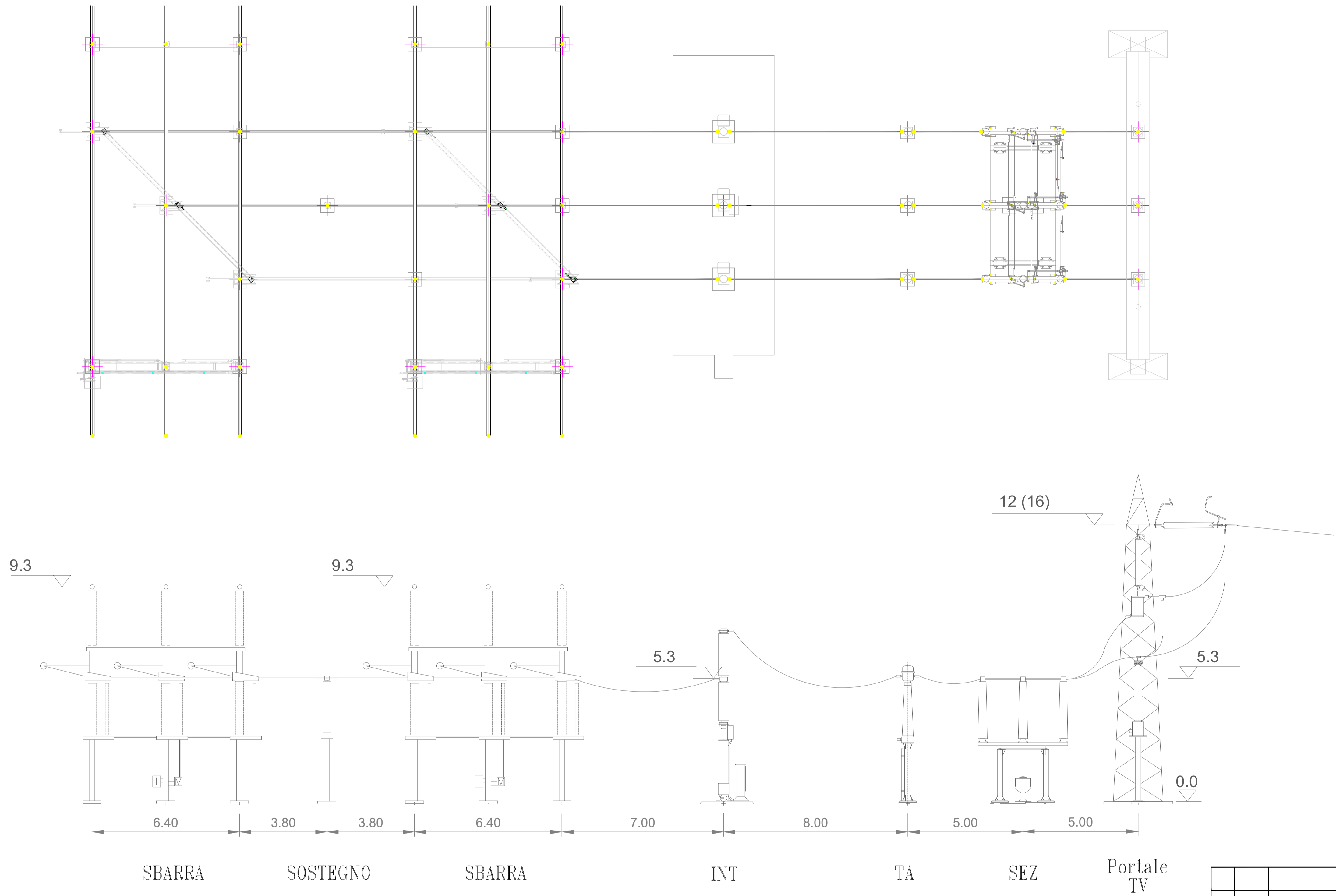
Sezione stallo linea aerea 220kV
