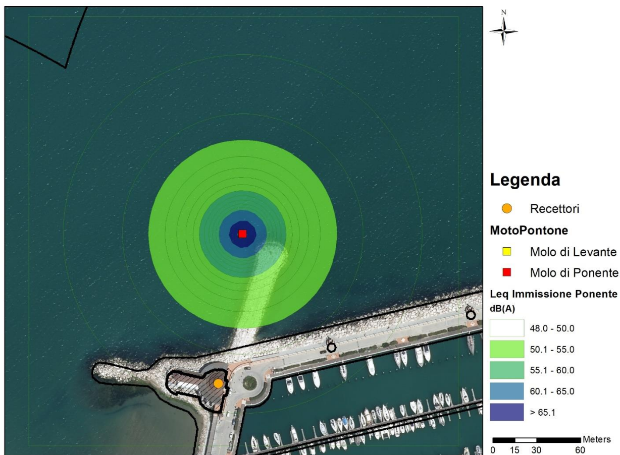
Figura 8 – Leq Immissione Diurna in dBA – Rumore ambientale in fase di cantiere (Molo Ponente)
