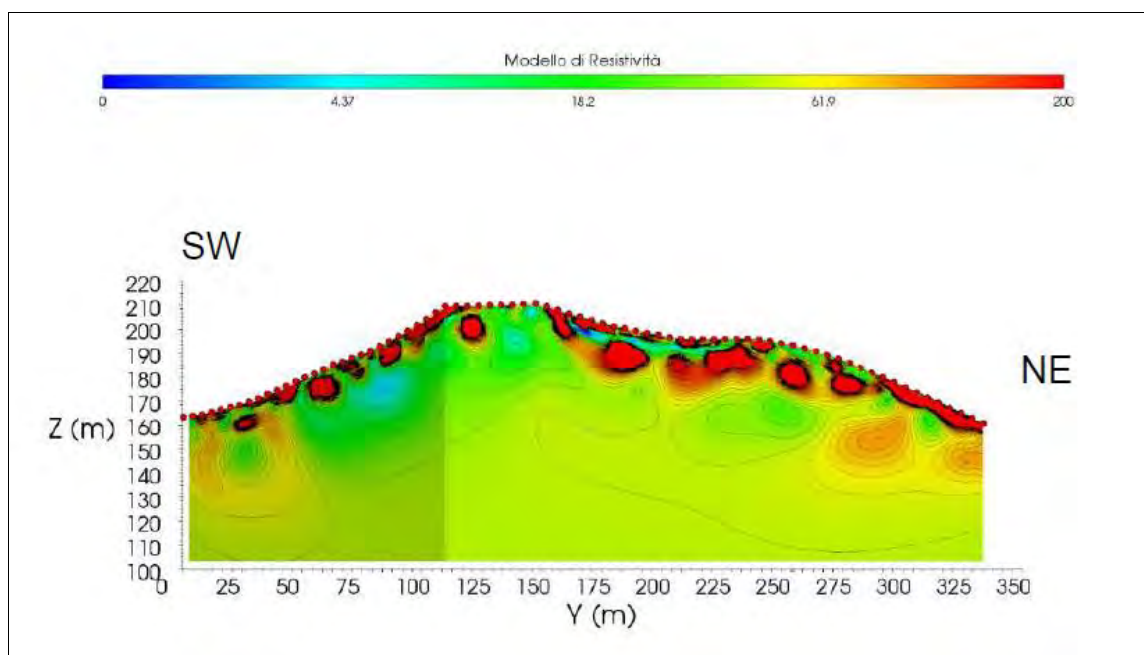
Figura 7-B: Tomografia elettrica ERT20_SM_L
