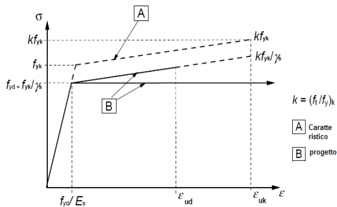
Legame elastico perfettamente plastico o inrudente o duttilità limitata per l'acciaio
