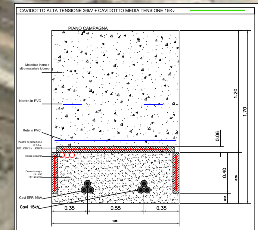
SEZIONE "B-B"
