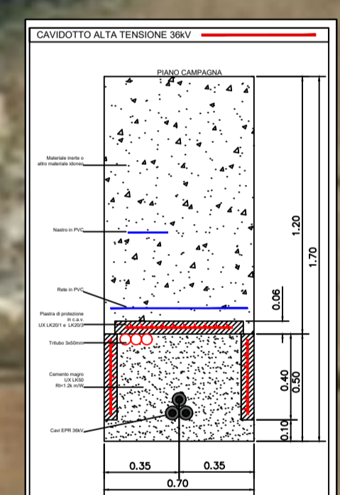
SEZIONE "A-A"
