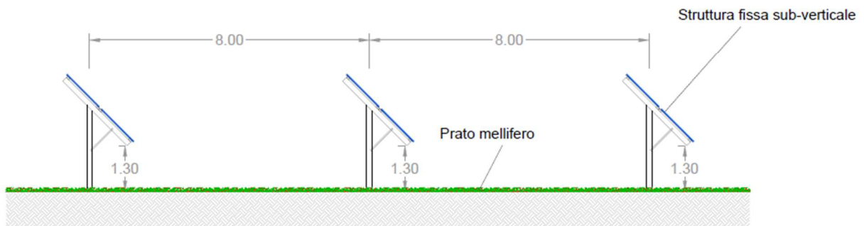
Sezione esemplificativa agrivoltaico Plot 2
