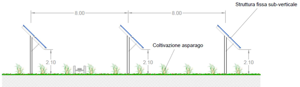
Sezione esemplificativa agrivoltaico Plot 1
