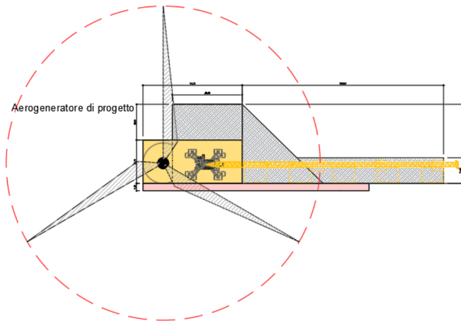
Figura 2. Dettaglio piazzola di montaggio
