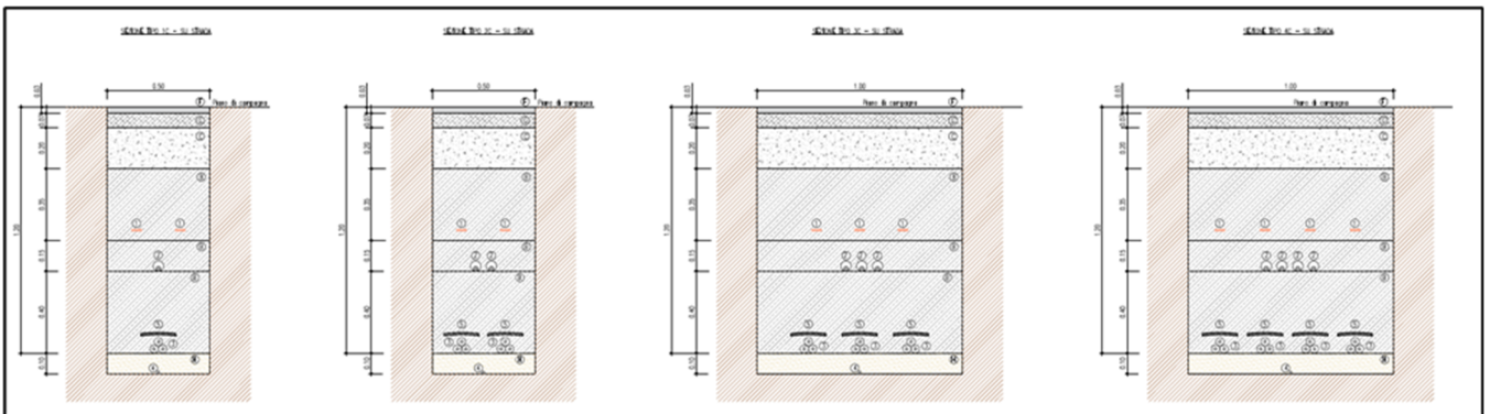
Figura 6: sezioni tipologiche cavidotto su strada
