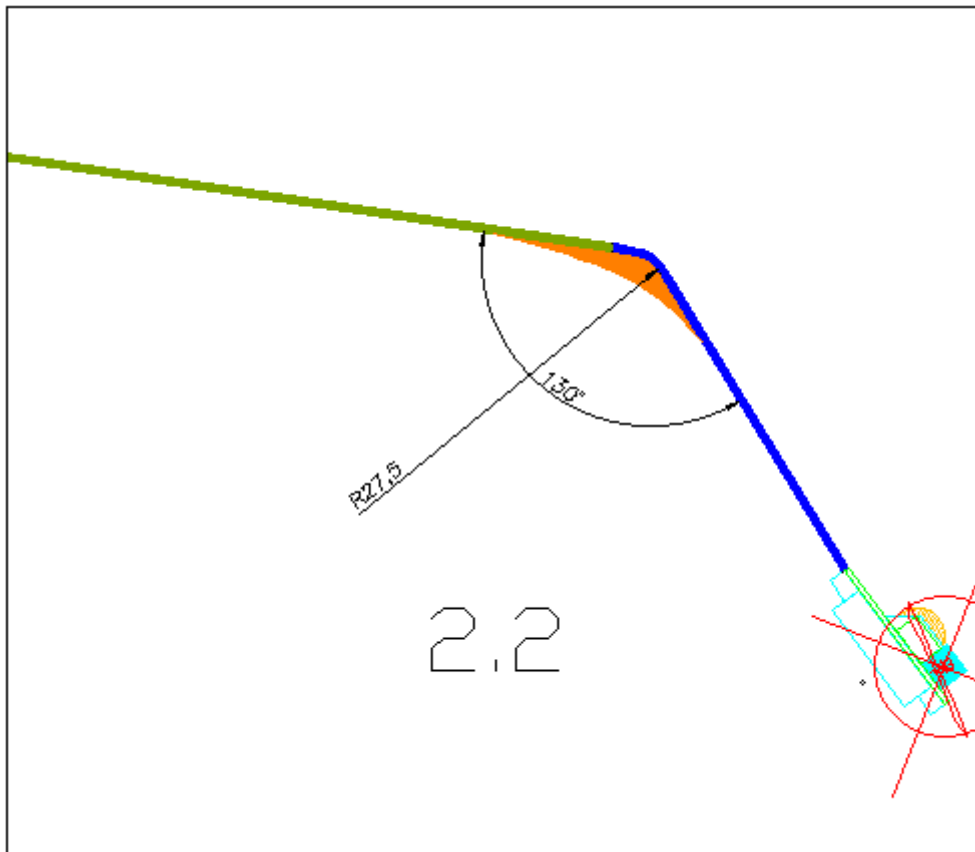
Figura 7 | Esempio di allargamenti in curva
