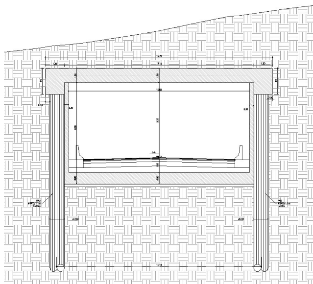
Figura 2: Sezione trasversale della galleria
