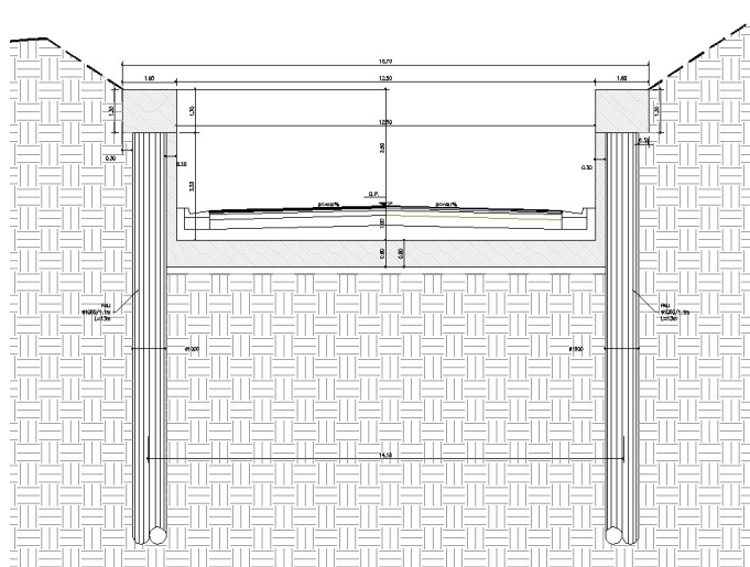
Figura 3: Sezione trasversale degli imbocchi
