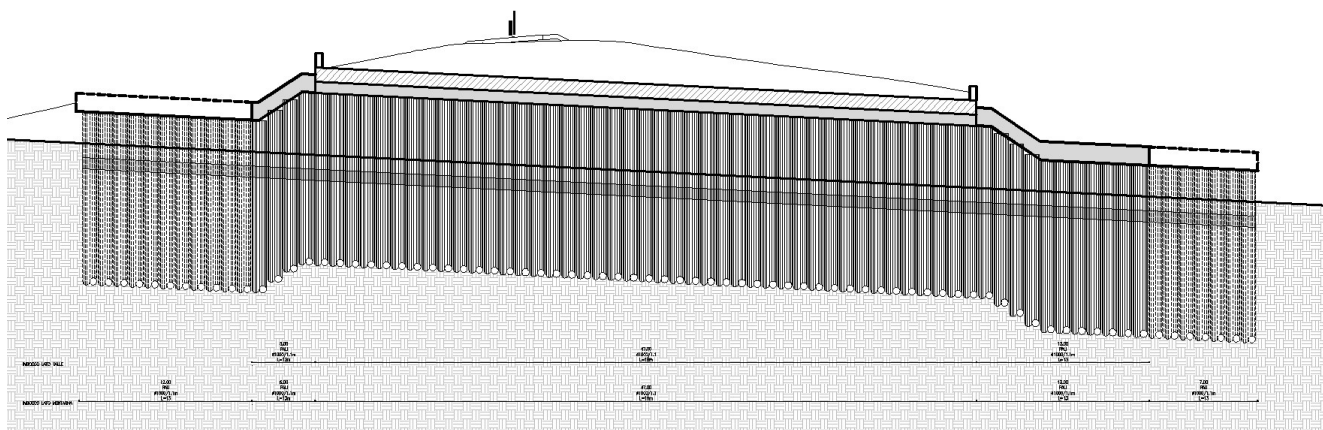
Figura 1: Profilo longitudinale dell'opera
