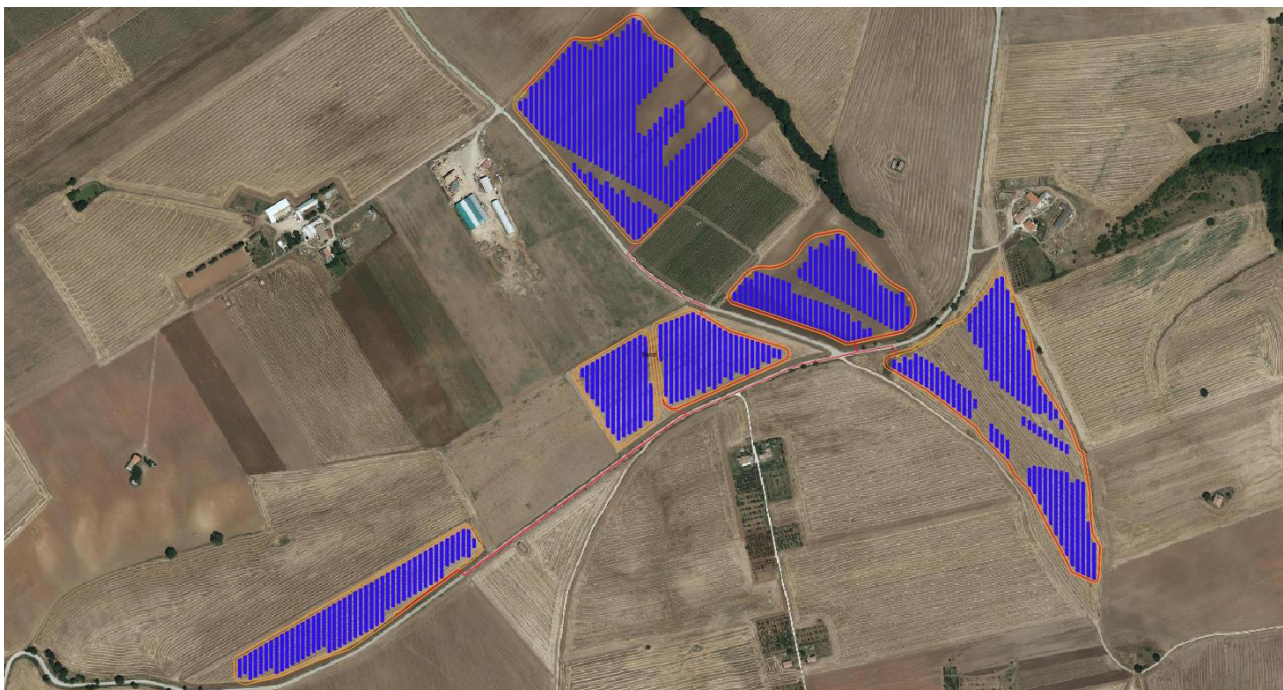
Figura 3.2. – Layout del sistema agrivoltaico con tracker.
