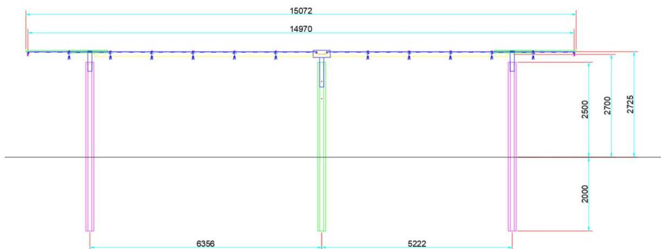
Figura 2.4 – Sezione longitudinale.
