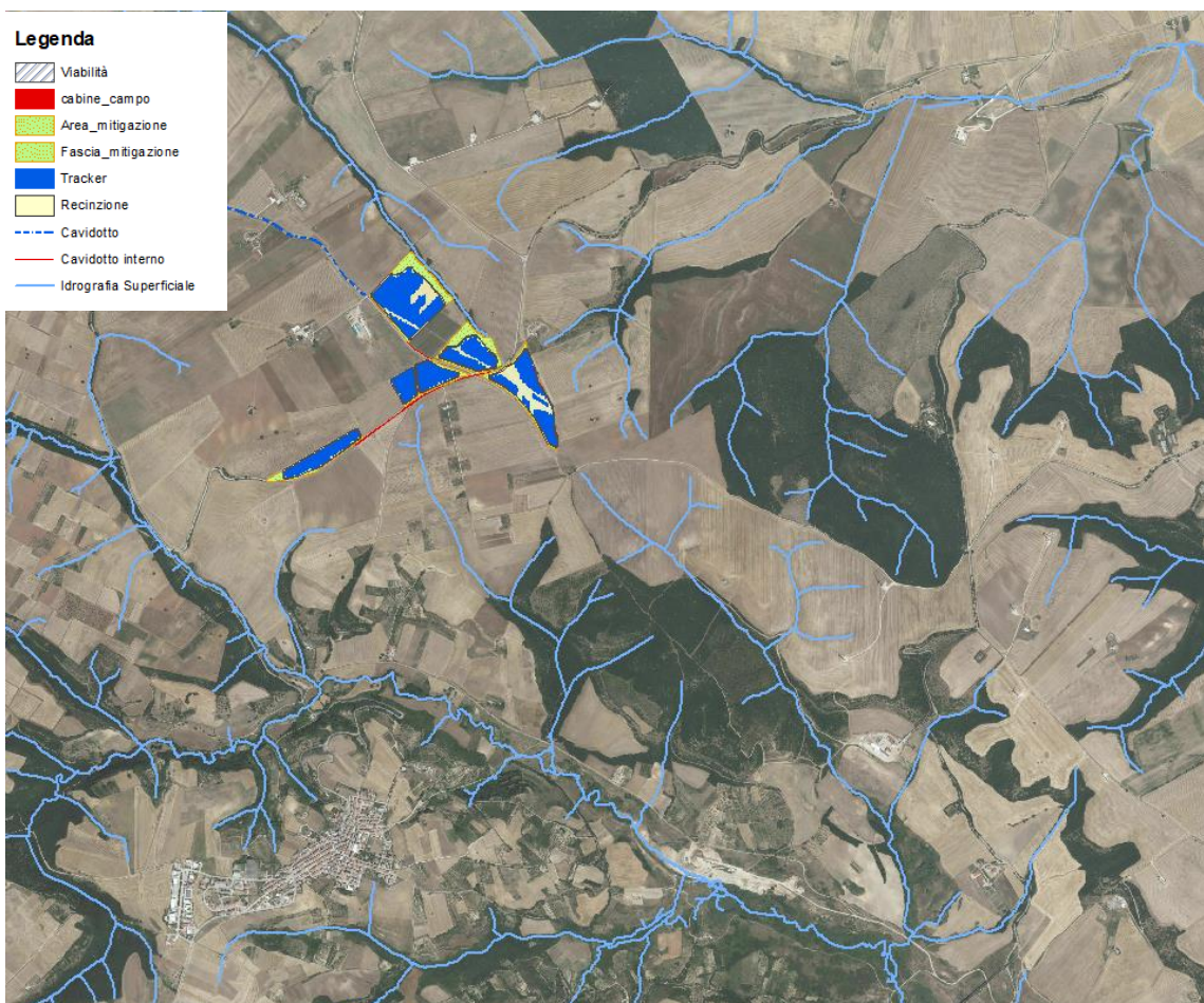
Figura 1.11. – Idrografia dell'area.
