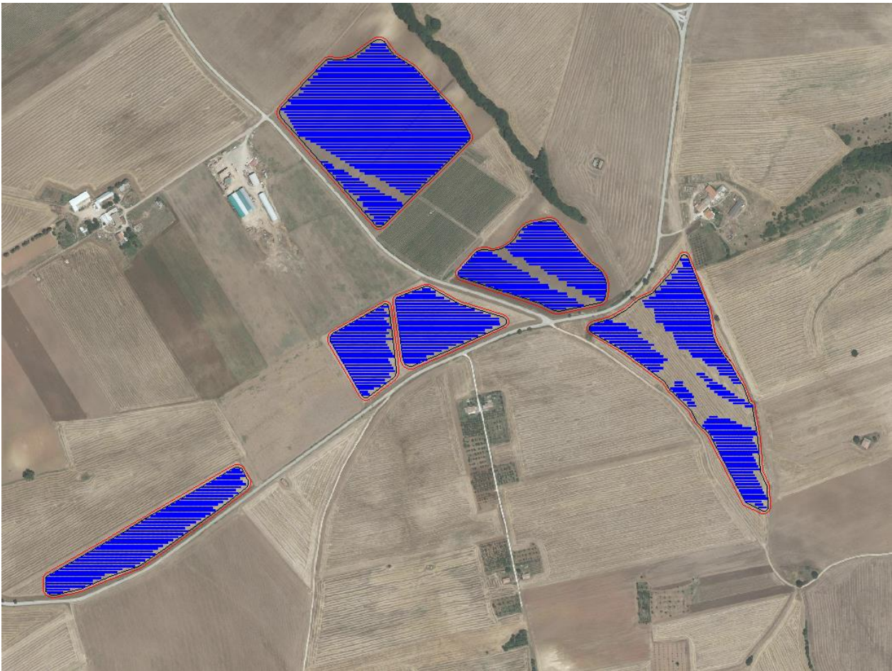
Figura 3.5. – Layout del sistema fotovoltaico con supporti fissi (area ovest).
