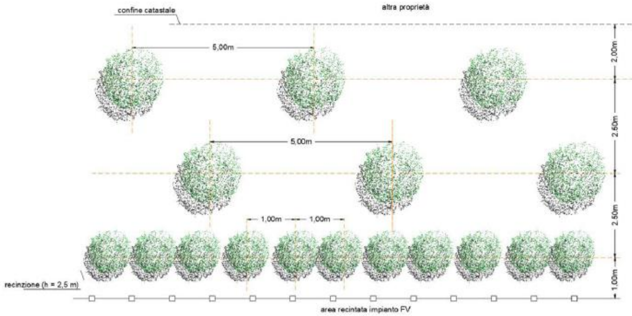
Figura 12.2. – Siepe polispecifica (planimetria di progetto) – siepe e doppio filare di olivo.
