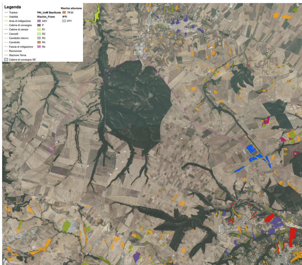
Figura 3.6. – Stralcio Carta delle aree a rischio frane e alluvioni: localizzazione impianto e sottostazioni.
