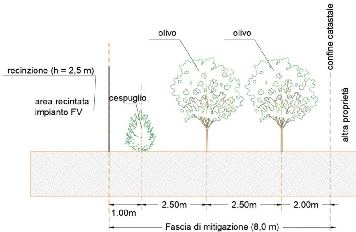
Figura 12.3. – Stralcio di sezione dell'area perimetrale dell'impianto – siepe e doppio filare di olivo.
