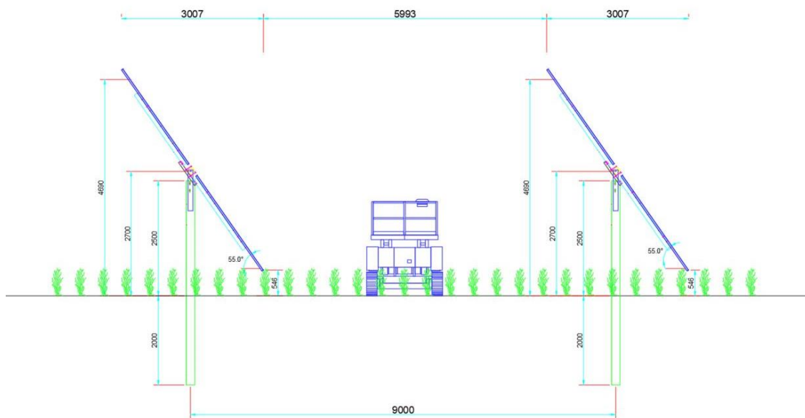
Figure 12.5. – Sezione tipo Aree coltivate.
