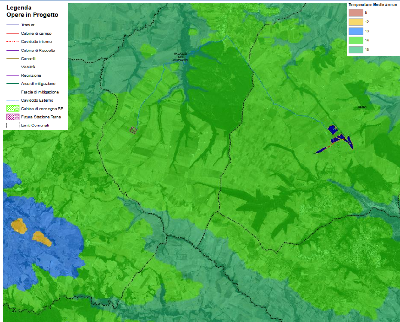
Figura 5.7. – Temperature Medie Annue area di progetto.
