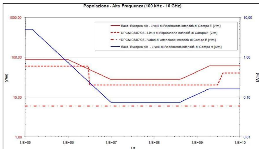
Figura 3.14. – Livelli esposizione Alta Frequenza (100Hz – 10 GHz).
