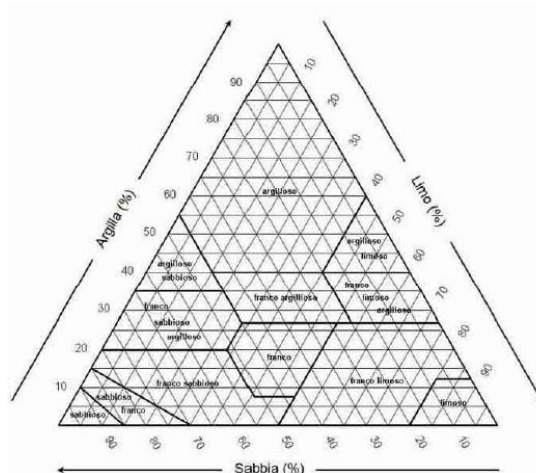
Figura 3.8. – Classificazione Tessitura del terreno USDA.
