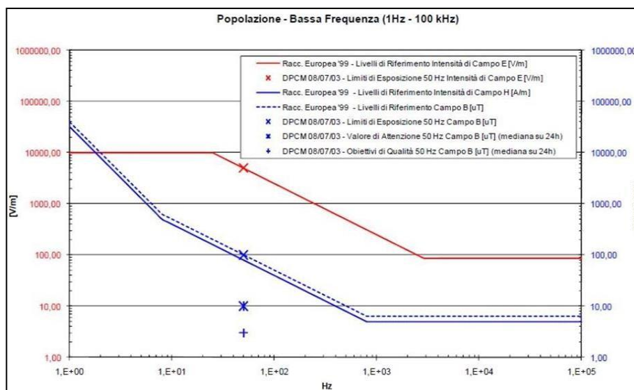
Figura 3.13. – Livelli esposizione Bassa Frequenza (1Hz – 100 kHz).
