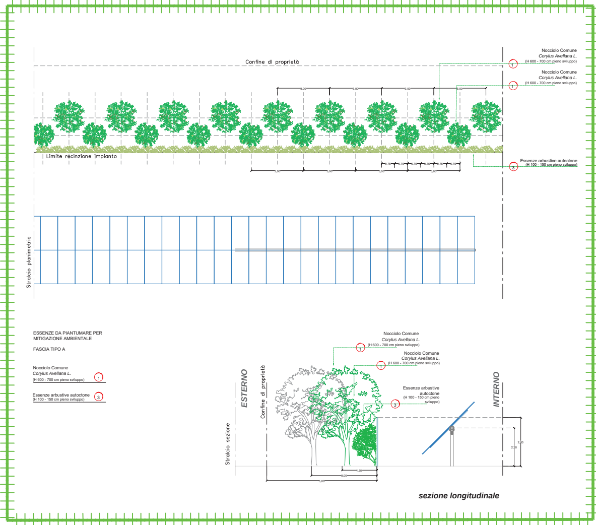
FASCIA DI MITIGAZIONE TIPOLOGIA A lunghezza complessiva fascia 3120,20 m
