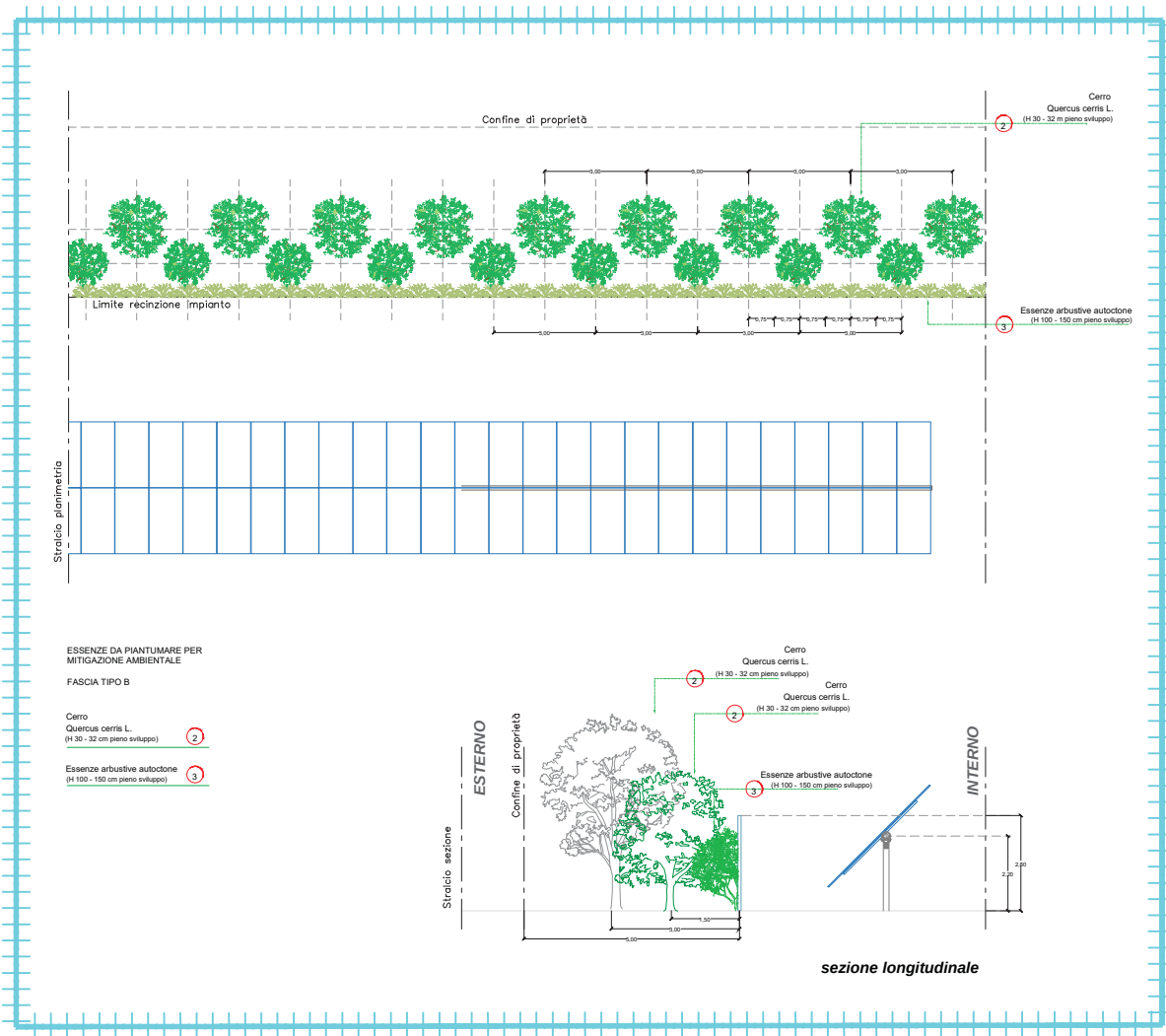
FASCIA DI MITIGAZIONE TIPOLOGIA B - FASCIA DI RICUCITURA CON VEGETAZIONE ESISTENTE lunghezza complessiva fascia 1567,19m
