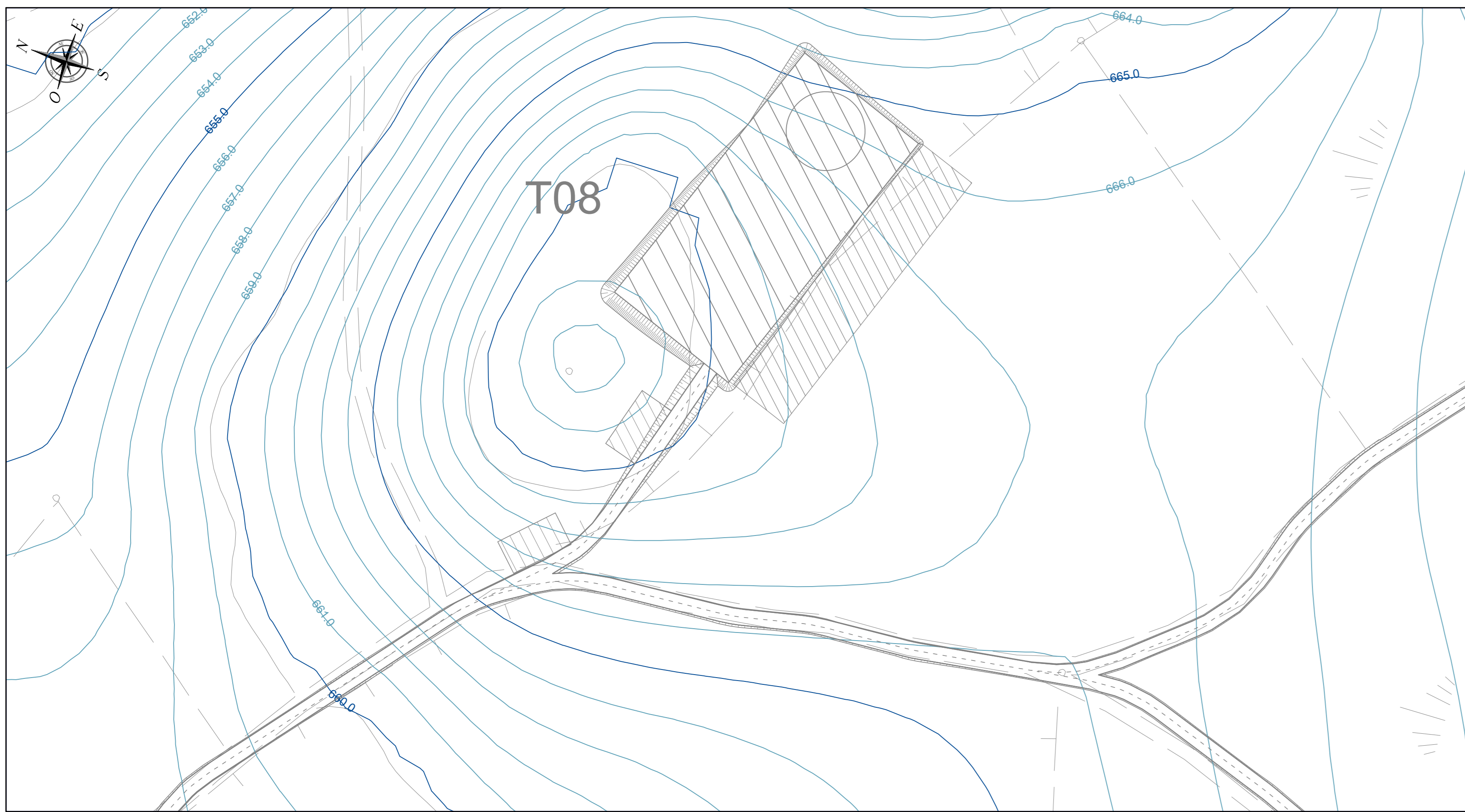
PLANIMETRIA QUADRO 16 - SCALA 1:1.000
