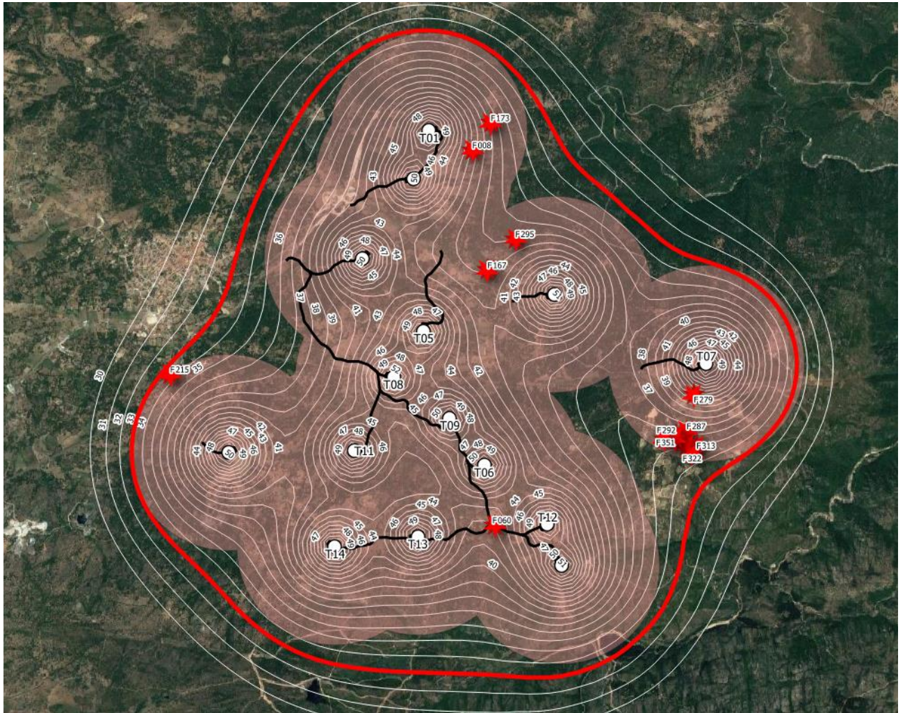
Figura 2.5 – Campo sonoro generato dall’impianto. In rosso l’isofonica dei 33 dBA, attestata ad una distanza indicativa di 1.000 m dalle postazioni eoliche in progetto. In giallo le postazioni eoliche e in rosso i potenziali ricettori.
