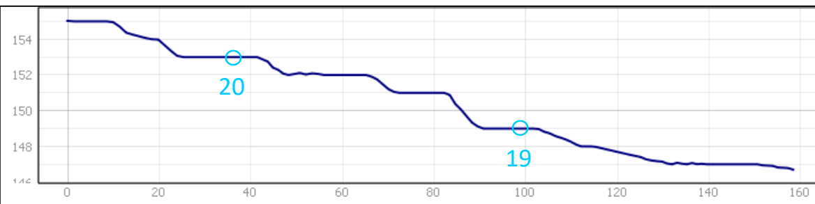
Profilo planoaltimetrico affluente in dx idraulica di V° ordine al f. Gornalunga – fuori scala
