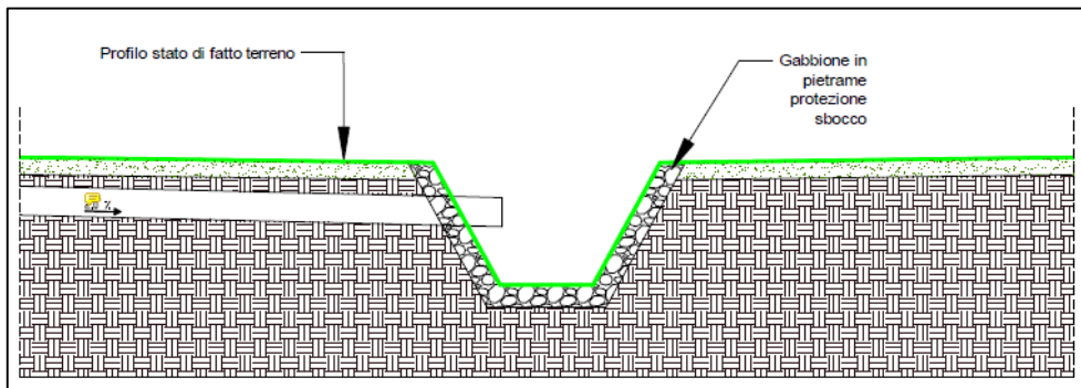
Sezione tipo recapito al corpo idrico recettore – fuori scala
