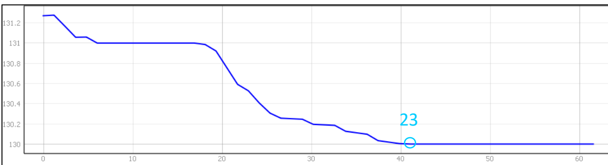
Profilo planoaltimetrico affluente in sx idraulica di IV° ordine al f. Gornalunga – fuori scala
