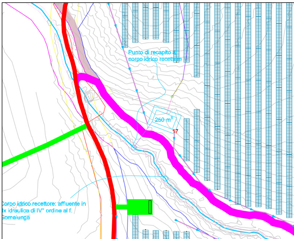
Planimetria affluente in dx idraulica di IV° ordine al f. Gornalunga – fuori scala
