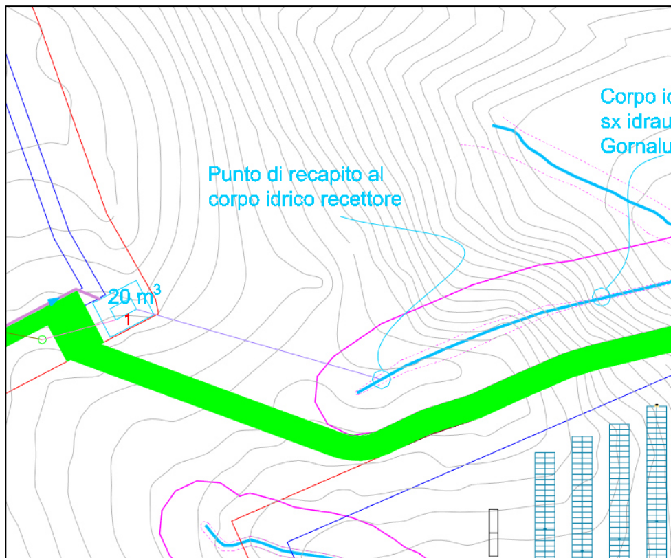
Planimetria affluente in sx idraulica di V° ordine al f. Gornalunga – fuori scala
