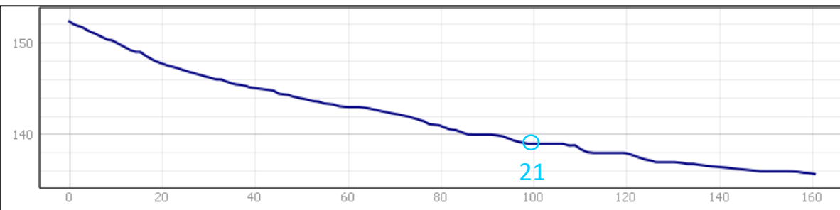
Profilo planoaltimetrico affluente in dx idraulica di V° ordine al v.ne sbarda l'asino – fuori scala
