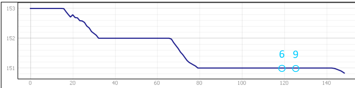
Profilo planoaltimetrico affluente in sx idraulica di IV° ordine al f. Gornalunga – fuori scala
