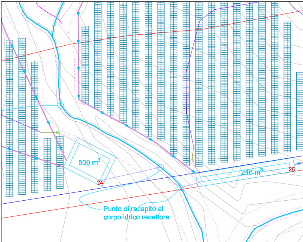
Planimetria affluente in sx idraulica di IV° ordine al f. Gornalunga – fuori scala
