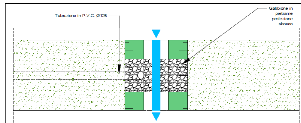
Particolare in Pianta recapito al corpo idrico recettore – fuori scala
