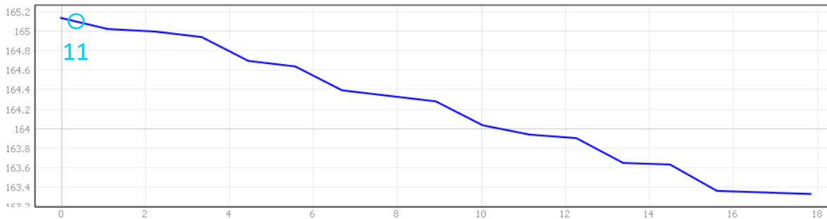
Profilo Planoaltimetrico affluente in dx idraulica di V° ordine al f. Gornalunga – fuori scala
