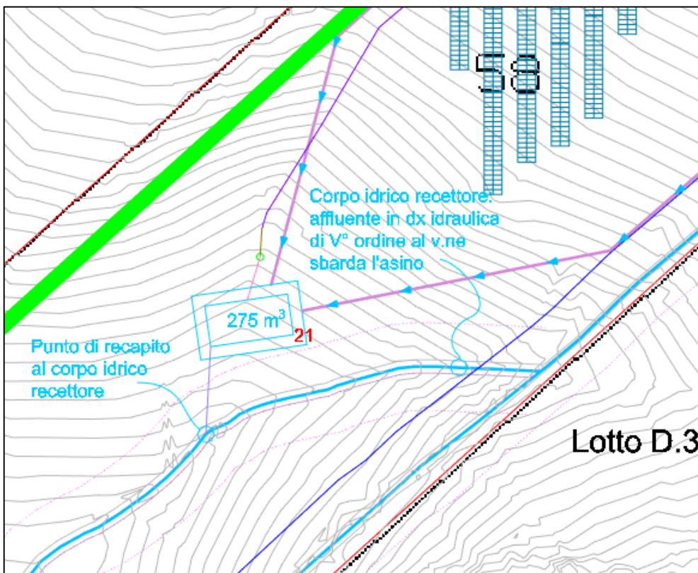
Planimetria affluente in dx idraulica di V° ordine al v.ne sbarda l'asino – fuori scala
