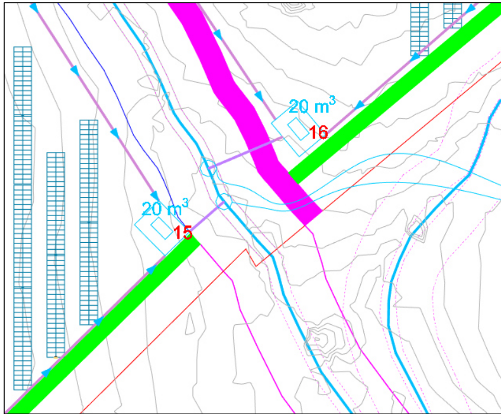
Planimetria affluente in dx idraulica di V° ordine al f. Gornalunga– fuori scala
