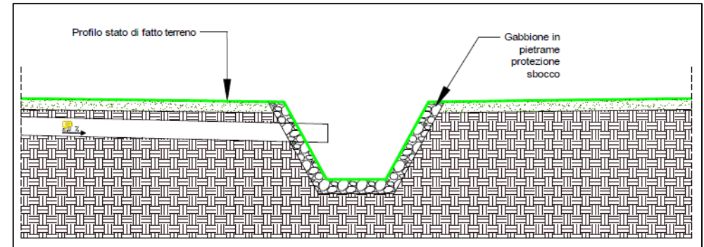
Sezione tipo recapito al corpo idrico recettore – fuori scala
