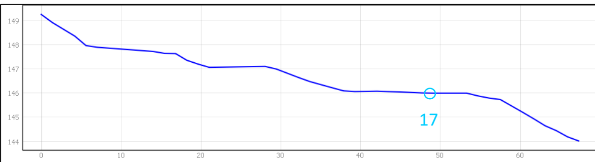
Profilo planoaltimetrico affluente in dx idraulica di IV° ordine al f. Gornalunga – fuori scala
