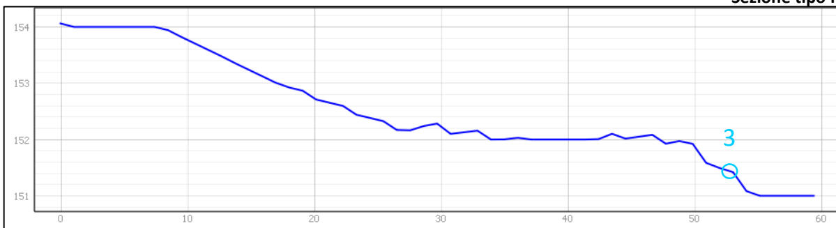
Profilo planoaltimetrico affluente in sx idraulica di V° ordine al f. Gornalunga – fuori scala
