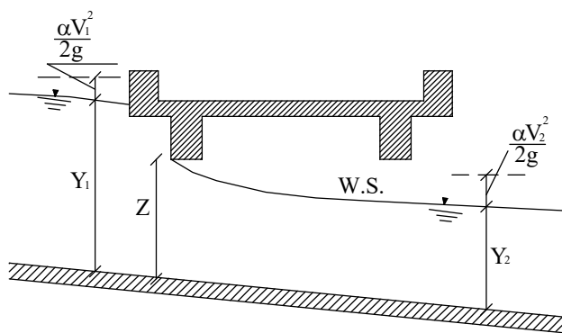
Figura 31 - Sezione schematica di un ponte – Schema di calcolo
