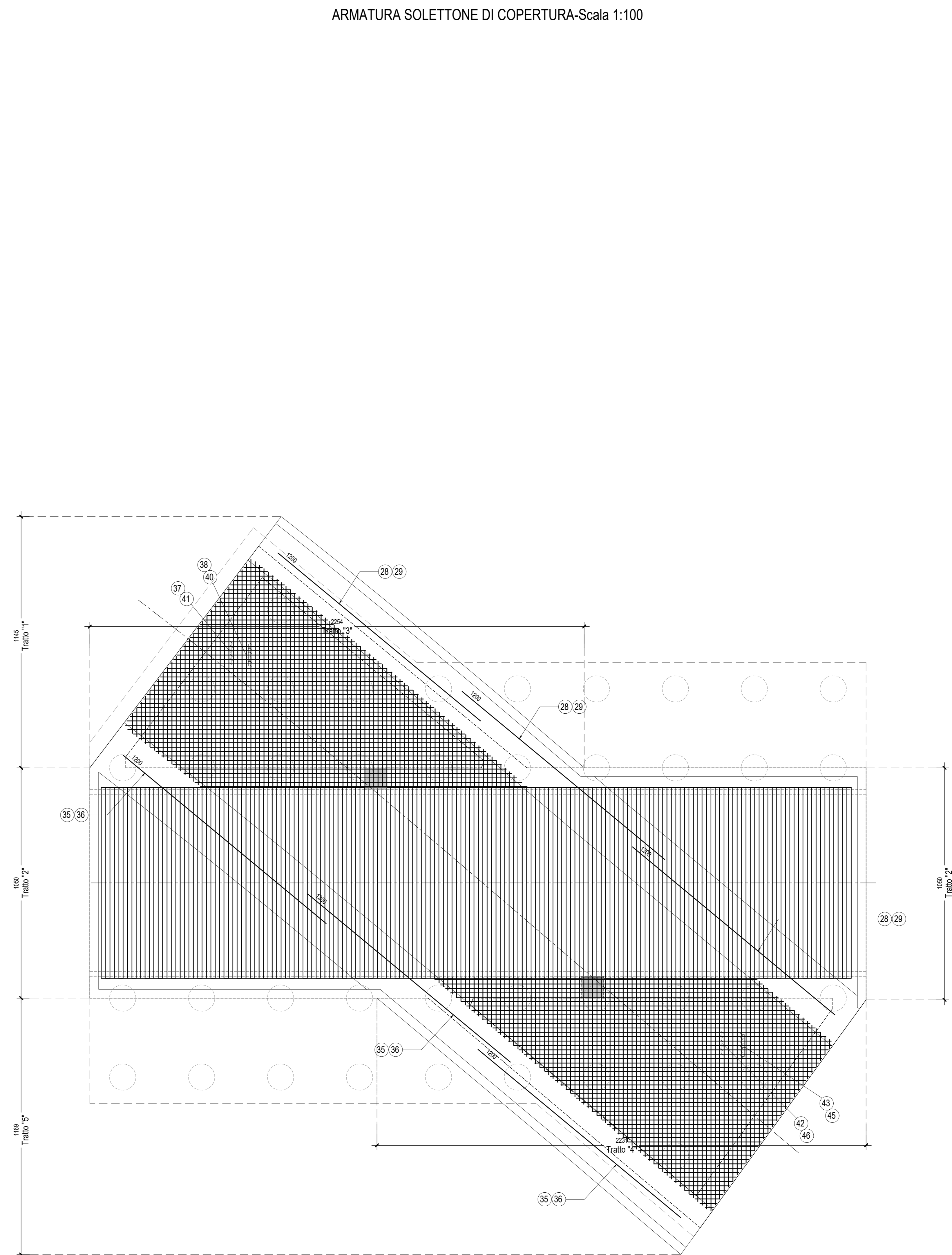
ARMATURA SOLETTONE DI COPERTURA-Scala 1:100
