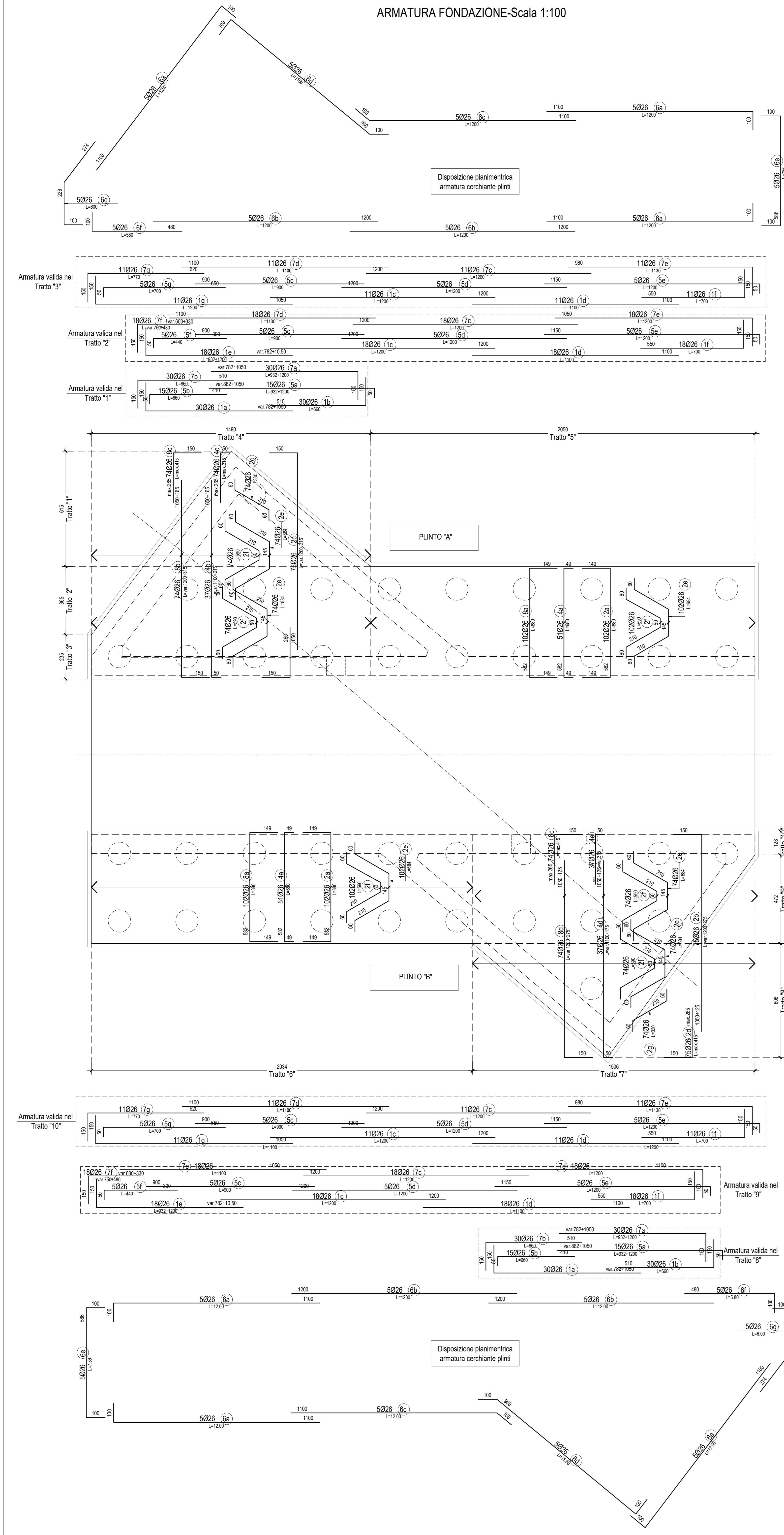
ARMATURA FONDAZIONE-Scala 1:100
