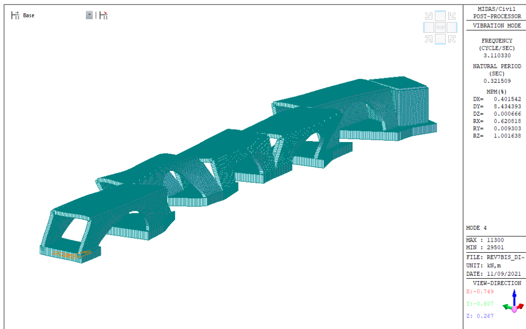
Figura 48: Deformata modo di vibrazione n° 4
