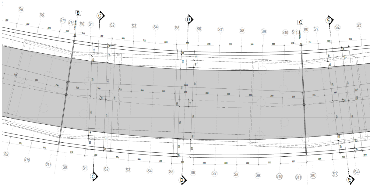
Figura 6: Pianta impalcato – Campata B/C.
