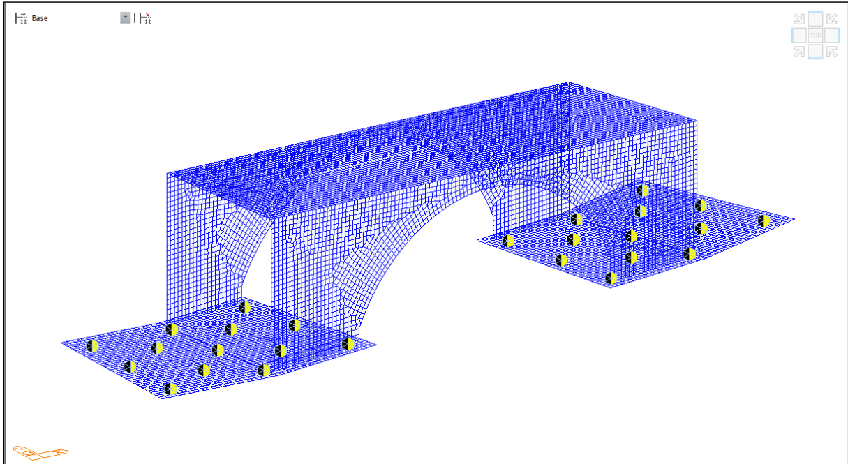
Figura 11: Modello: Vista Campata B/C con vincoli
