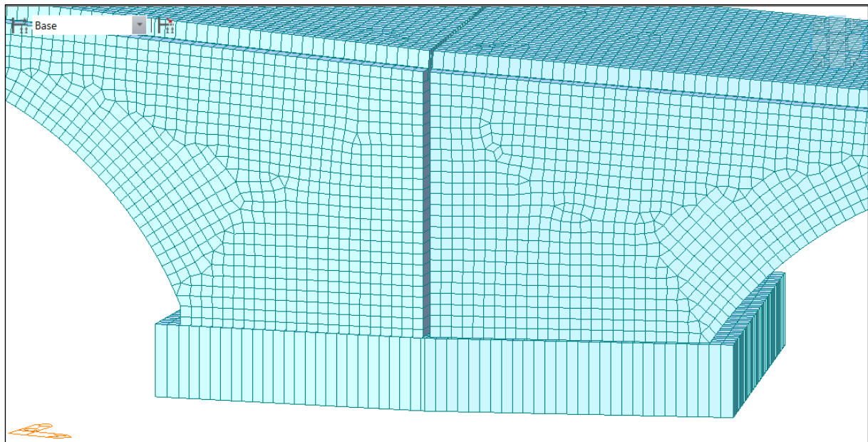
Figura 14: Modello: Particolare giunto strutturale
