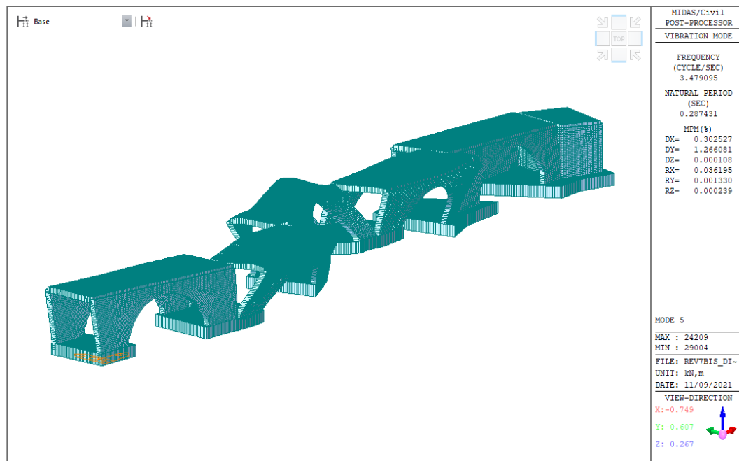
Figura 49: Deformata modo di vibrazione n° 5
