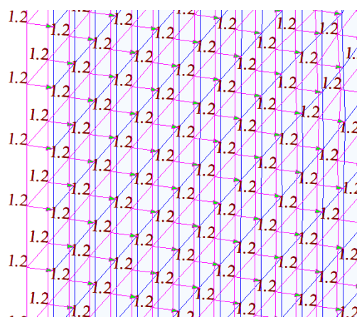
Figura 32: Azione del vento a ponte scarico
