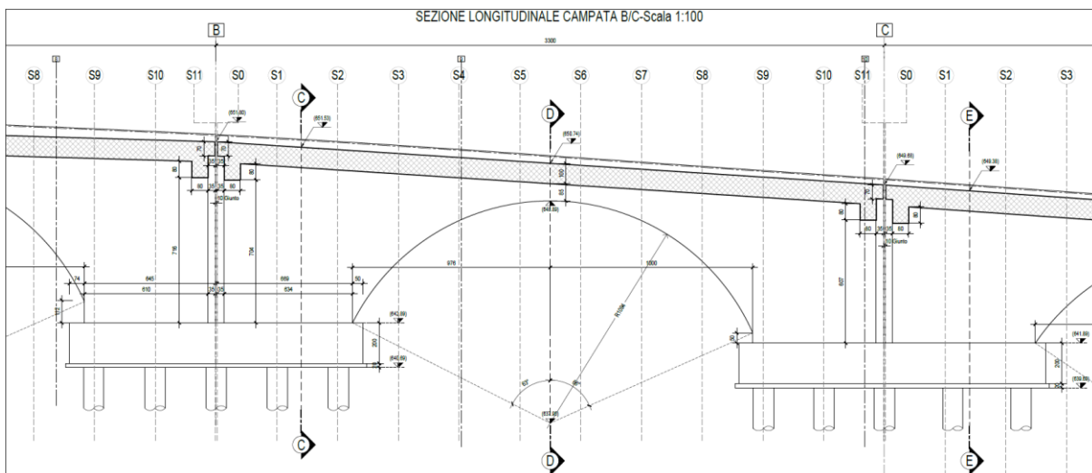
Figura 5: Sezione longitudinale – Campata B/C.
