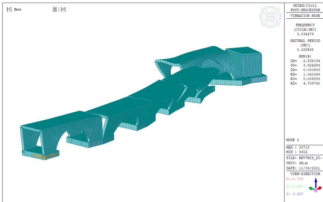
Figura 47: Deformata modo di vibrazione n° 3
