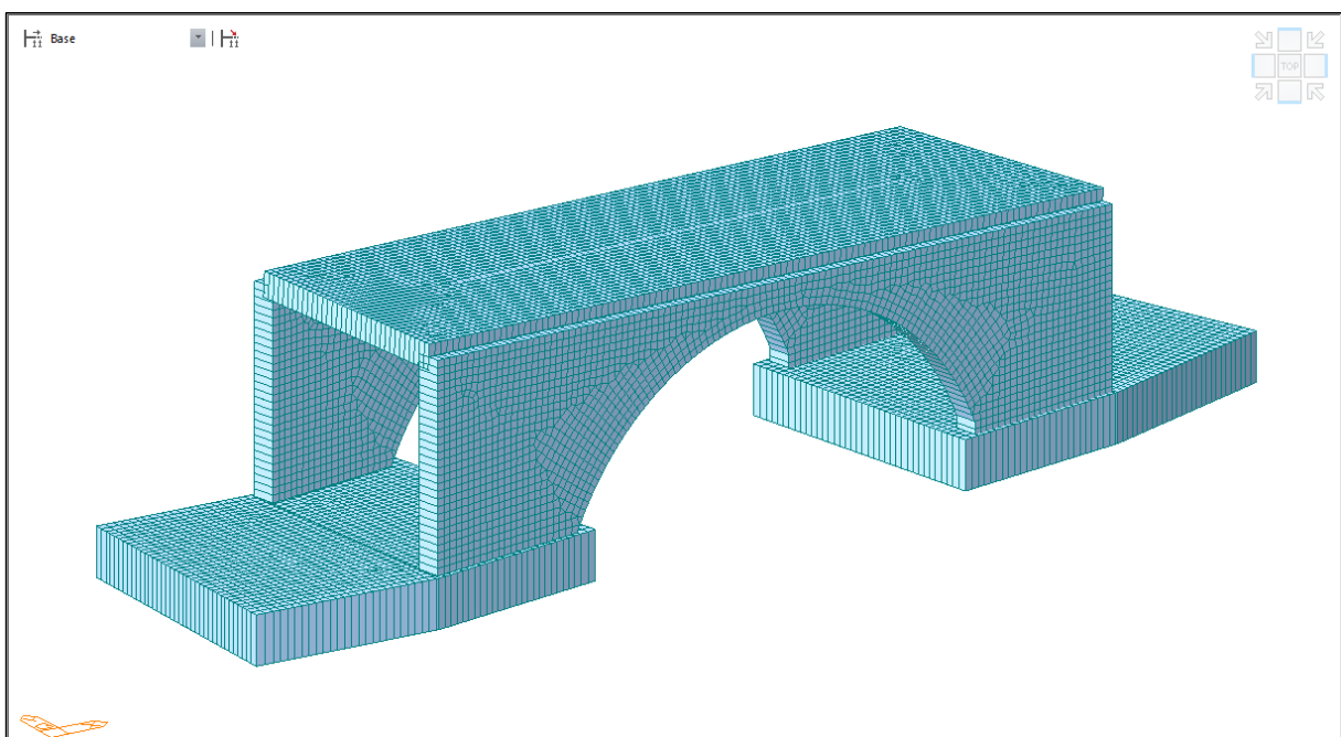
Figura 12: Modello: Vista Campata B/C con spessori elementi strutturali
