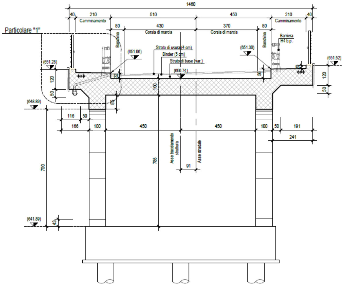
Figura 8: Sezione trasversale in corrispondenza della mezzeria – Campata B/C.
