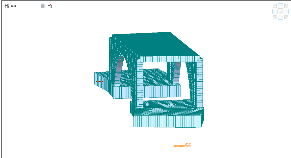
Figura 13: Modello: Vista longitudinale Campata B/C
