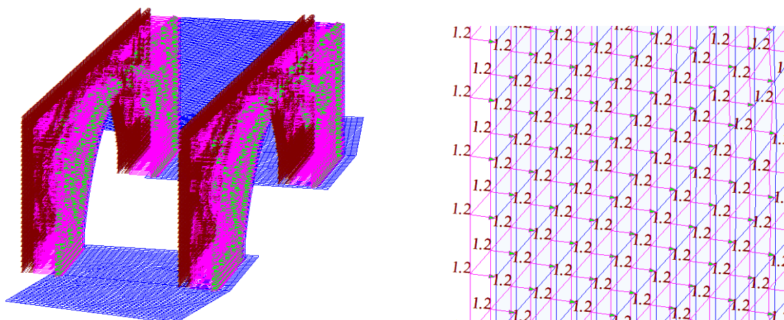
Figura 32: Azione del vento a ponte scarico
