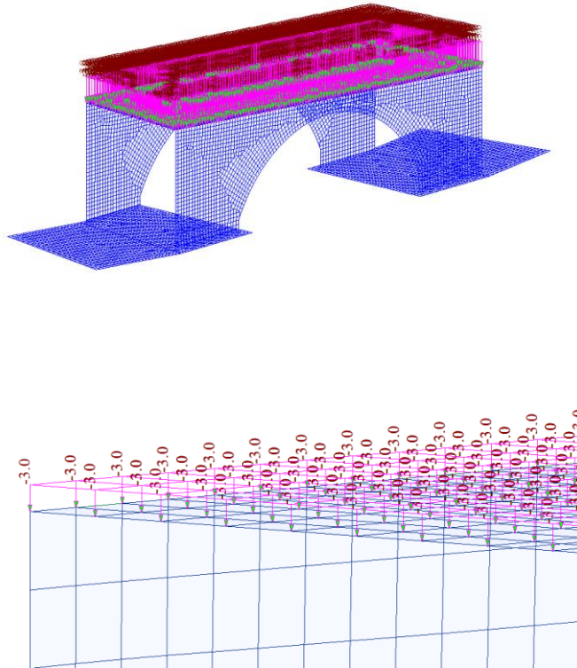
Figura 18: Carichi pavimentazione
