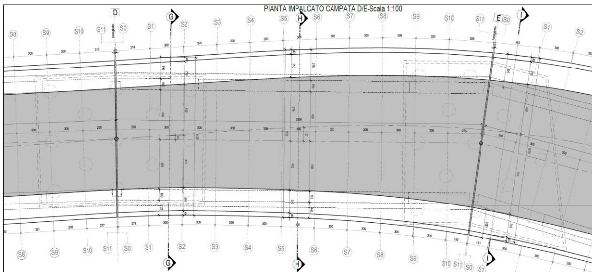
Figura 6: Pianta impalcato – Campata D/E.
