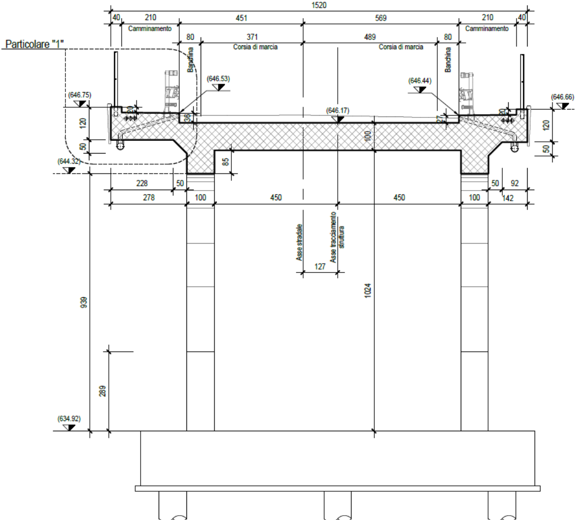
Figura 8: Sezione trasversale in corrispondenza della mezzeria – Campata D/E.
