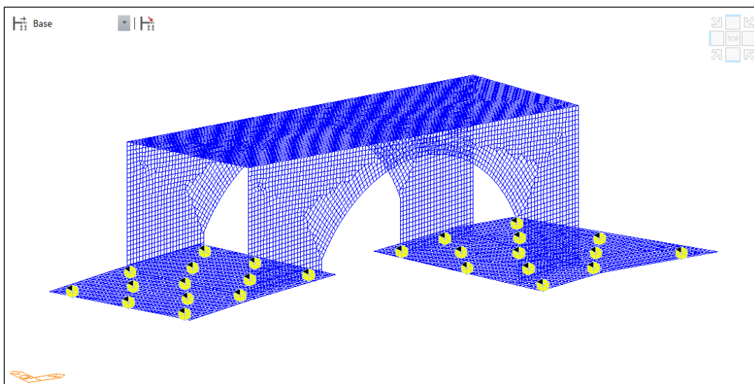
Figura 11: Modello: Vista Campata D/E con vincoli
