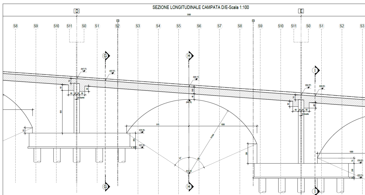
Figura 5: Sezione longitudinale - Campata D/E.
