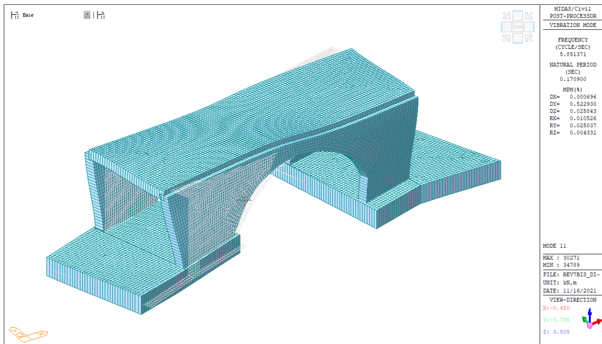
Figura 49: Deformata modo di vibrazione n° 11
