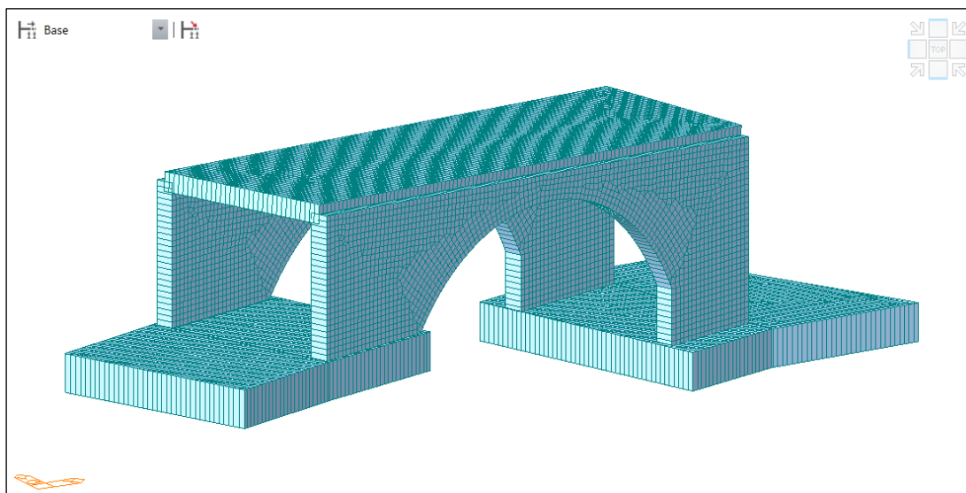
Figura 12: Modello: Vista Campata D/E con spessori elementi strutturali
