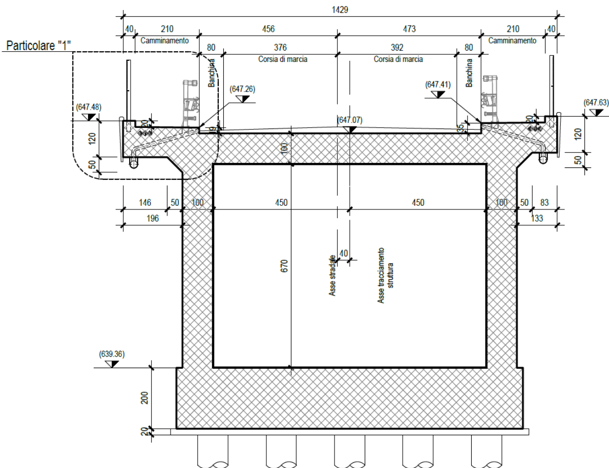
Figura 7: Sezione trasversale in corrispondenza del plinto C – Campata D/E.
