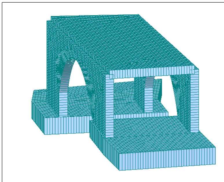
Figura 13: Modello: Vista longitudinale Campata D/E
