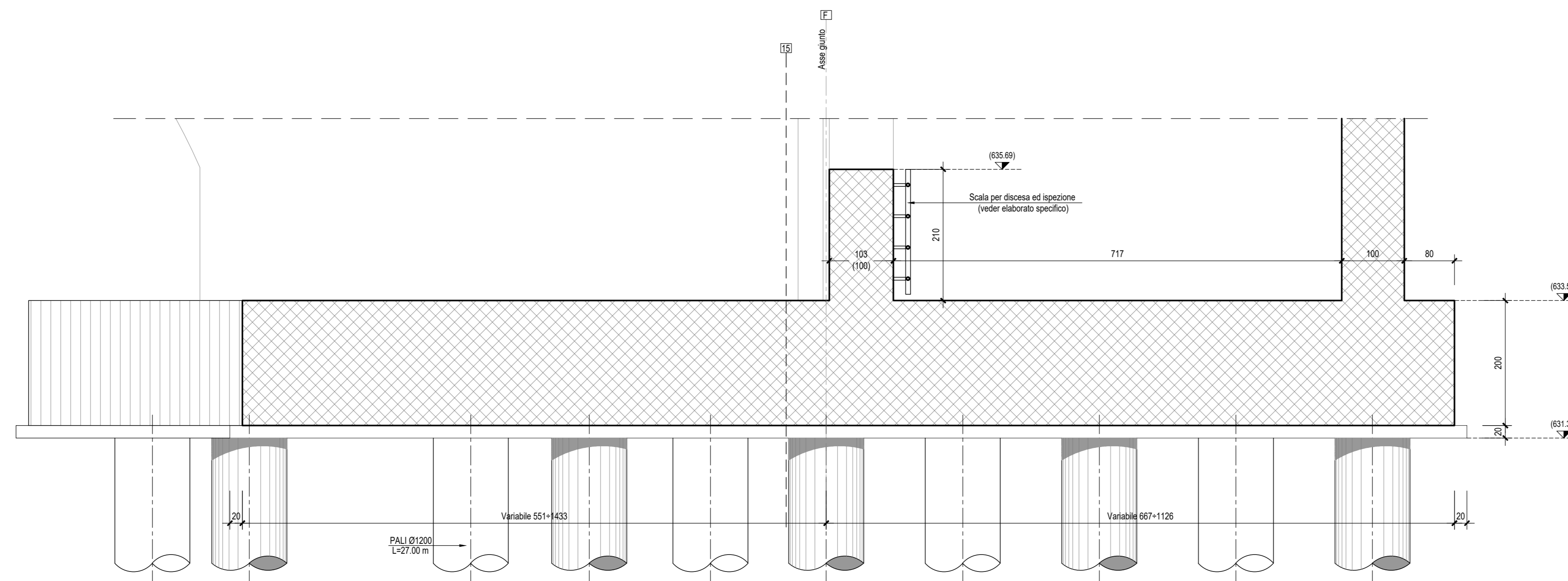
SEZIONE A-A PLINTO "F"-Scala 1:50
