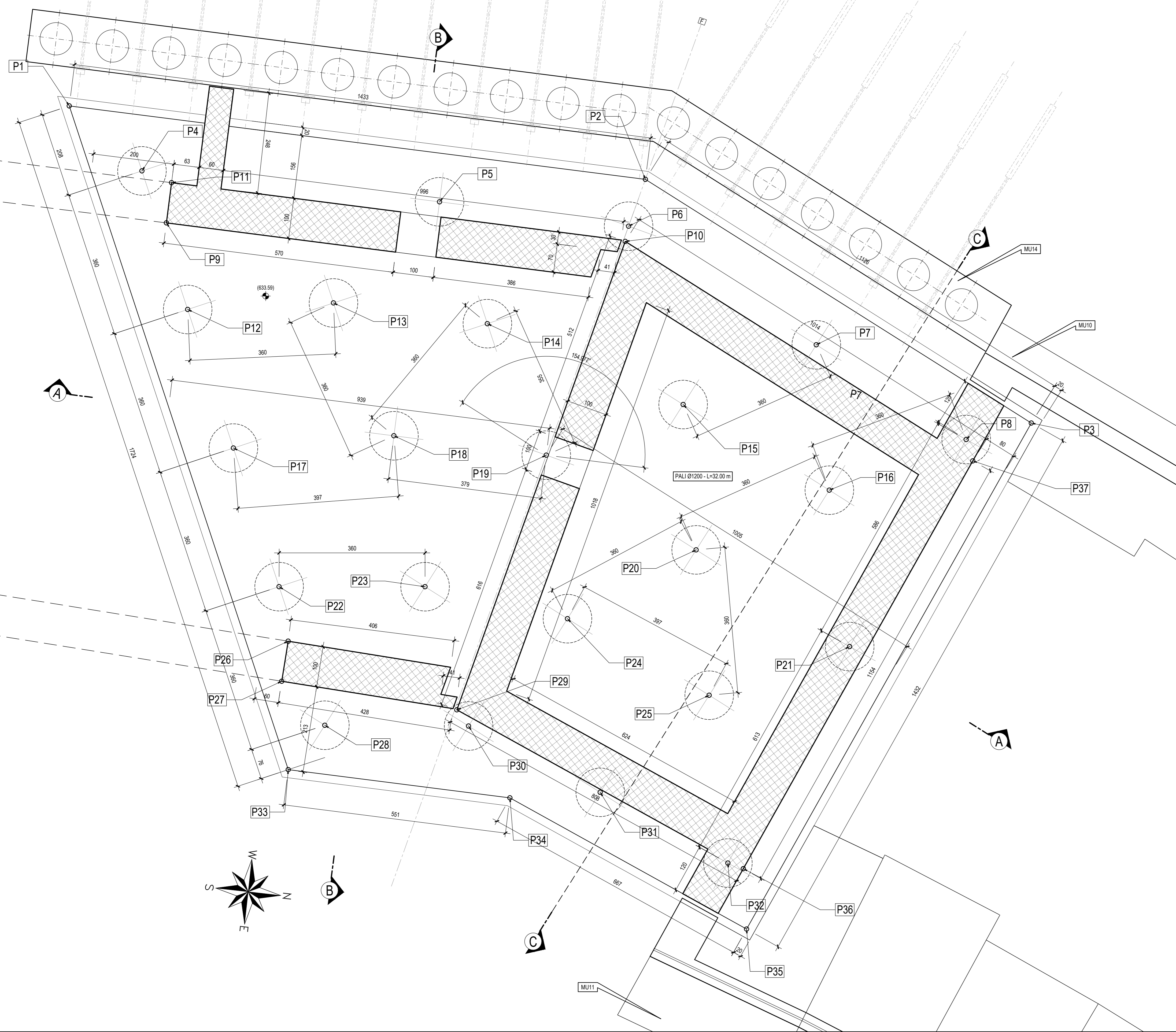
PIANTA FONDAZIONI PLINTO "F"-Scala 1:50
