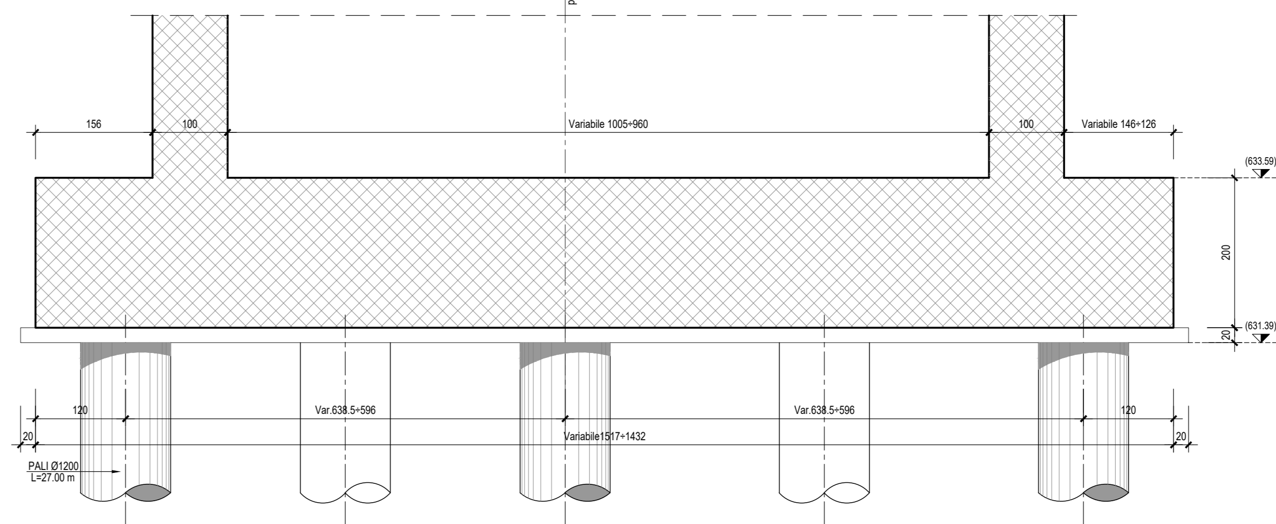
SEZIONE C-C PLINTO "F"-Scala 1:50
