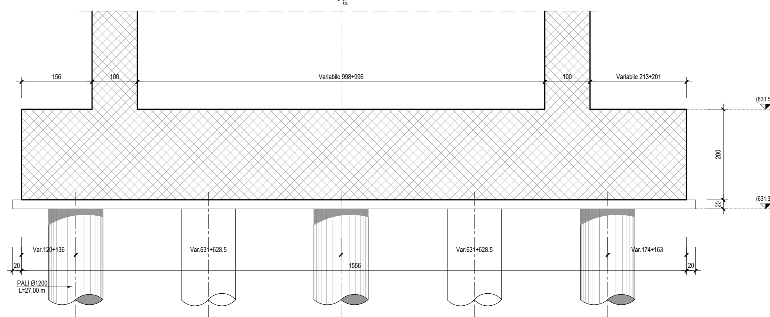
SEZIONE B-B PLINTO "F"-Scala 1:50
