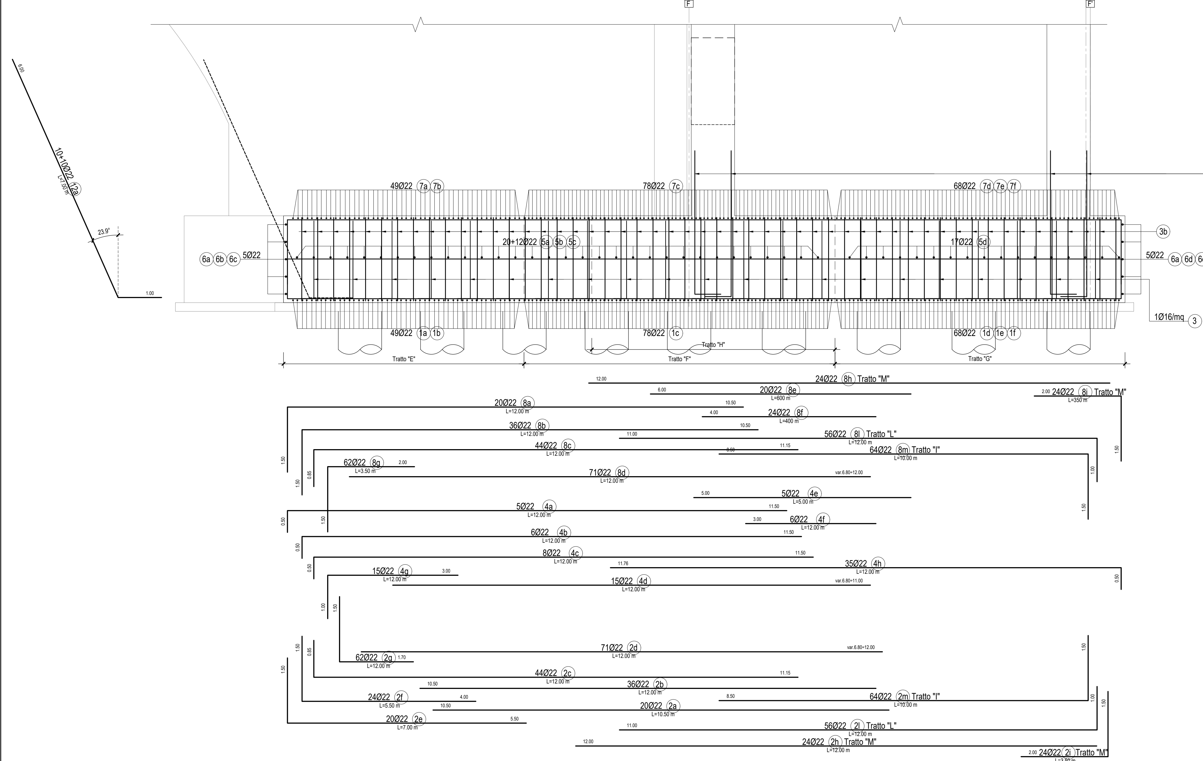
ARMATURA SEZIONE A-A-Scala 1:50
