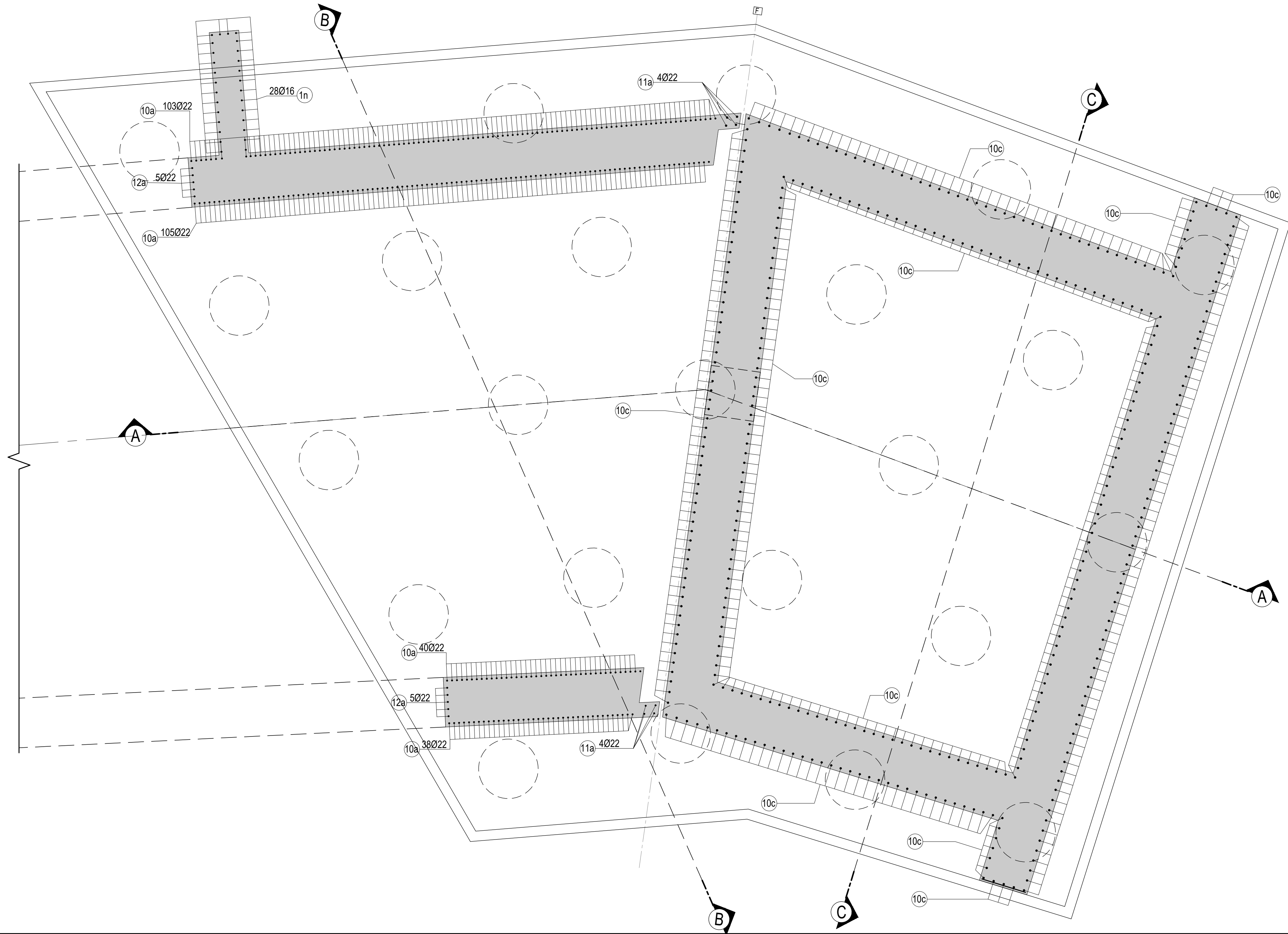
DISPOSIZIONE PLANIMETRICA ARMATURA PLINTO "F"-Scala 1:50
