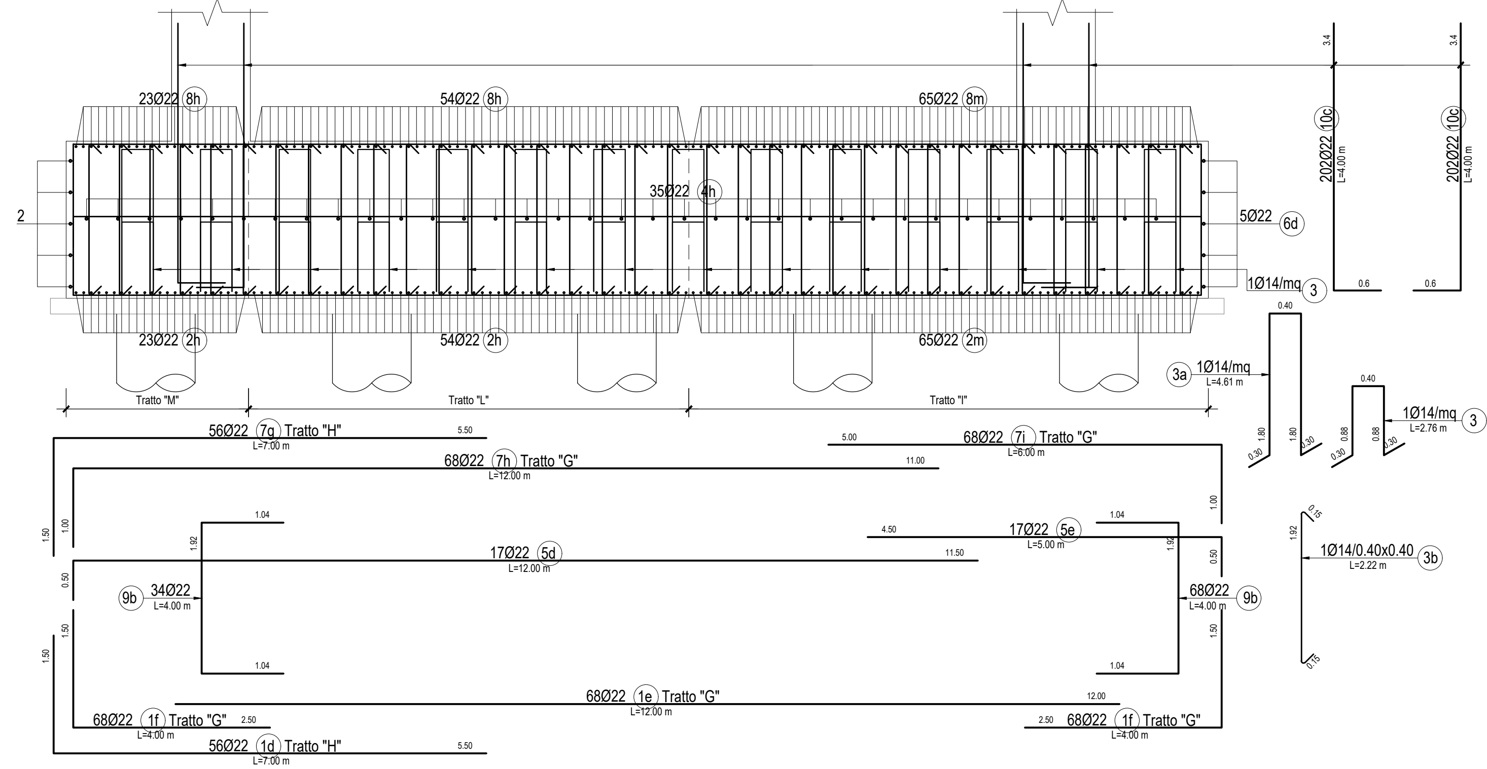
ARMATURA SEZIONE C-C-Scala 1:50
