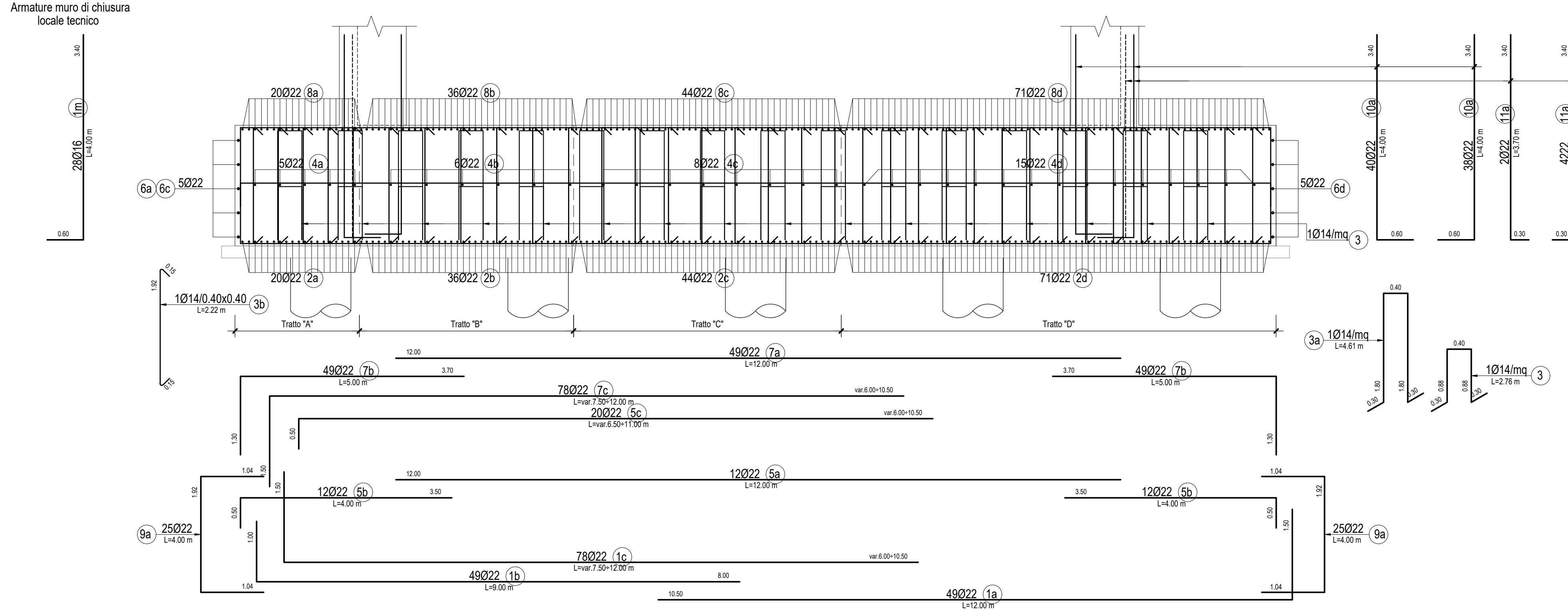
ARMATURA SEZIONE B-B-Scala 1:50
