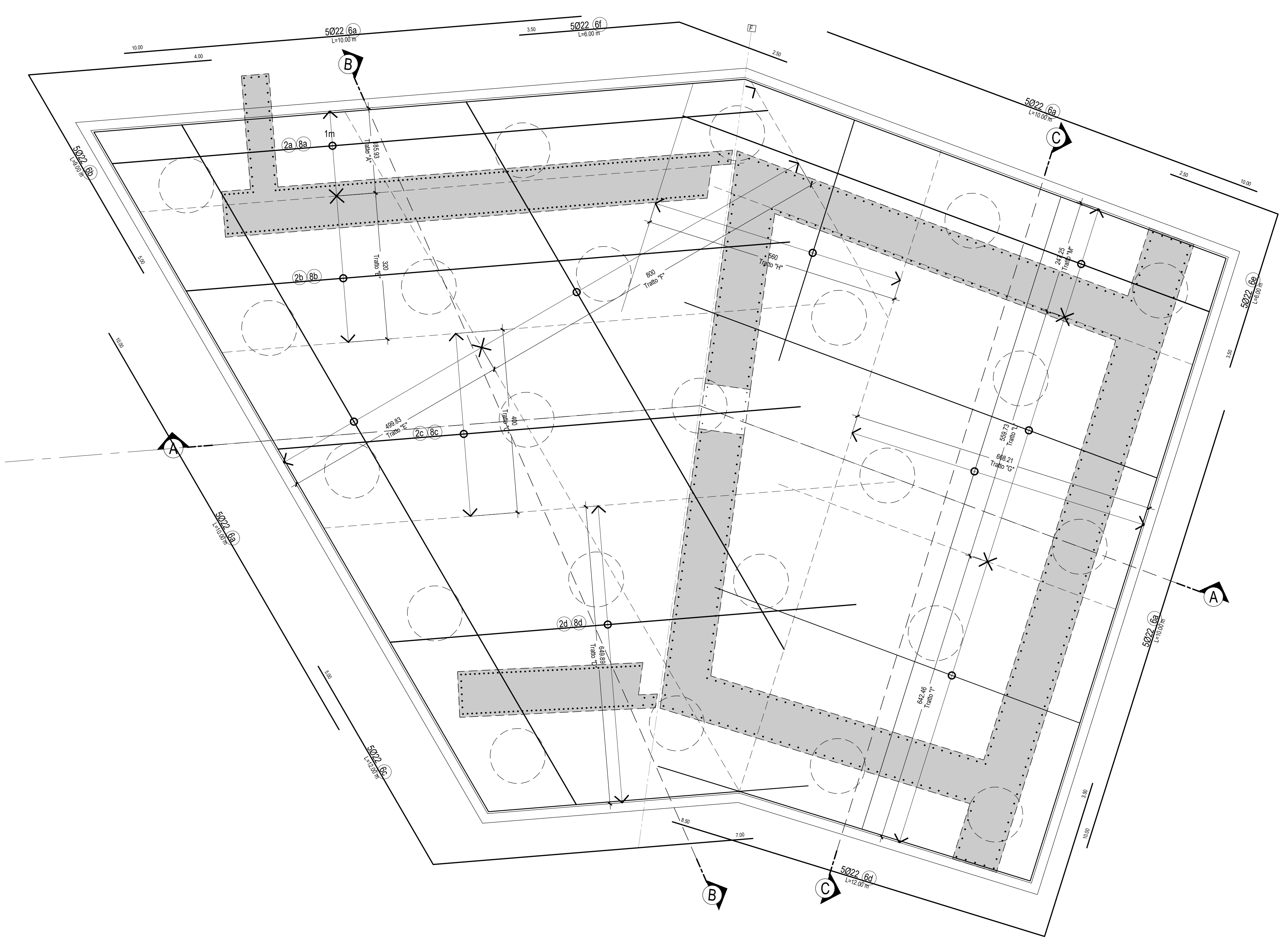
DISPOSIZIONE PLANIMETRICA ARMATURA PLINTO "F"-Scala 1:50
