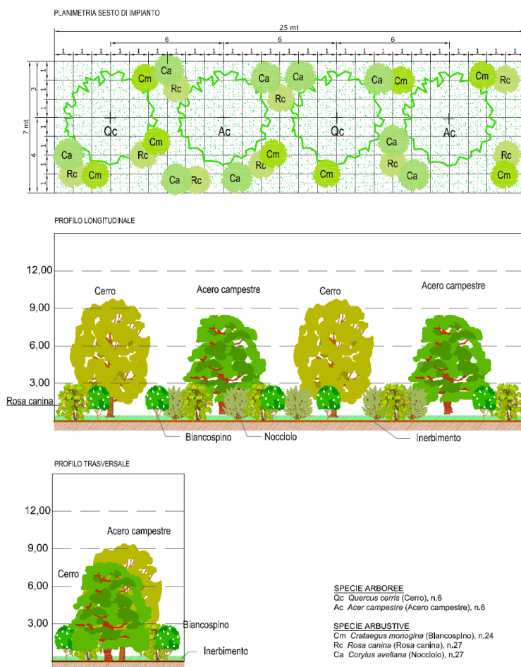
Figura 4-1 Sesto di impianto della fascia arboreo-arbustiva.
