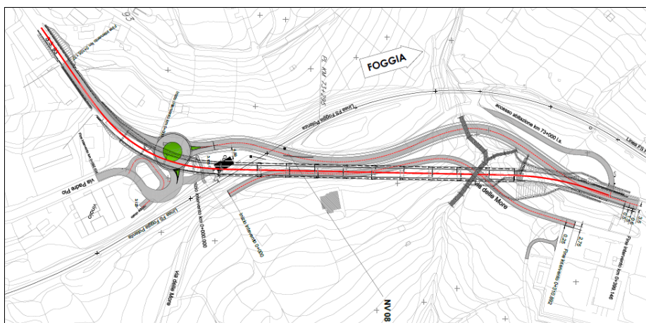
Figure 1-3 Confronto soluzioni viabilità NV08 di PD 2015 e integrazione al PD 2016
