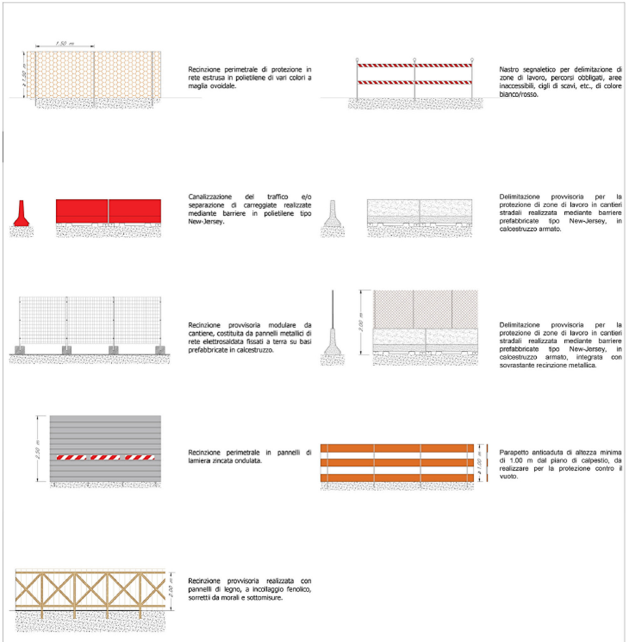
Figura 2-1 Recinzioni tipo
