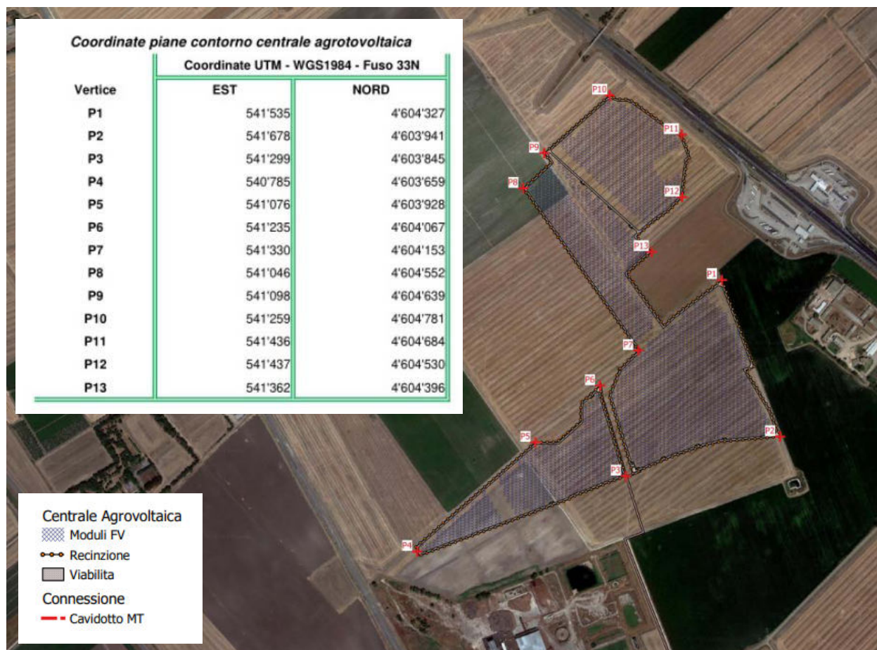
Ortofoto con l'individuazione dell'impianto in progetto, riportante i punti dell'area recintata e le relative coordinate.
