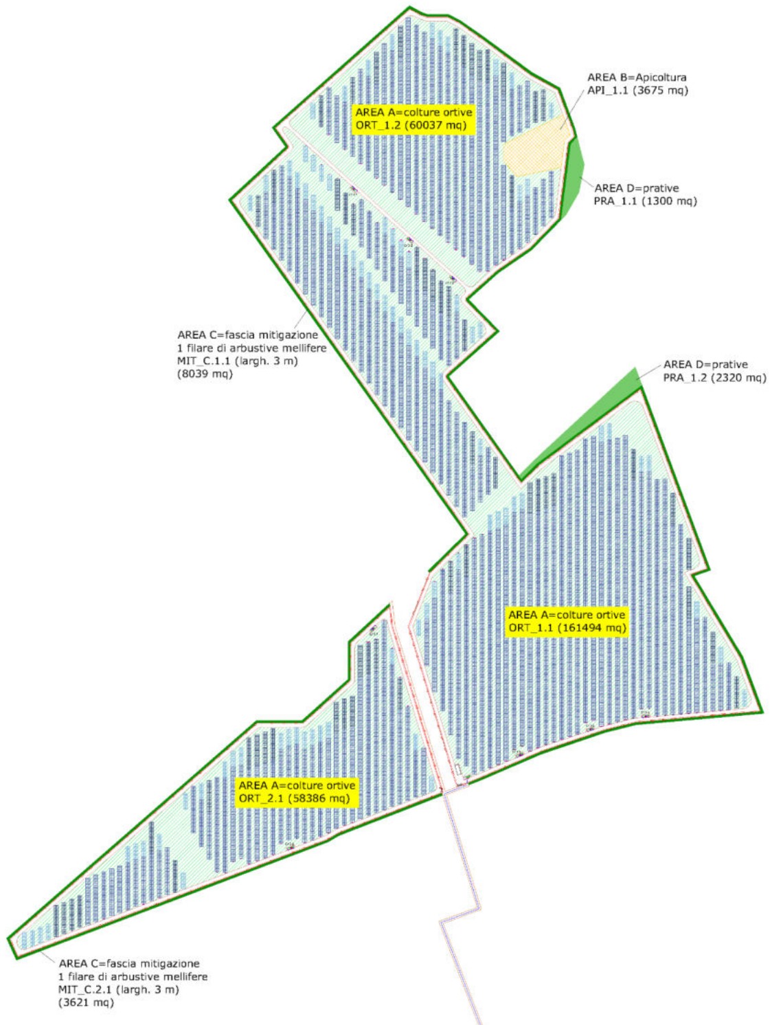
Layout dell'impianto agrovoltaico con l'indicazione delle diverse aree individuate dal progetto agronomico.
