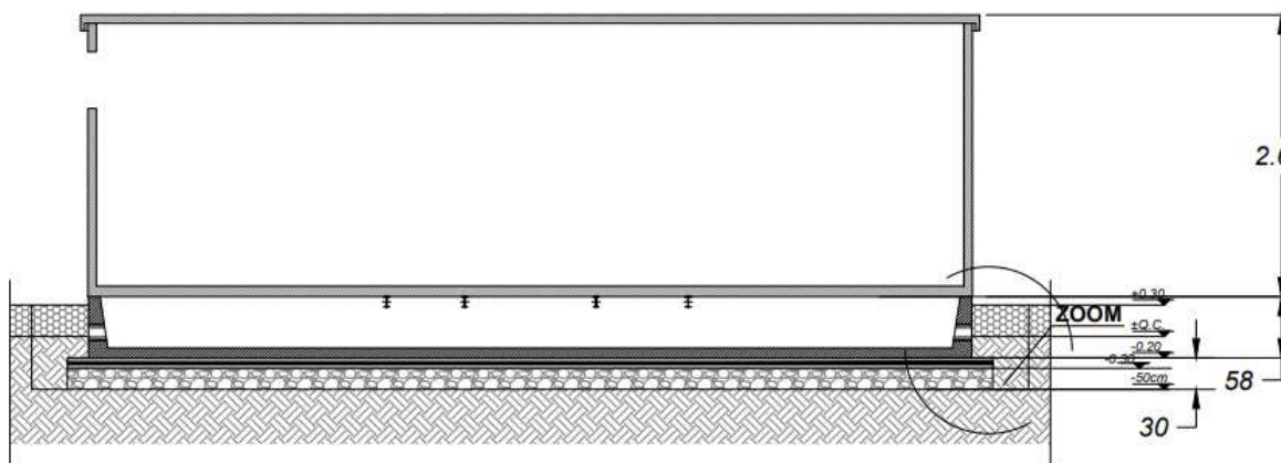
SEZIONE A-A
