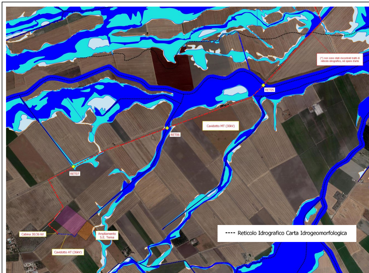
Figura 6 – Cavidotto di vettoriamento e interferenze con reticolo idrografico (da RET05 a RET07) e fasce a pericolosità idraulica del PAI Puglia (aggiornamento 2023)
