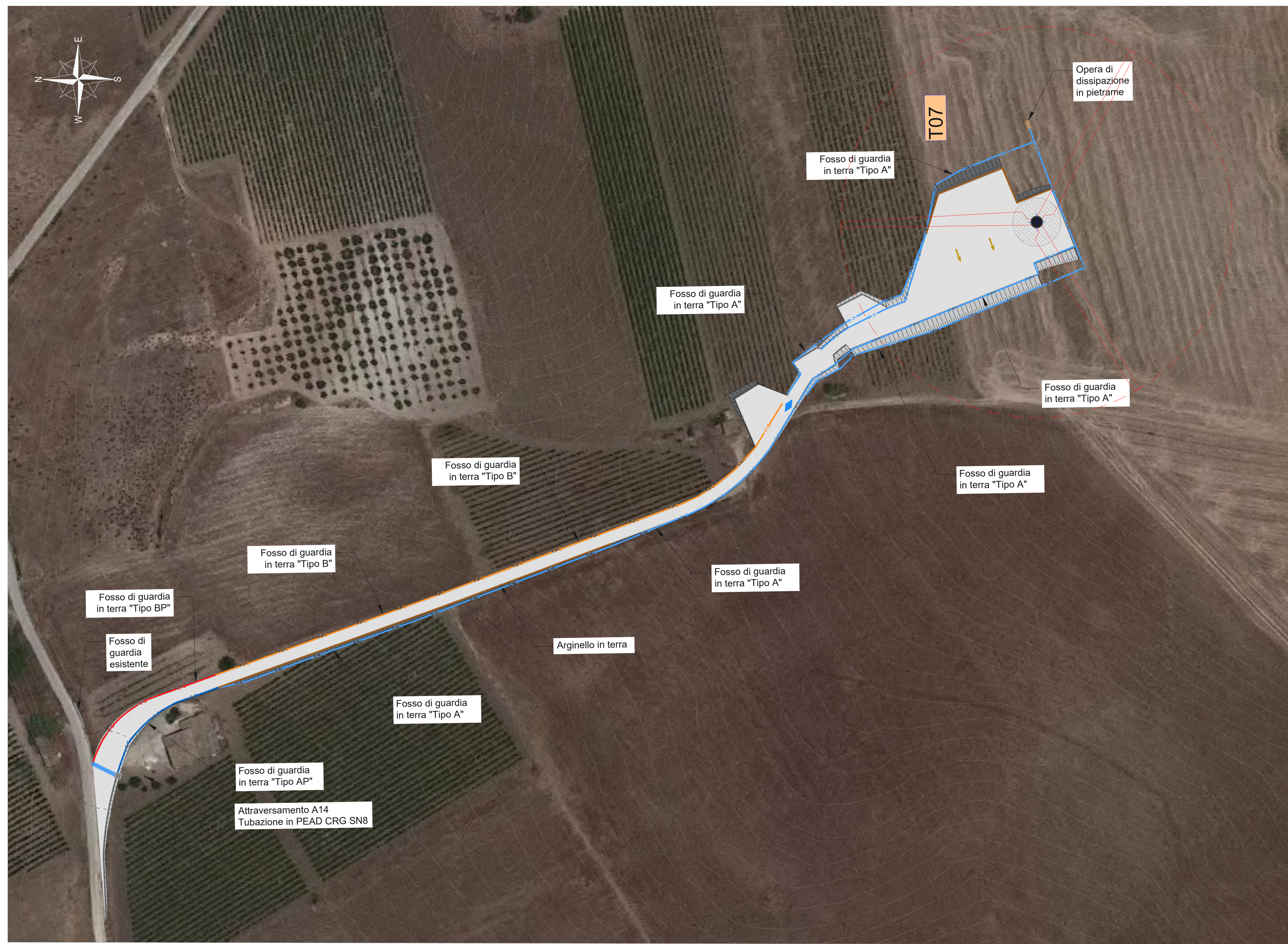
Layout opere idrauliche Asse T07 - Scala 1:1.000
