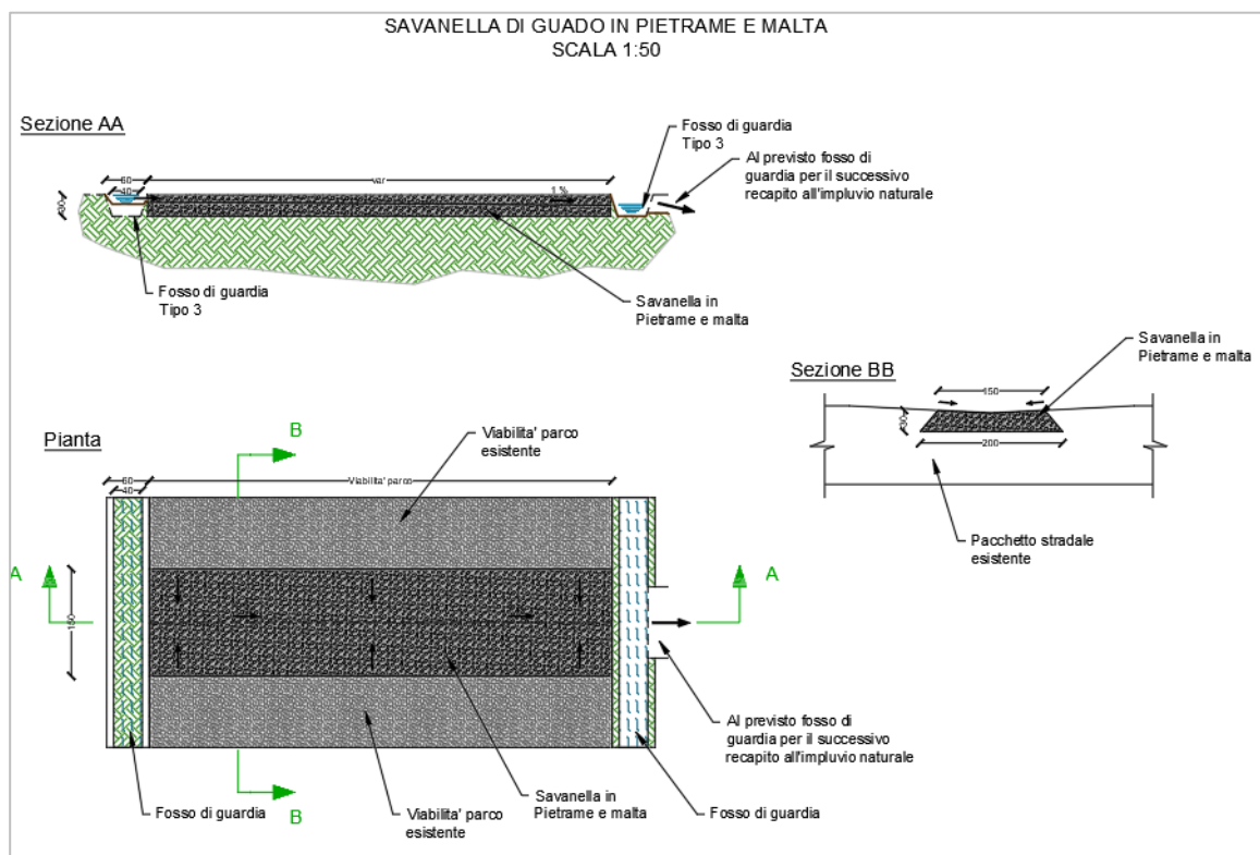
Figura 15- Sezioni longitudinali, trasversali e pianta della savanella di guado.
