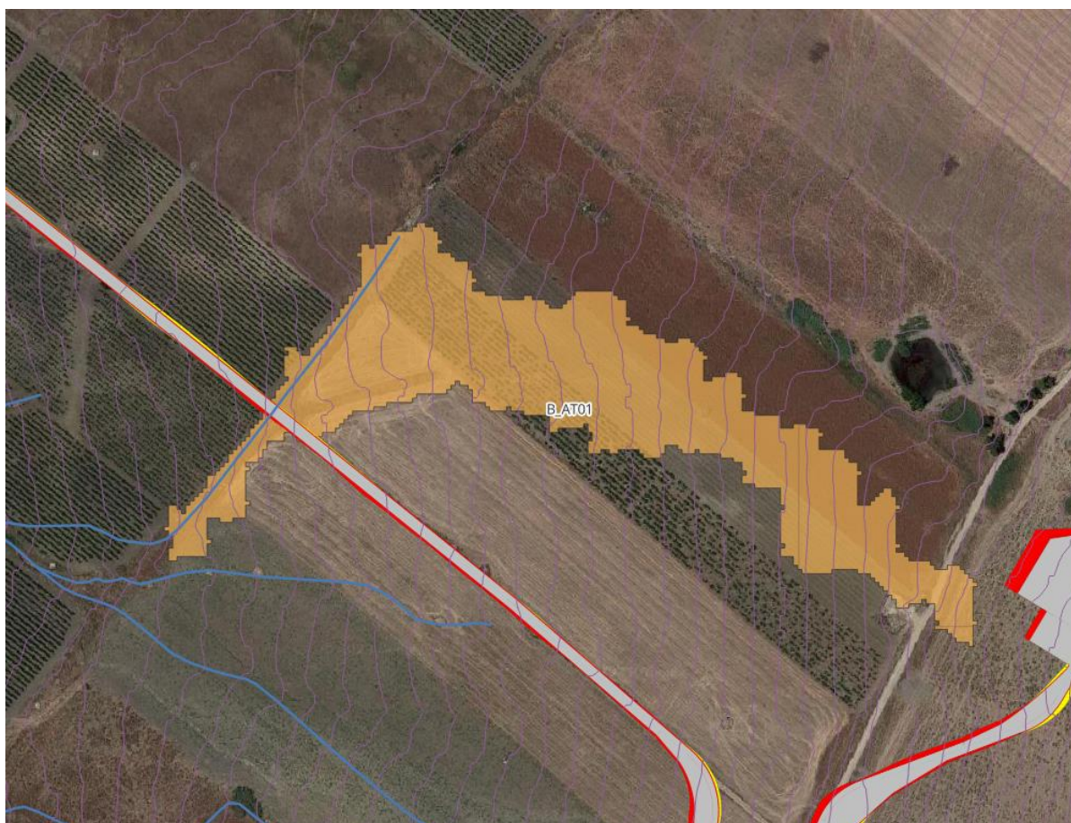
Figura 20- Individuazione bacino idrografico sotteso alla sezione di attraversamento – BAT01.
