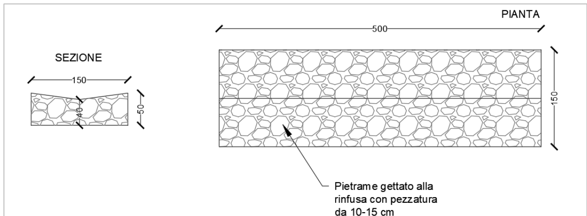
Figura 11- Opera di dissipazione in pietrame.
