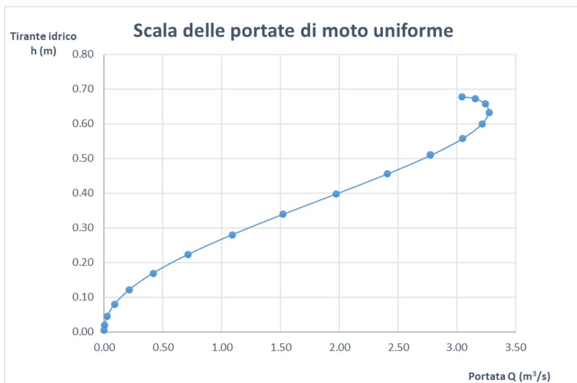
Figura 22- Scala delle portate di moto uniforme per la sezione PEAD CRG SN8 a sezione circolare.
