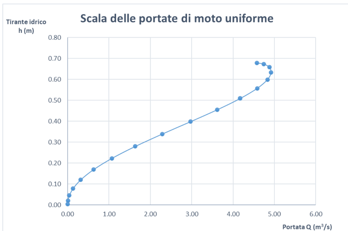
Figura 23- Scala delle portate di moto uniforme per la sezione PEAD CRG SN8 a sezione circolare.
