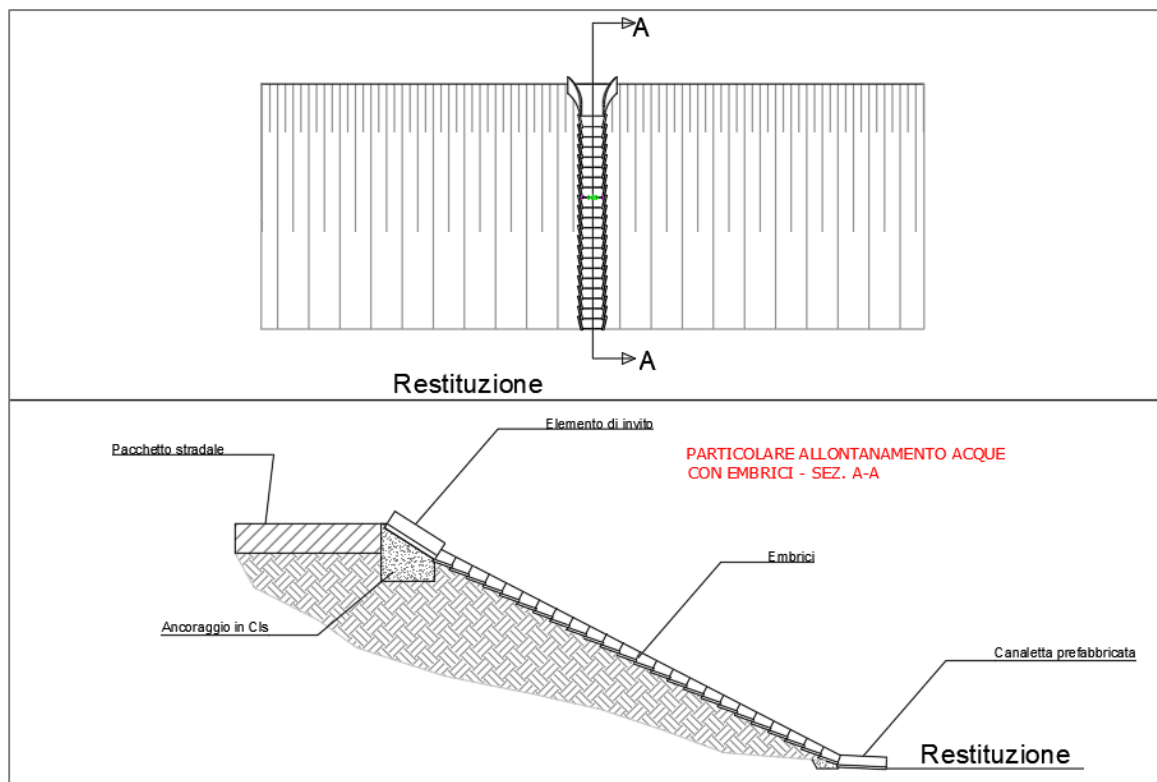
Figura 14- Sezione longitudinale e pianta degli embrici.
