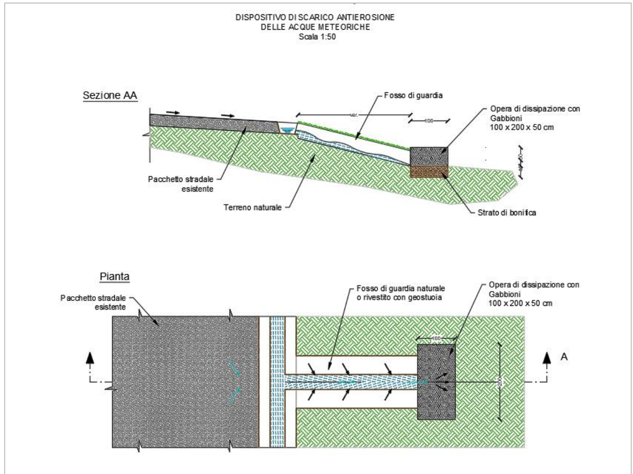
Figura 12- Opera di dissipazione realizzate mediante gabbioni e materassi reno.
