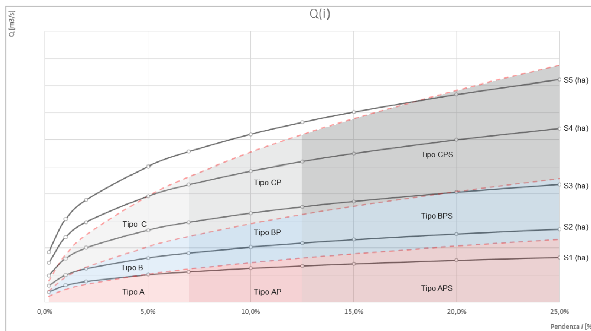
Figura 16- Tipologia di grafico Q(i) con individuazione delle zone omogenee per il pre-dimensionamento dei fossi di guardia.
