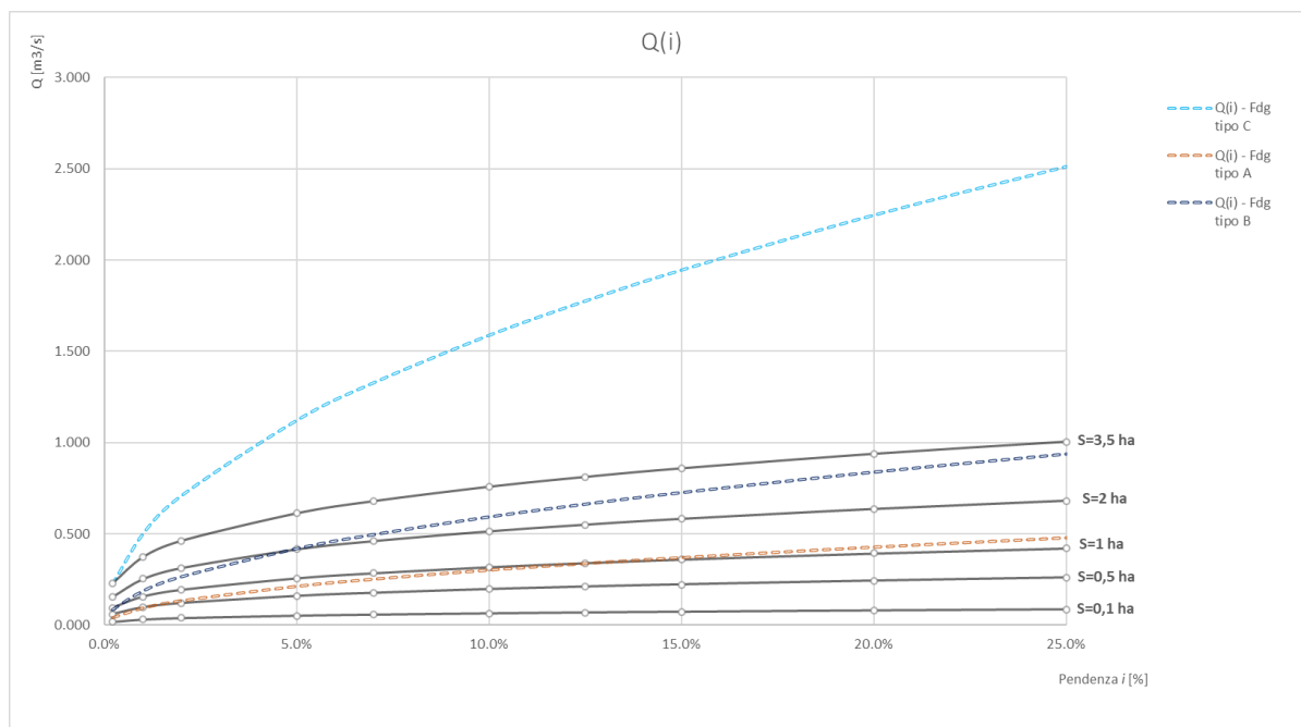
Figura 17- Definizione del grafico Q(i) per il caso in studio, con riferimento ad un tempo di ritorno T pari a 30 anni.
