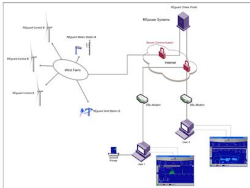
Figura 1 Schema di interconnessione con Sistema SCADA .
