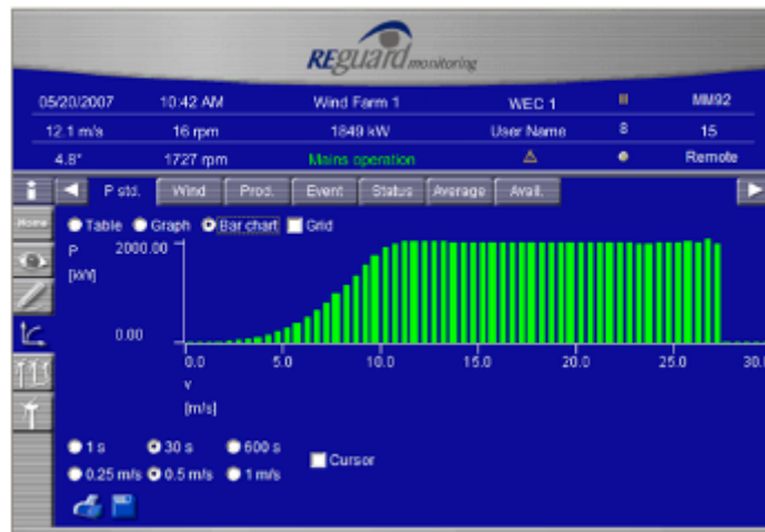
Figura 3 SCADA – Visualizzazione Curva di Potenza – Velocità.
