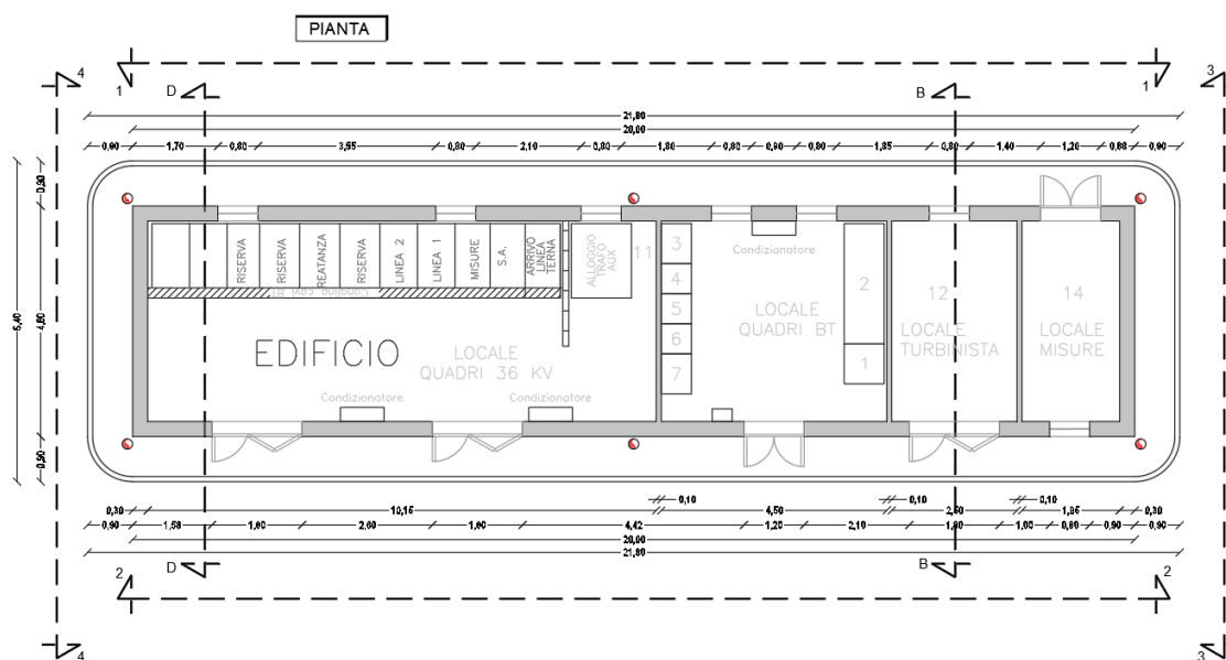
Layout edificio consegna
