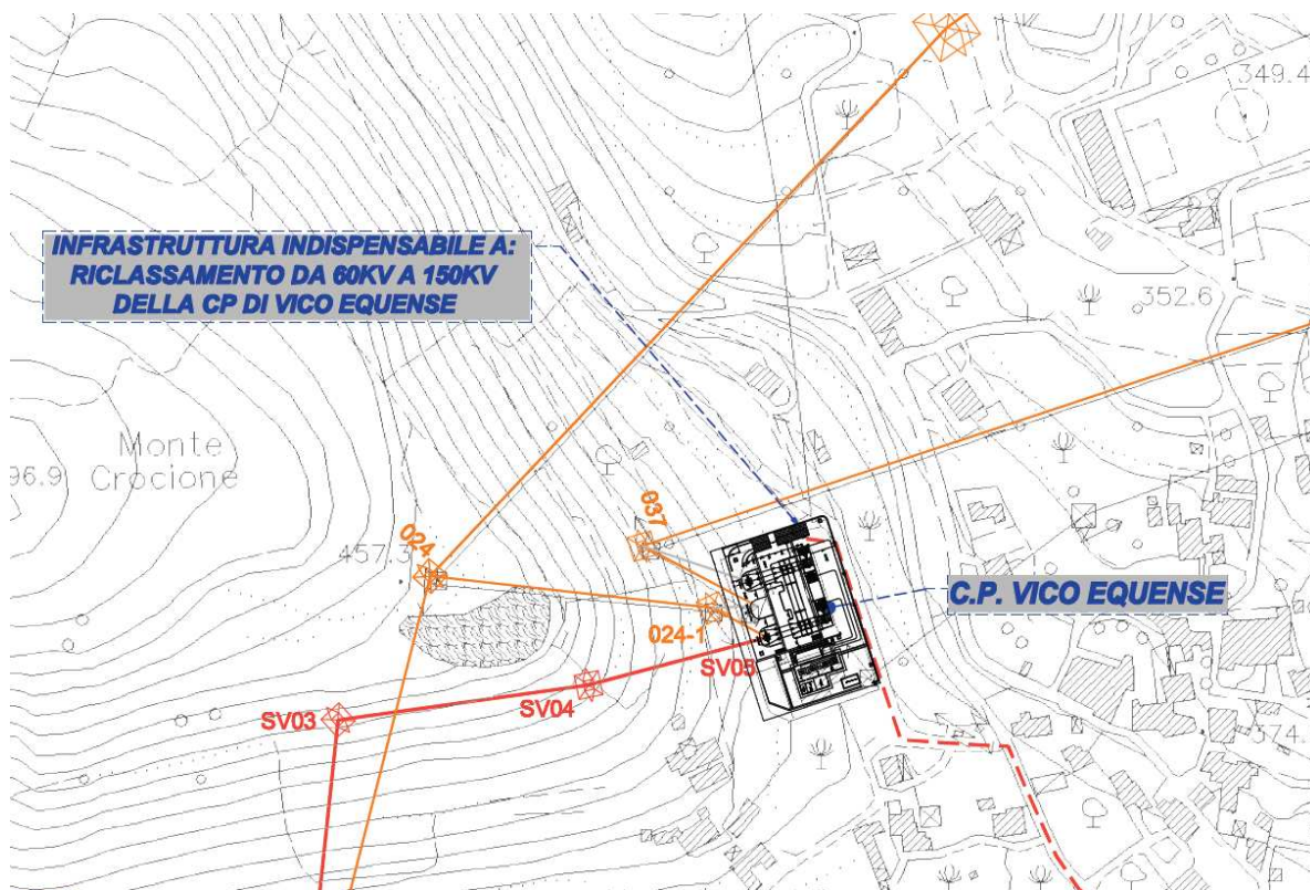
Figura 1 – Corografia 1:2000 Doc. A-ENEL-002R
