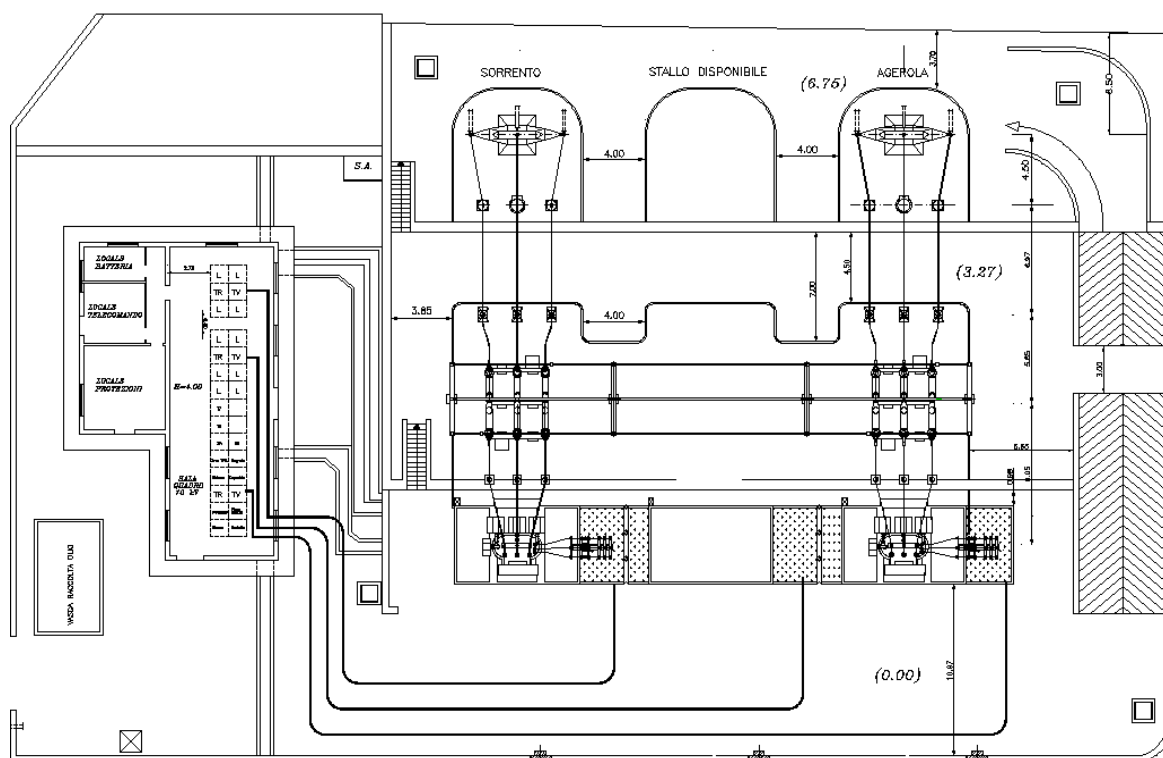
Figura 2 – Planimetria generale Doc. A-ENEL-004D
