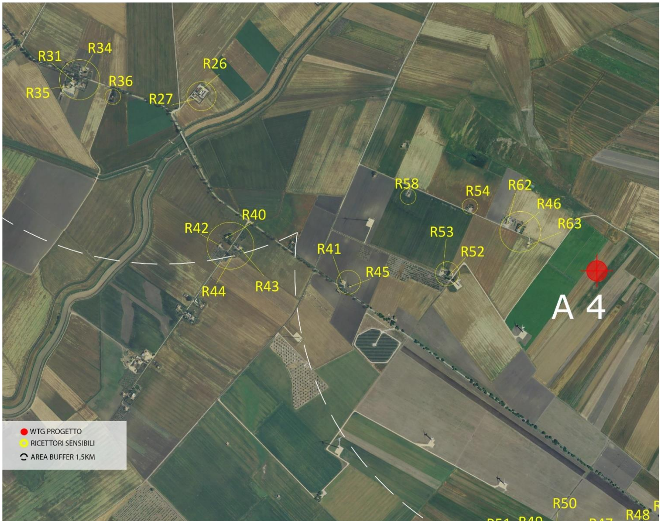
figura 15: Vista della porzione del parco di Progetto con evidenza della turbina A4 e dei ricettori sensibili, indicati con etichetta "R", rientranti nel buffer di 1,5 km dalle torri.
