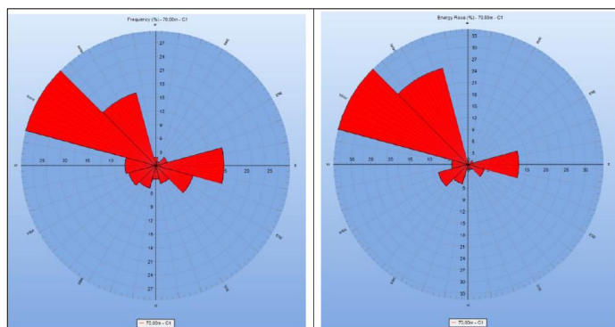
figura 12: Rosa dei venti a 70 m di altezza, per frequenza (sinistra) ed energia (destra).
