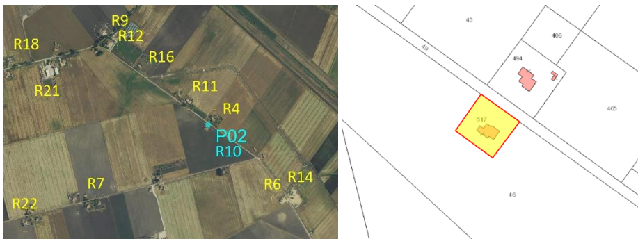
figura 23: Inquadramento geografico della postazione fonometrica PF 02 ed inquadramento catastale del ricettore R10.
