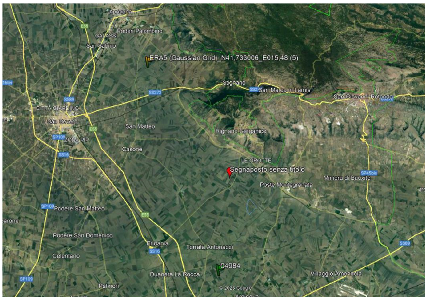
figura 11: Posizione delle due stazioni anemometriche virtuali rispetto al sito di progetto (EMD-WFR rappresenta la stazione virtuale MESO DATA). La puntina rossa indica la posizione prevista del parco eolico in progetto.
