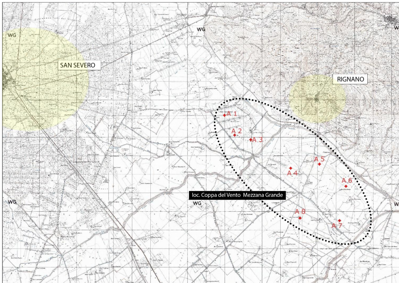
figura 10: inquadramento impianto di Progetto su IGM 1.25000
