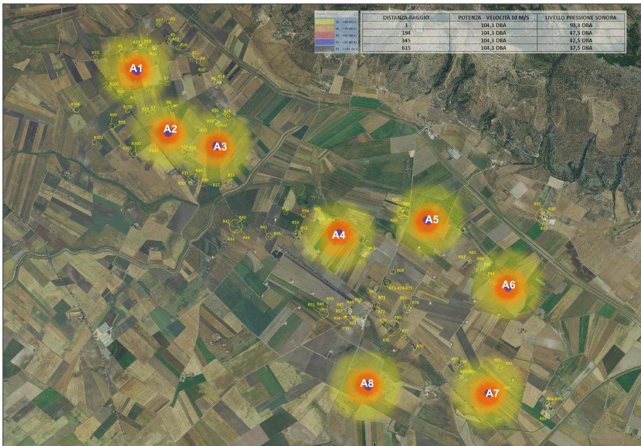
figura 39: Mappa curve Isolivello del rumore emesso dagli aerogeneratori di progetto espresso in Leq(A) nelle condizioni di massima emissione elaborata per velocità del vento di 10 m/s in vista estratta da Google Earth
