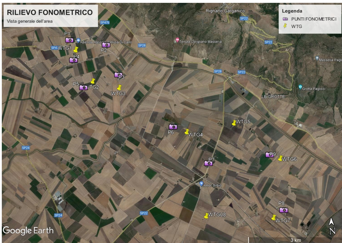
figura 20: Inquadramento geografico dell'area di progetto e delle postazioni fonometriche scelte.
